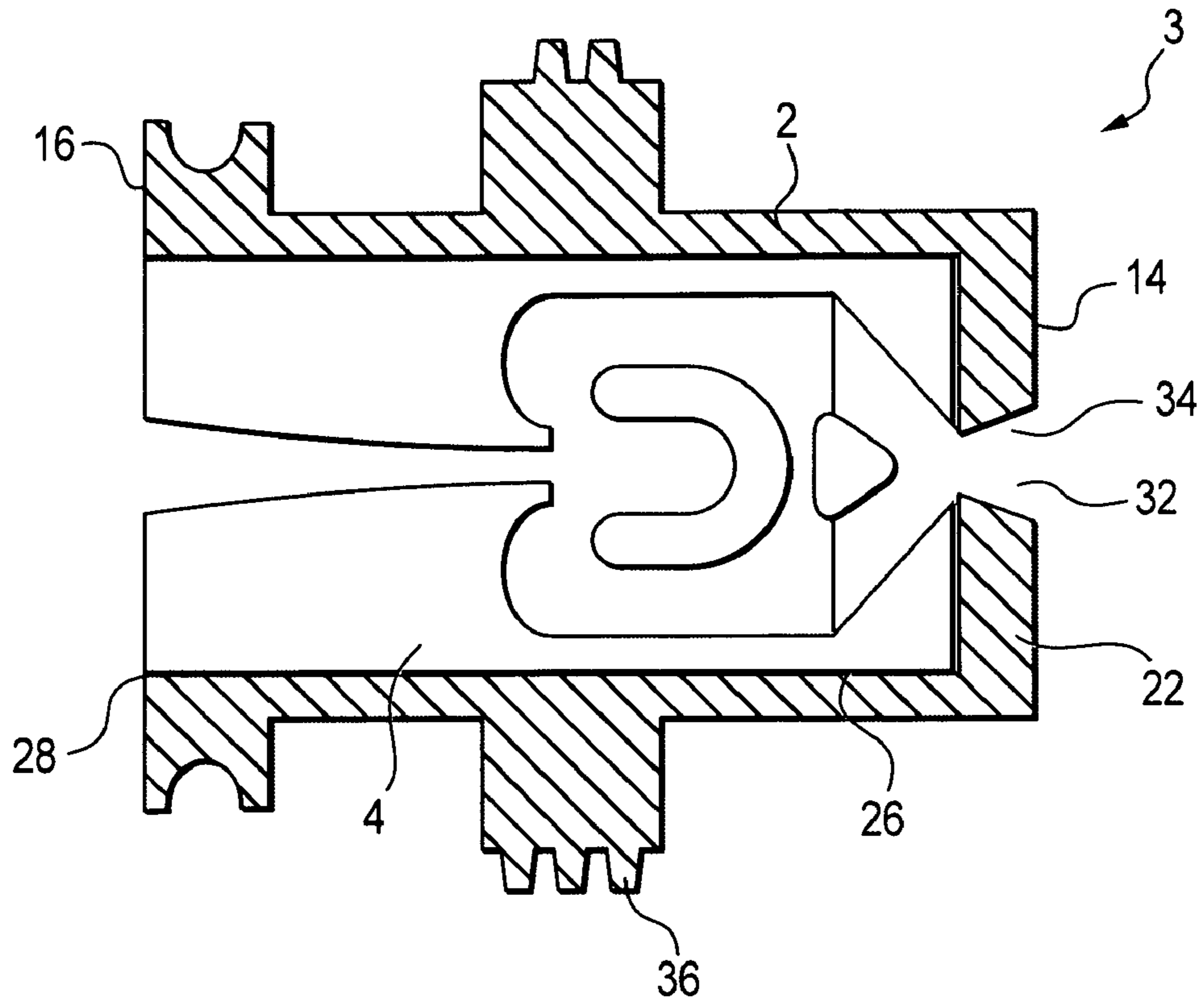
SECTION A-A FIG. 9C
