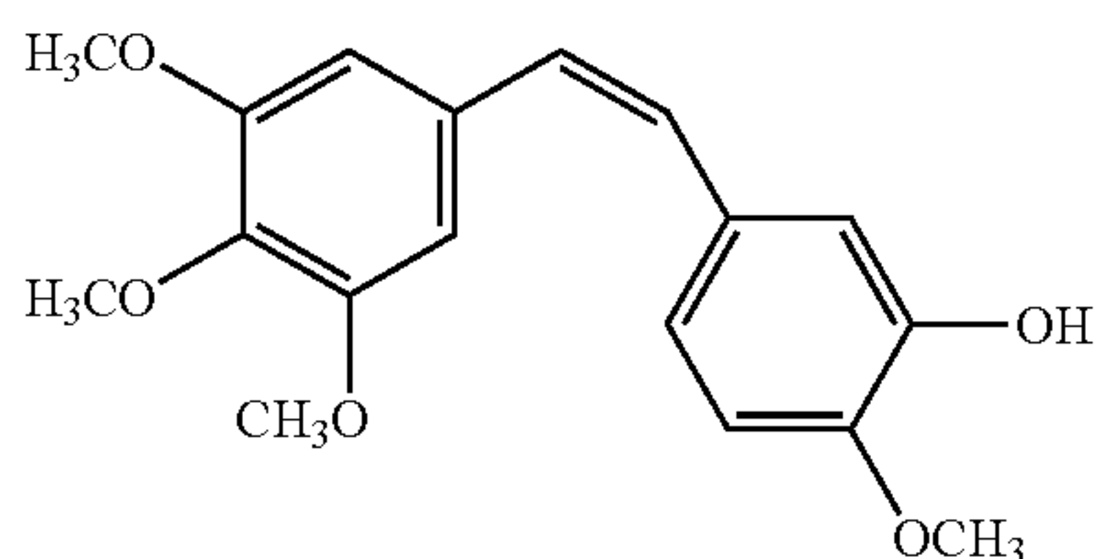
Combretastatin A-4
