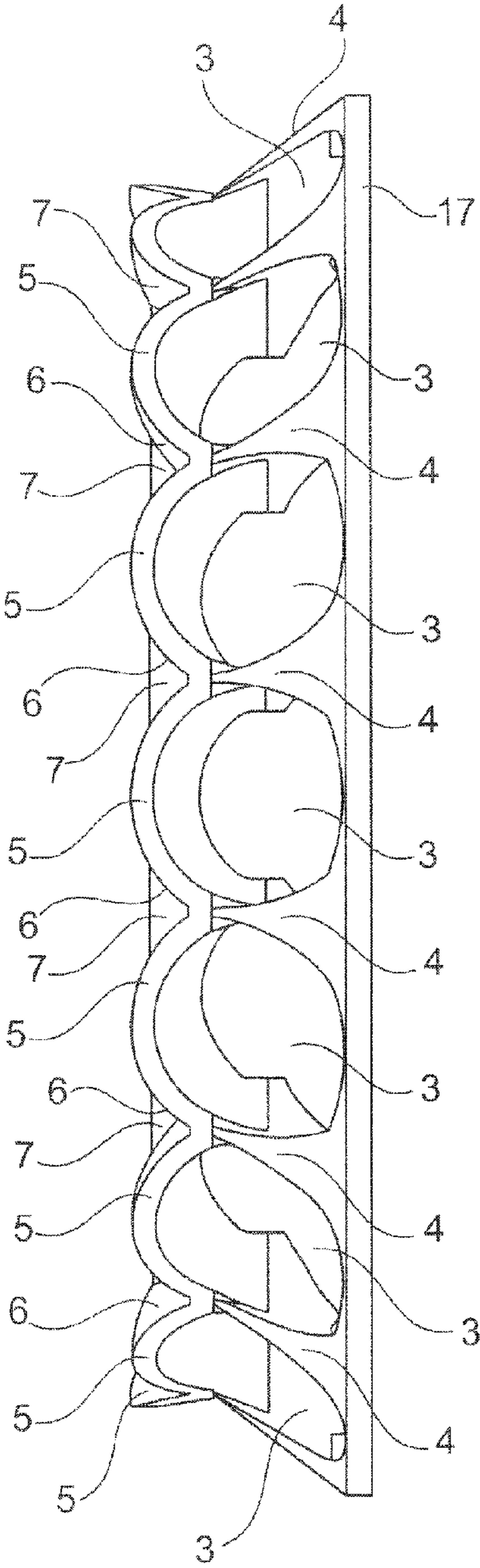
Fig. 3
