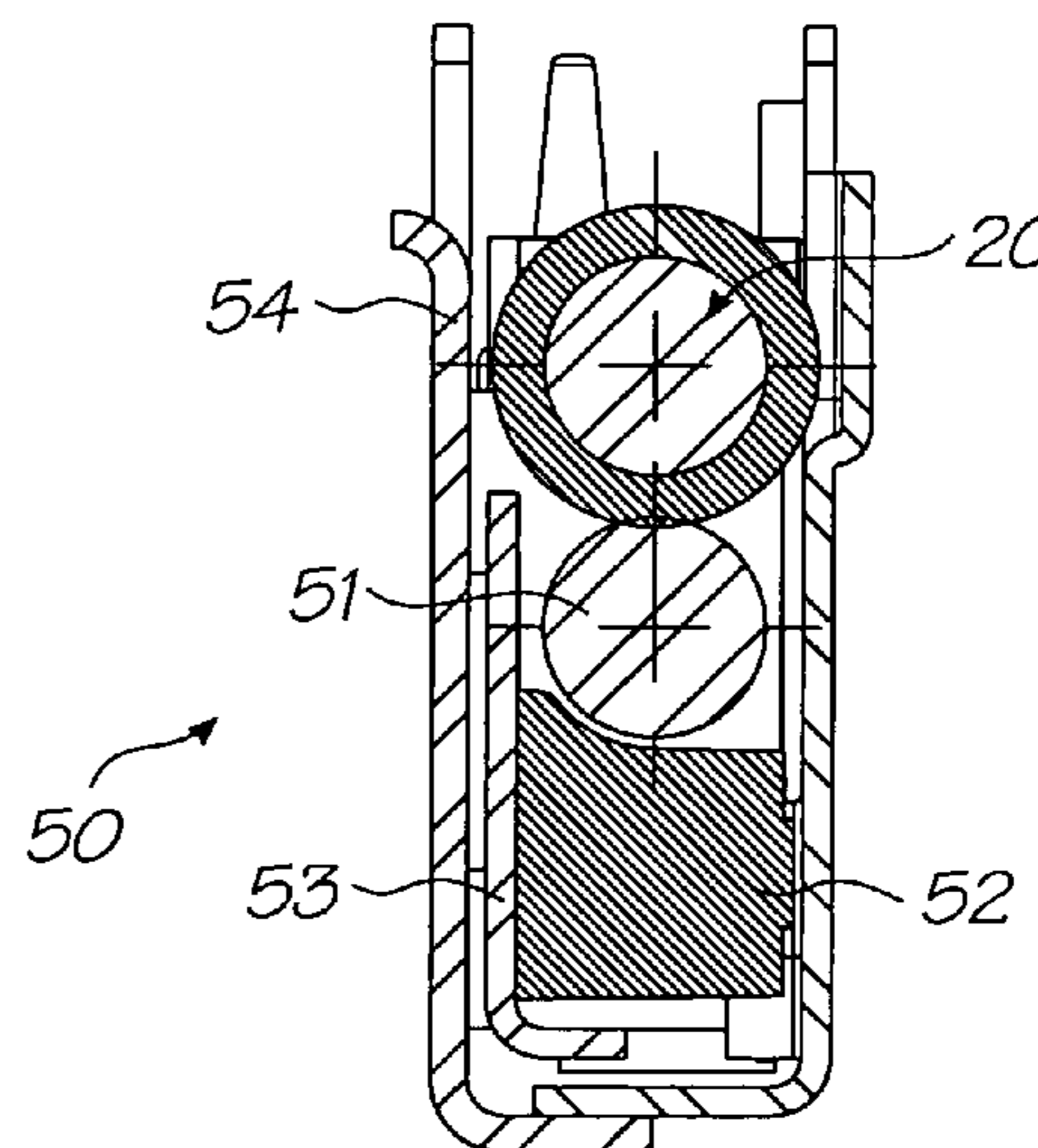
Section A-A
