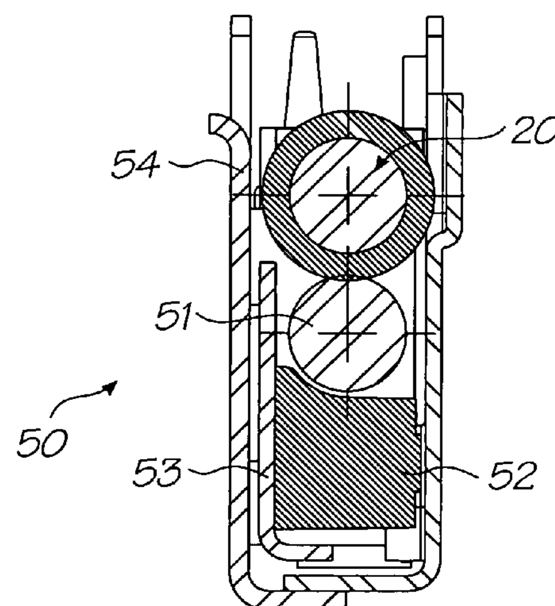
Section A-A
