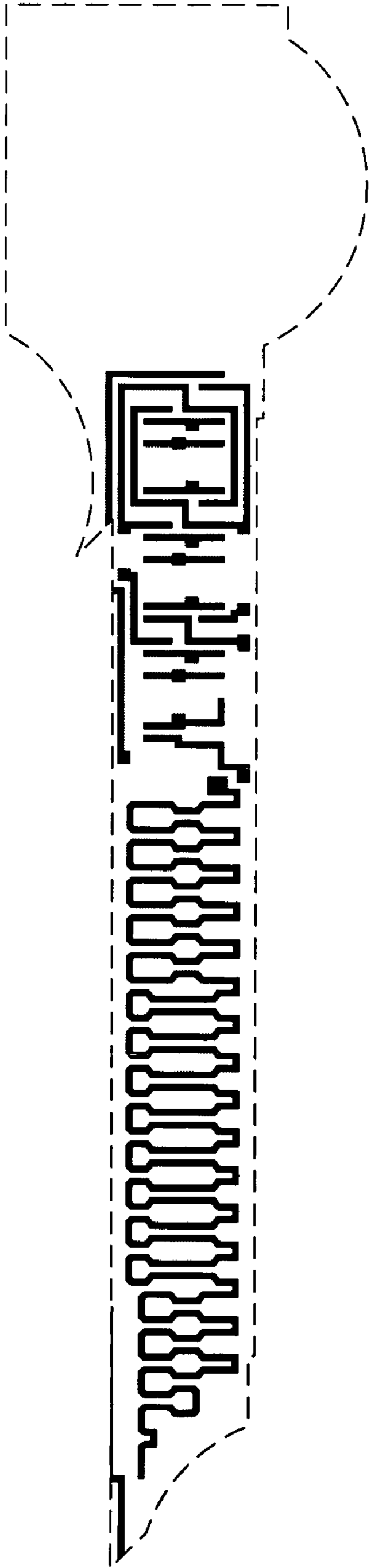
Poly mask
