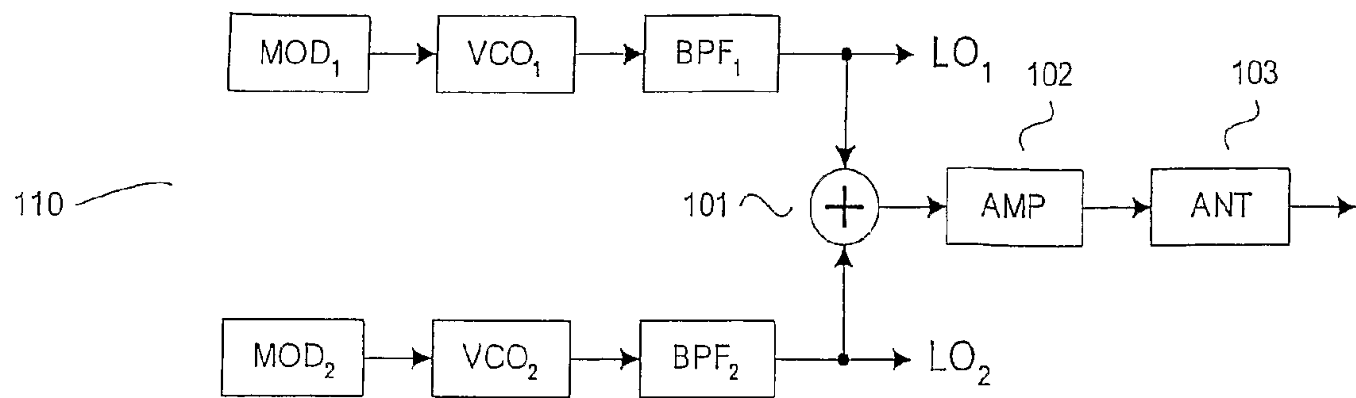
Fig. 1a Transmitter
