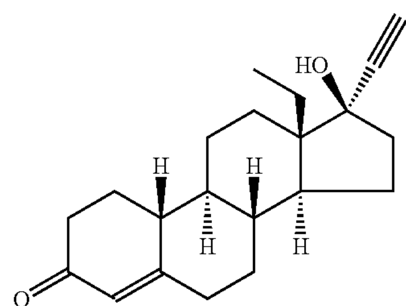
Levonorgestrel
