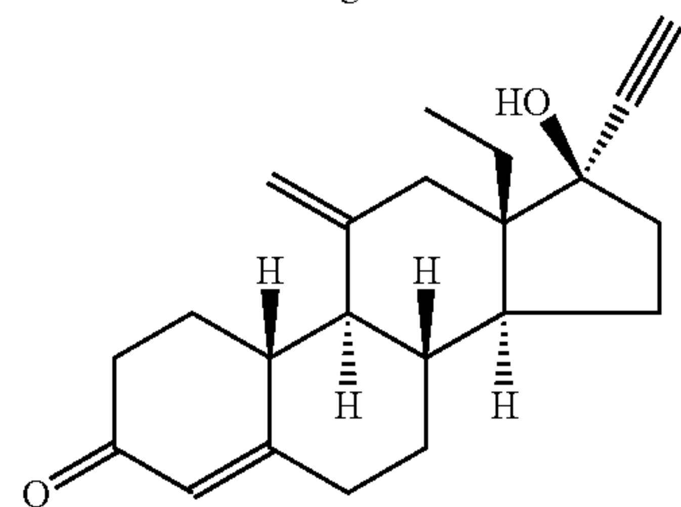
Etonogestrel
