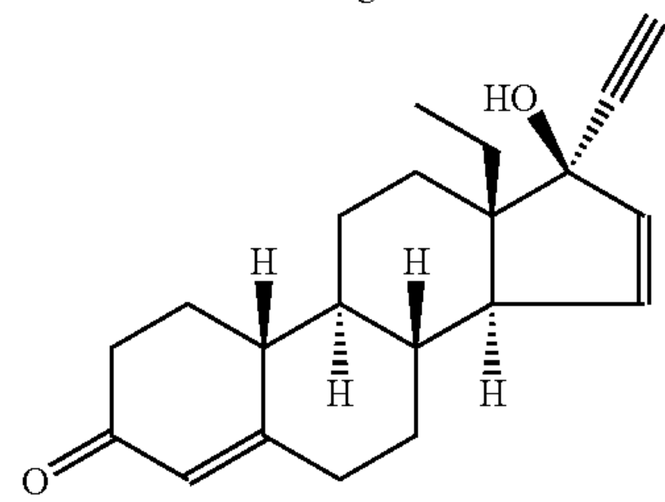
Gestodene
