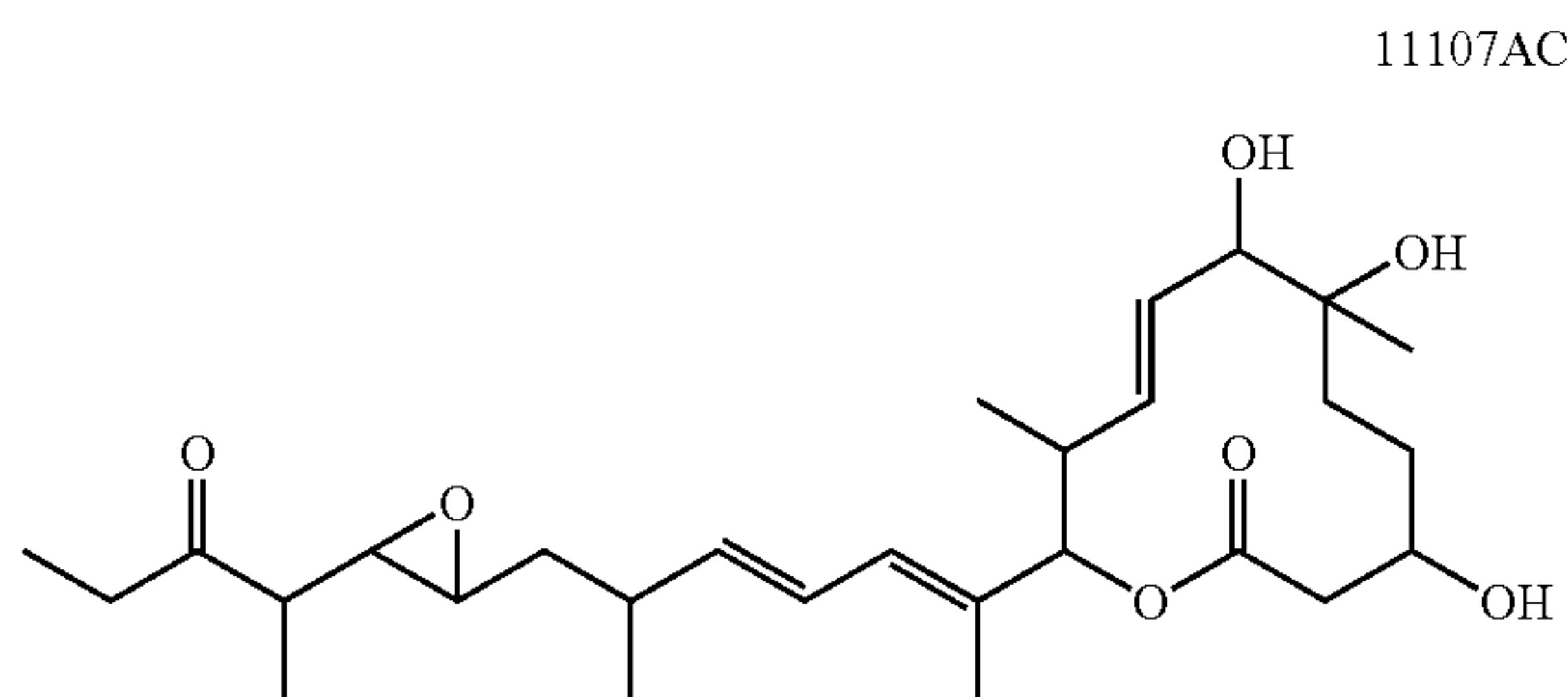
Example A36
