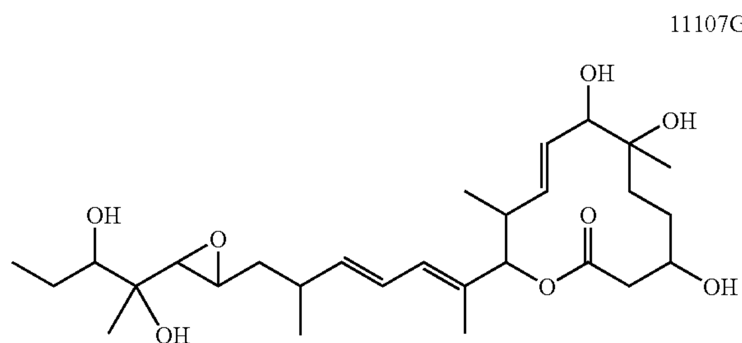
Example A10
