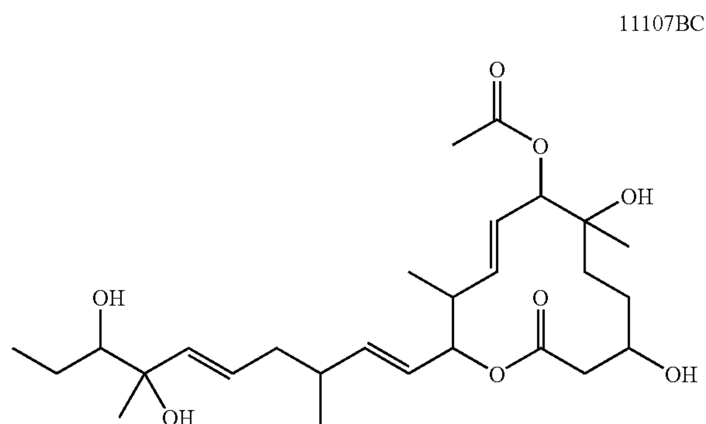
Example A56
