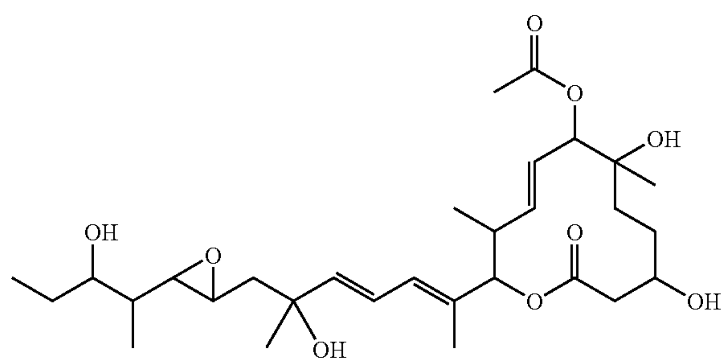
Example A7
