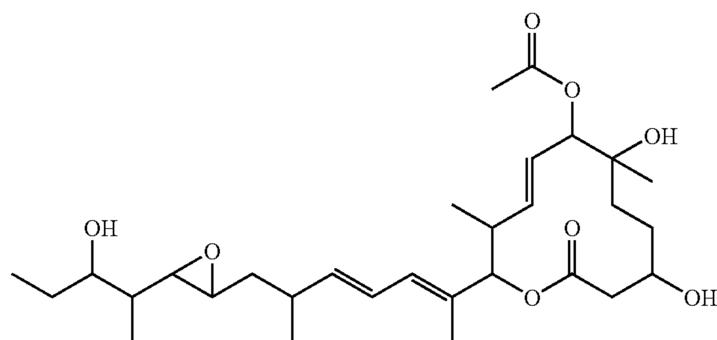
Example A5
