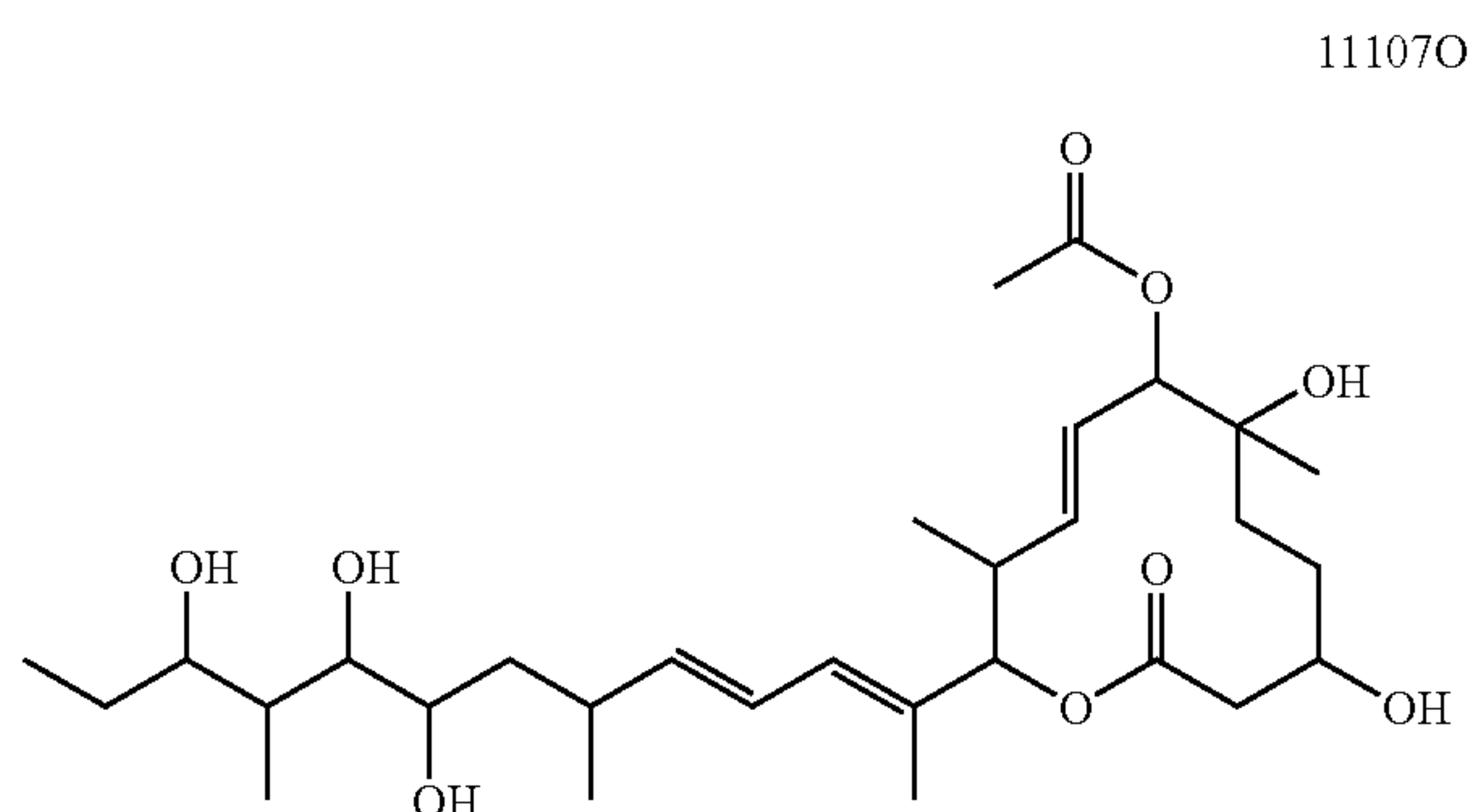
Example A22
