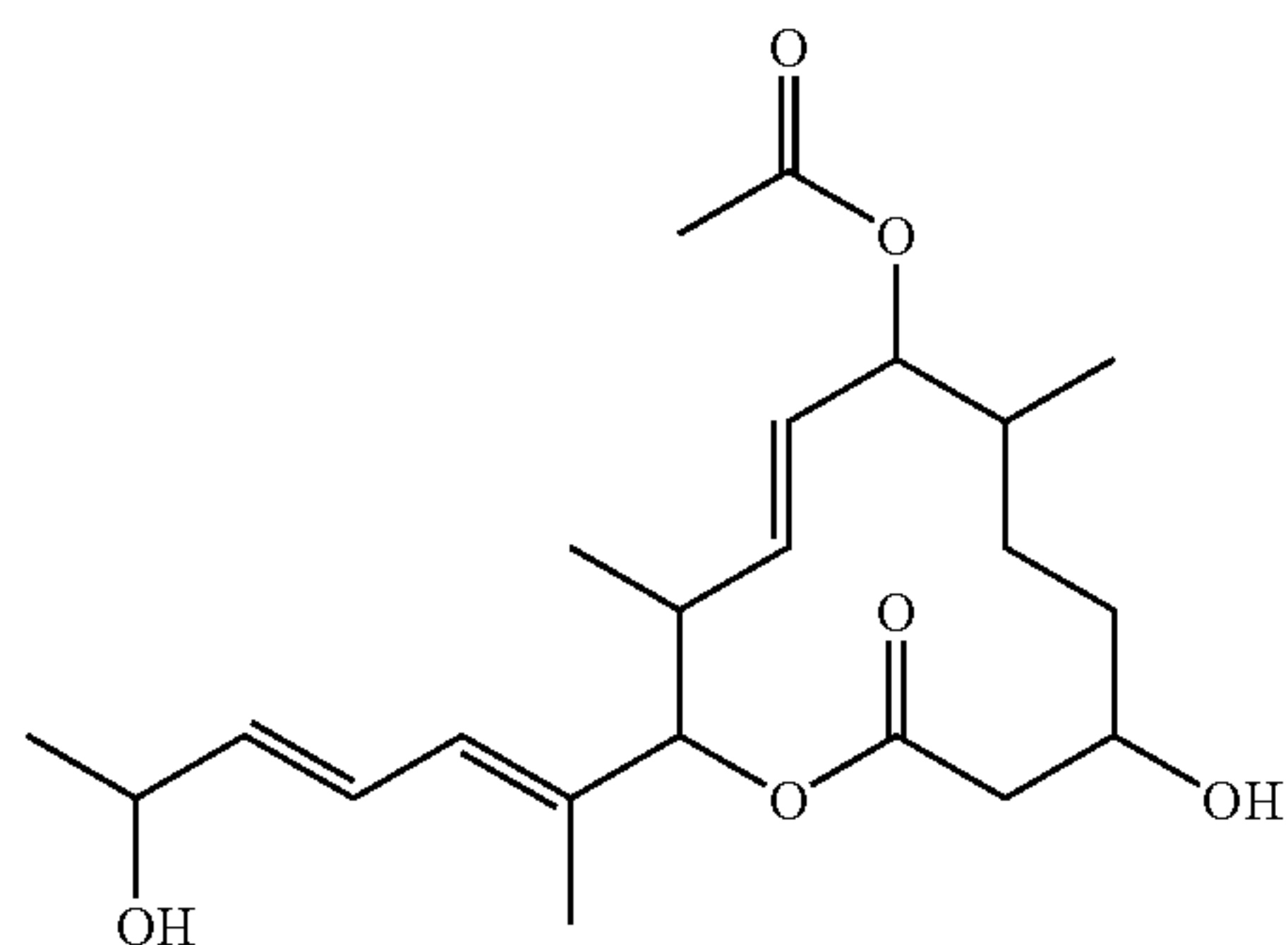
Example A50
