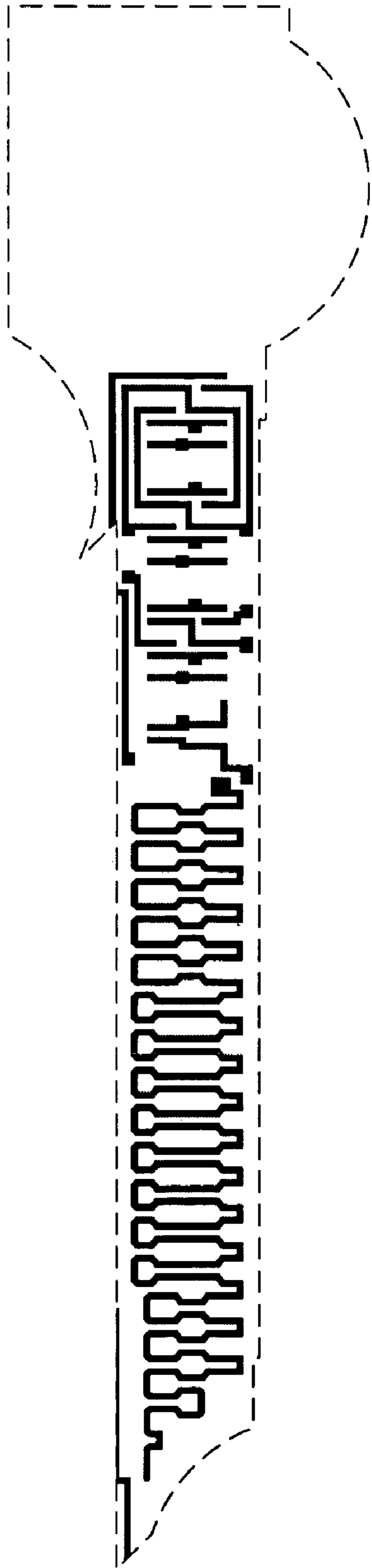
Poly mask
