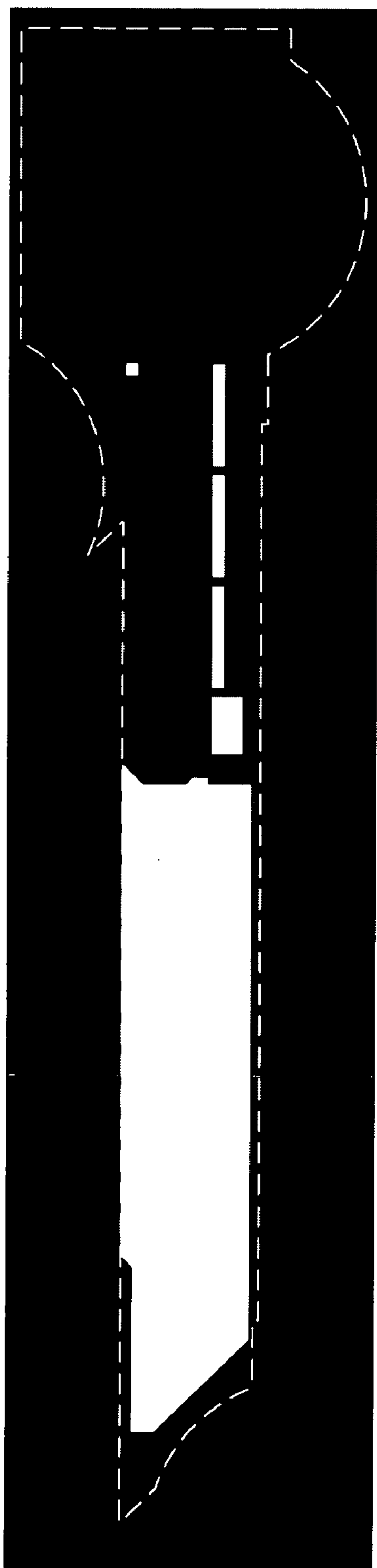
p+ mask
