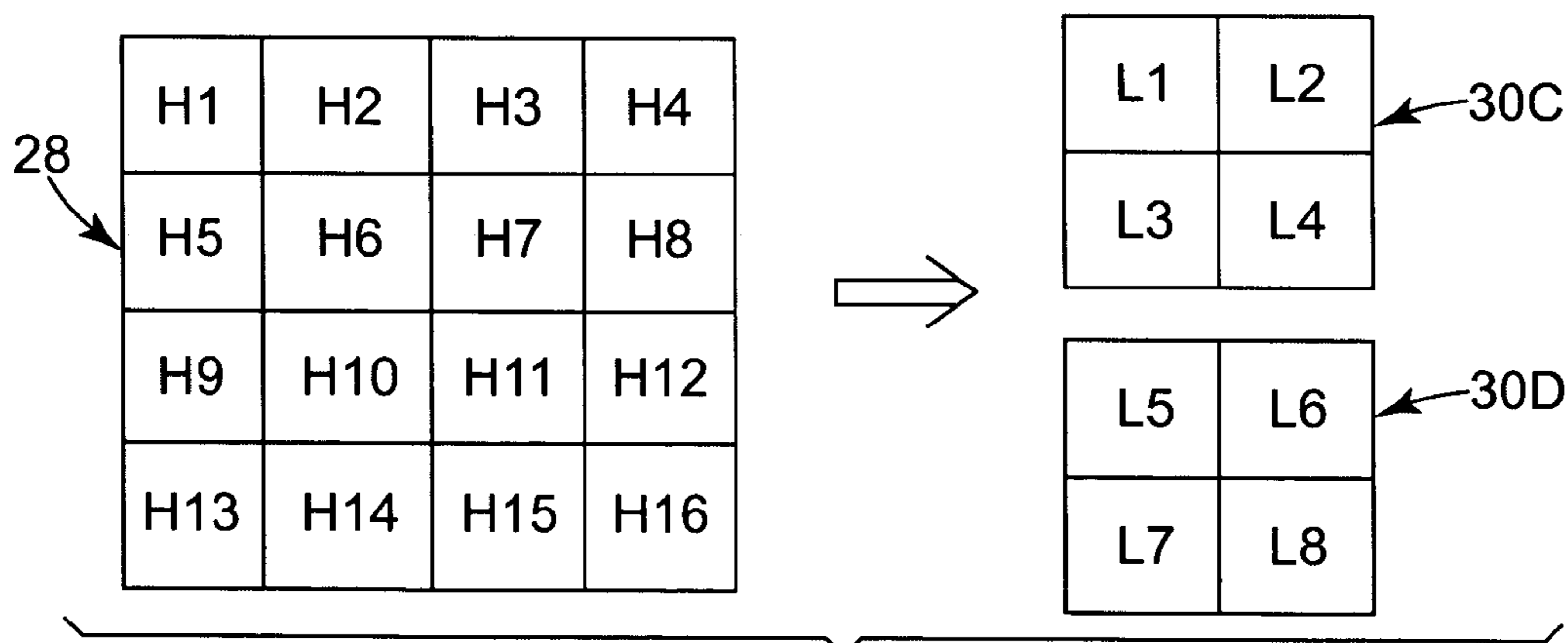
Fig. 6 (BILINEAR)
