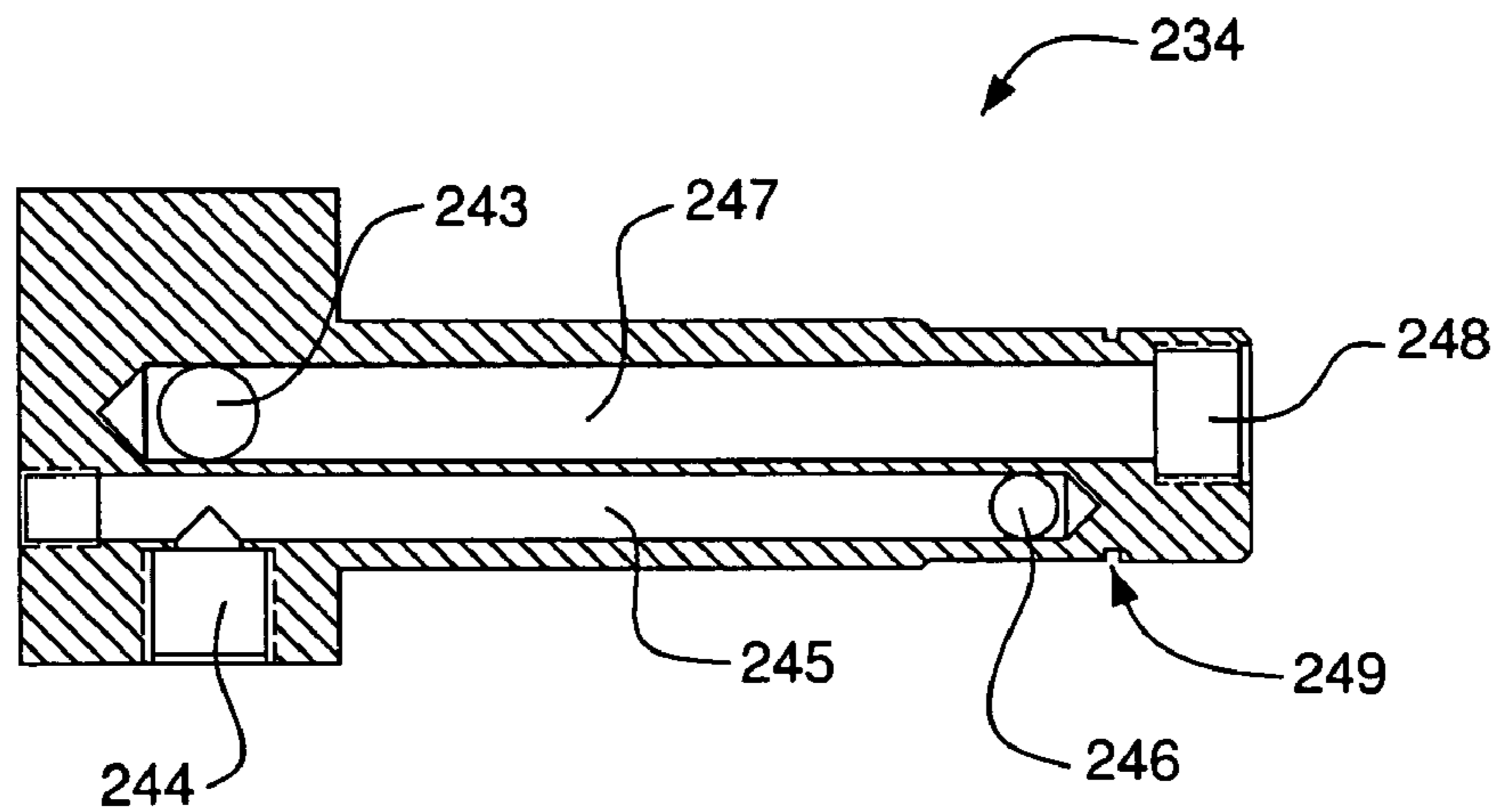
SECTION A-A
