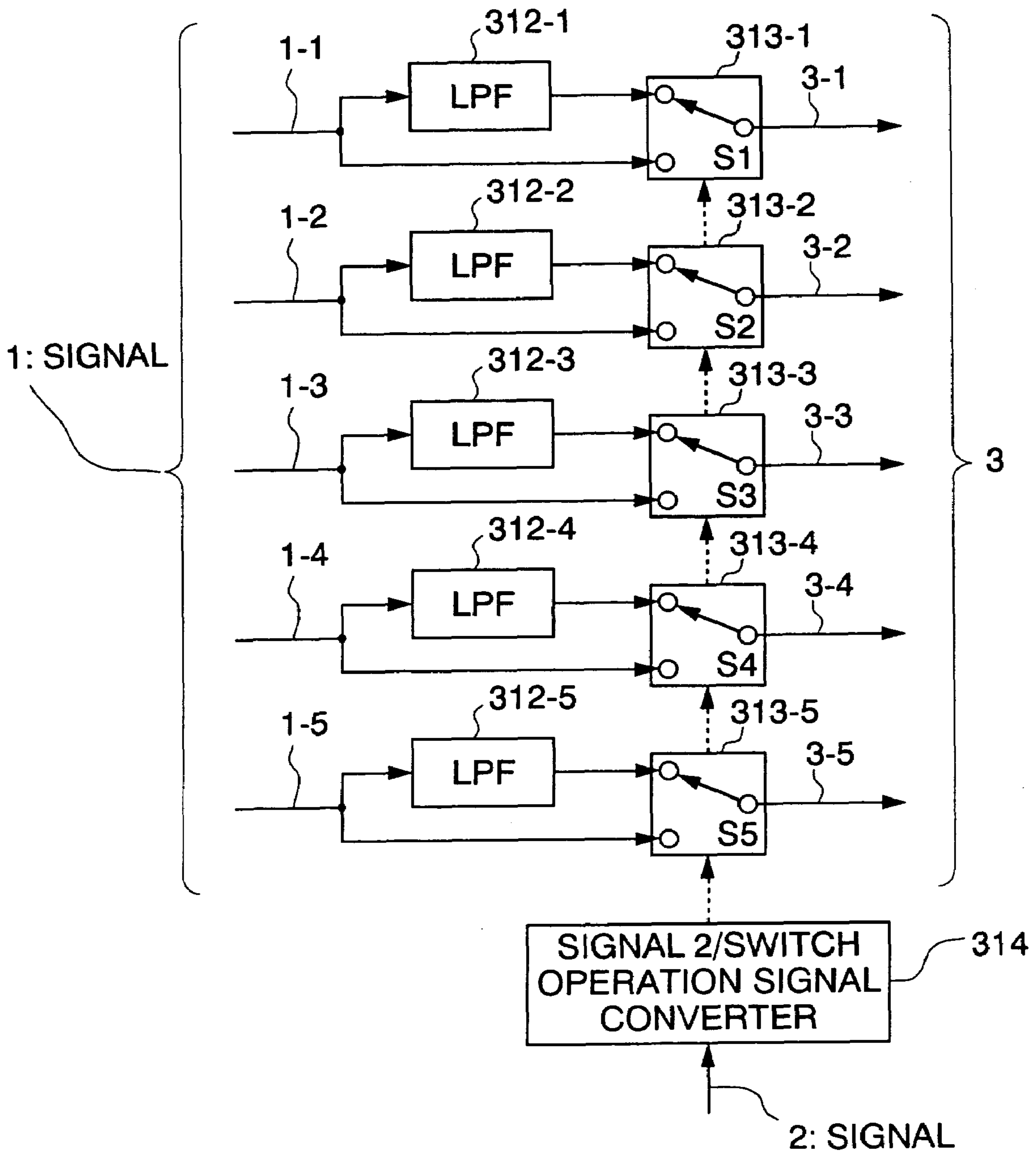
FIG. 21
