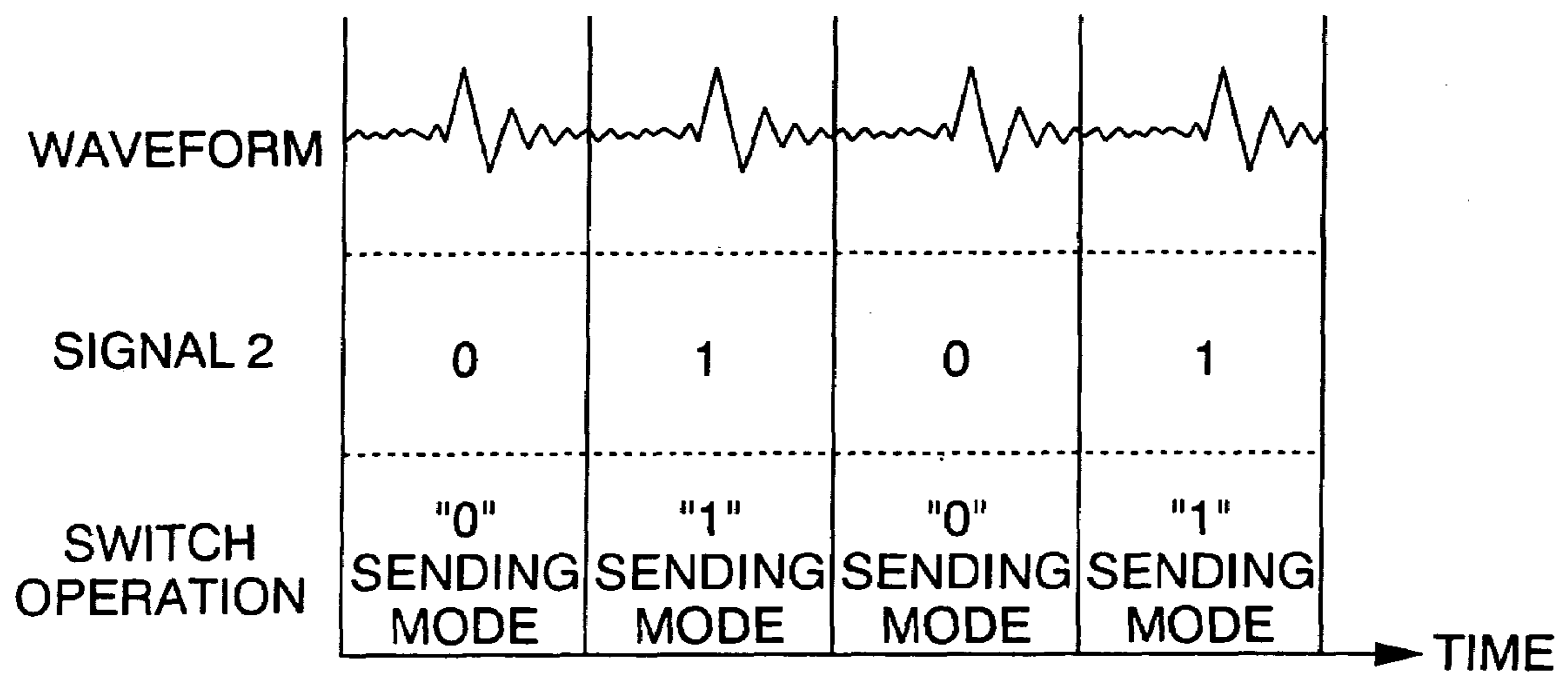
FIG. 22B
