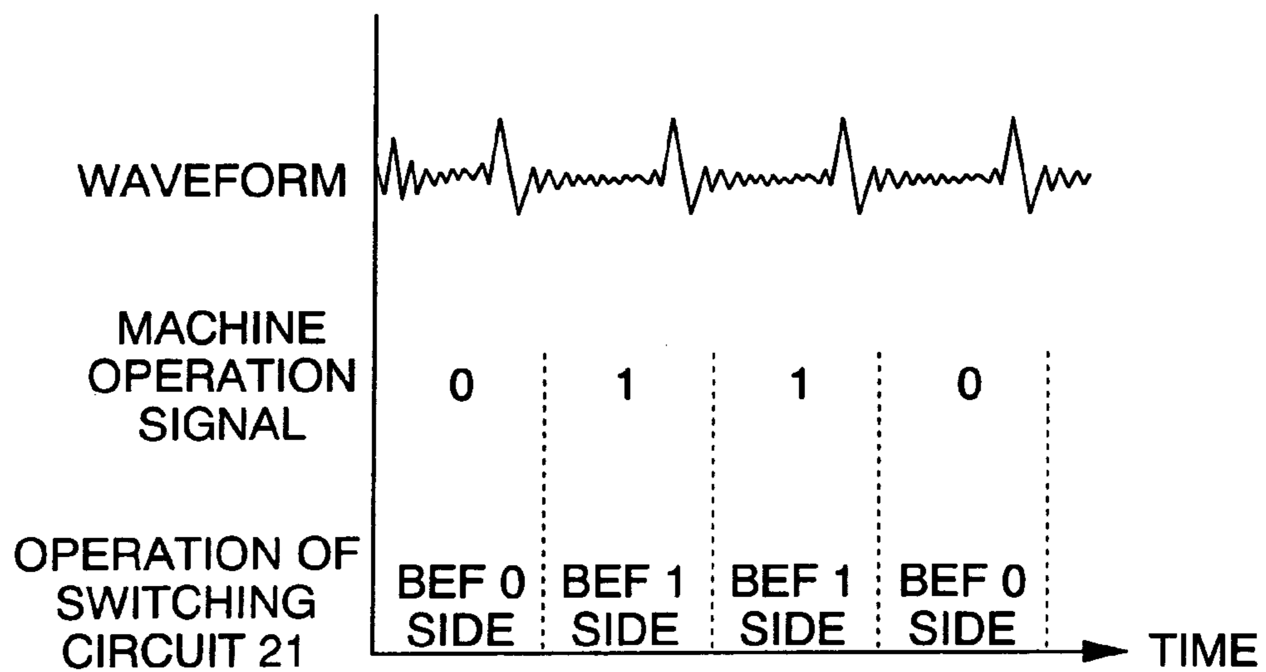
FIG. 4B
