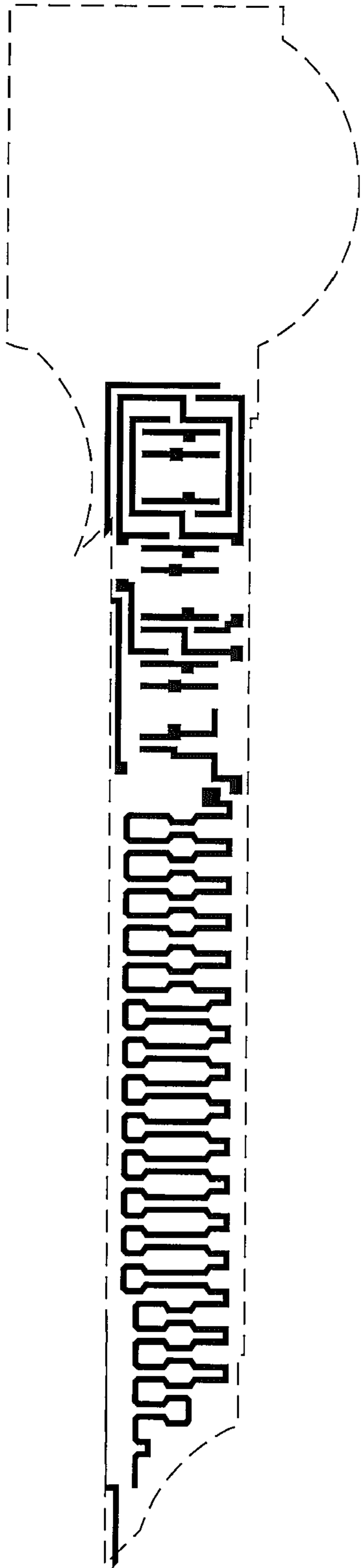
Poly mask
