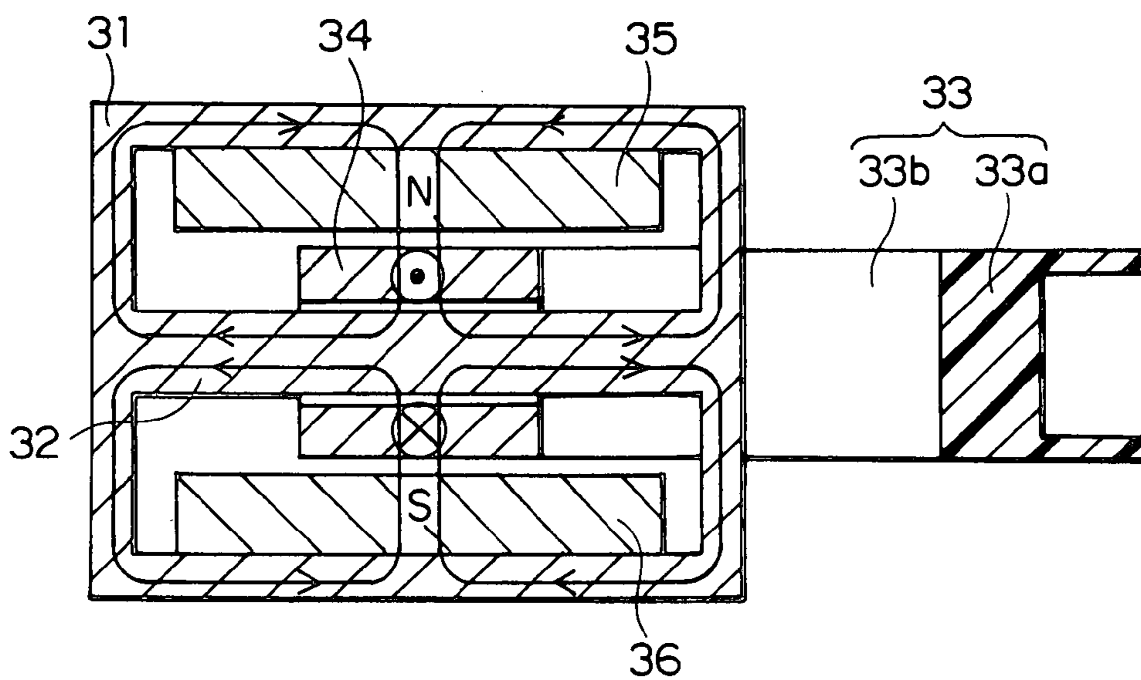
FIG. 18B
