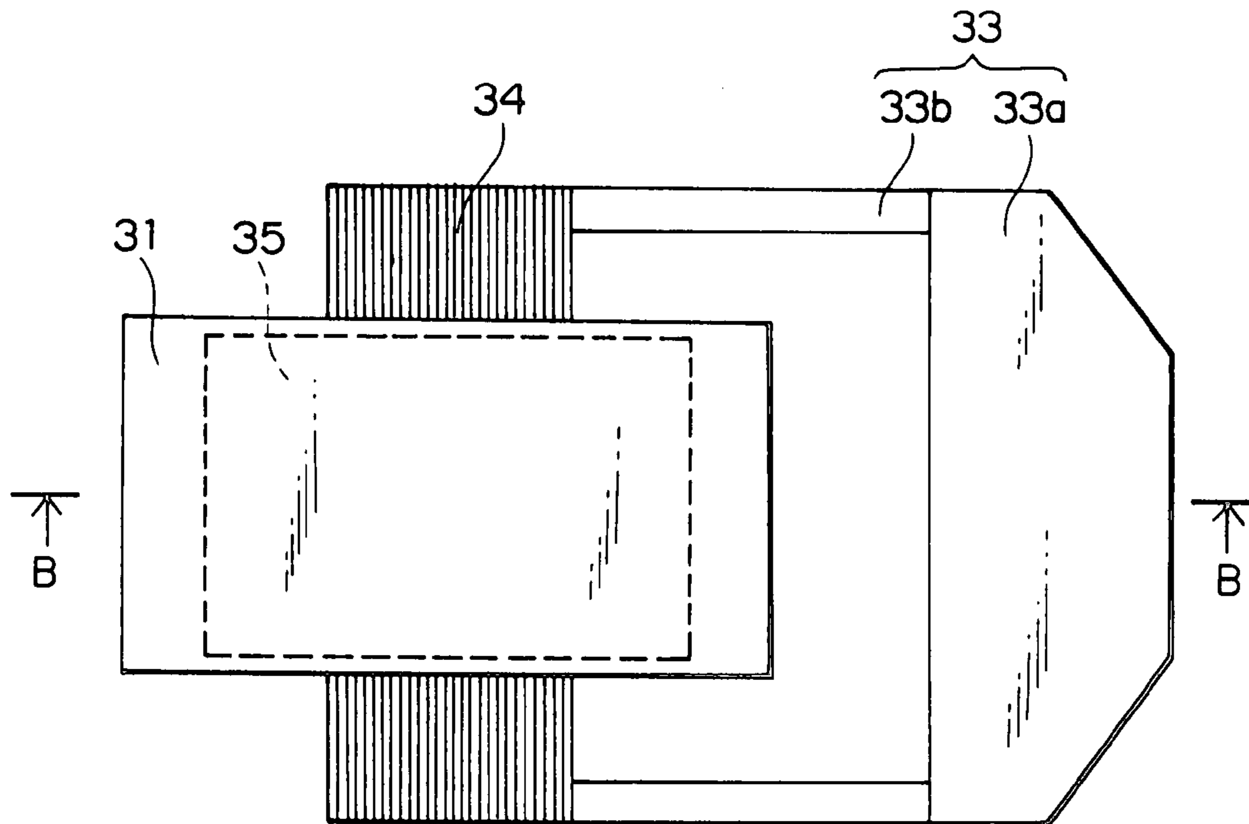
FIG. 18B
