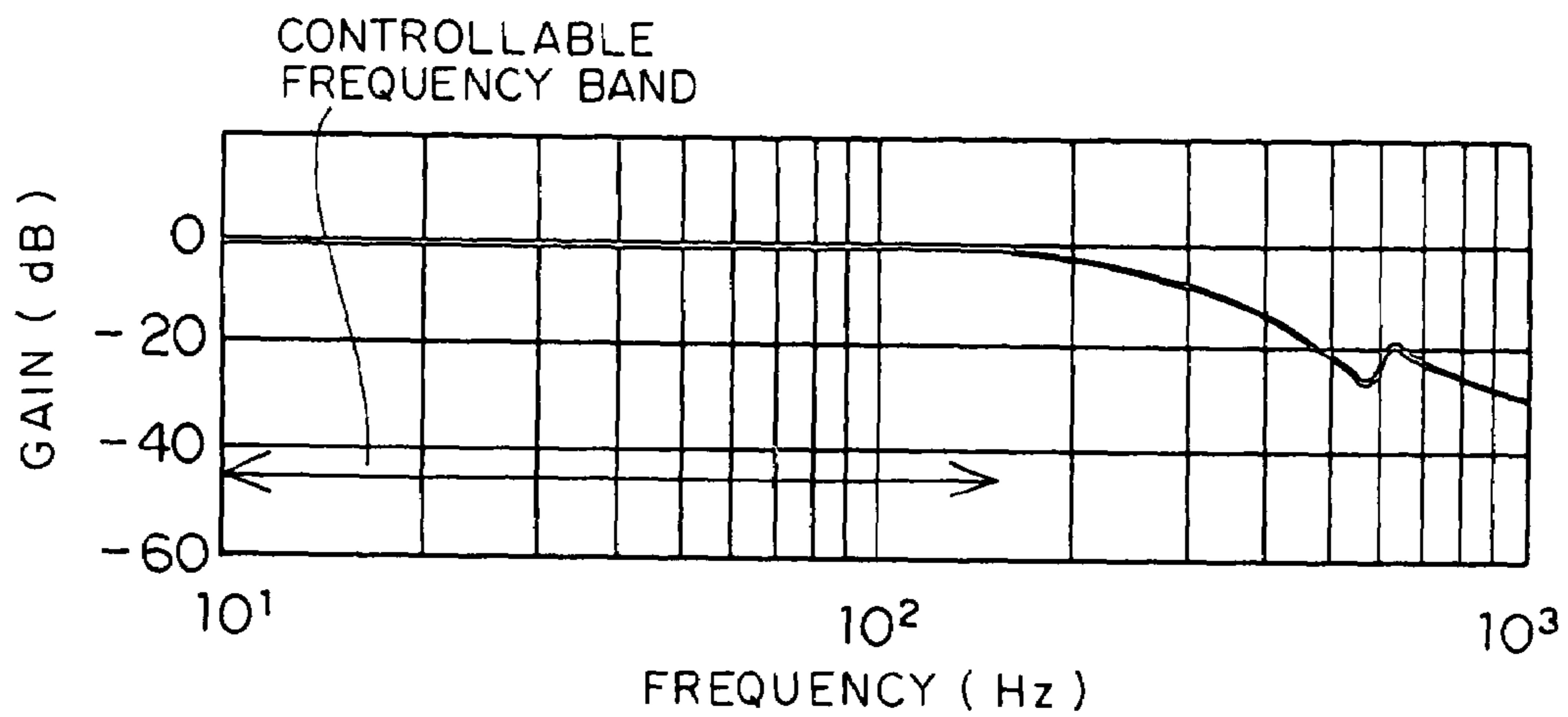
FIG. 16A
