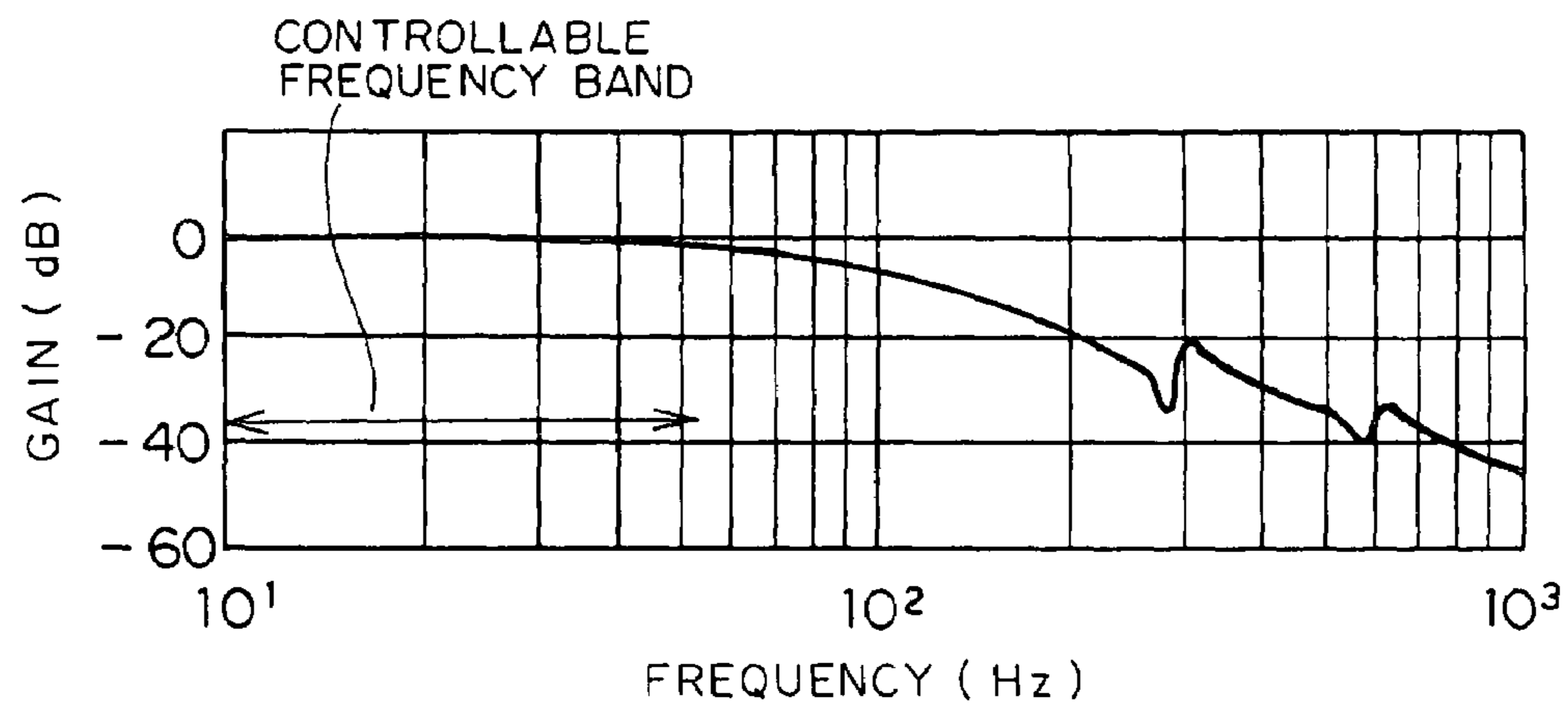
FIG. 15A
