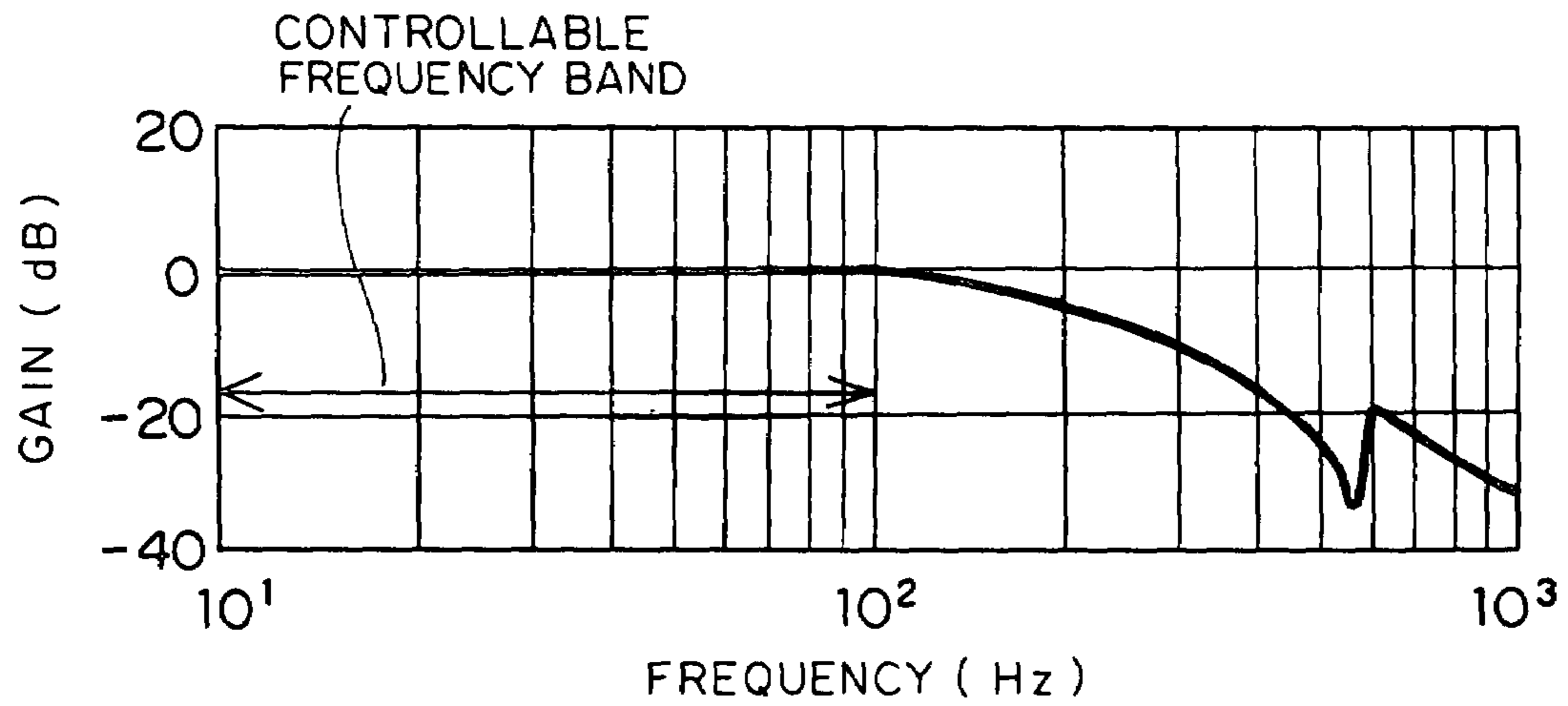
FIG. 12A
