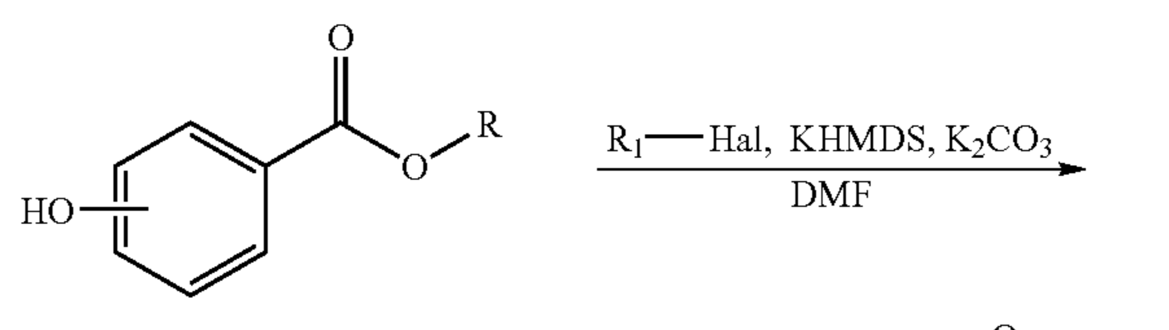
Scheme VI
