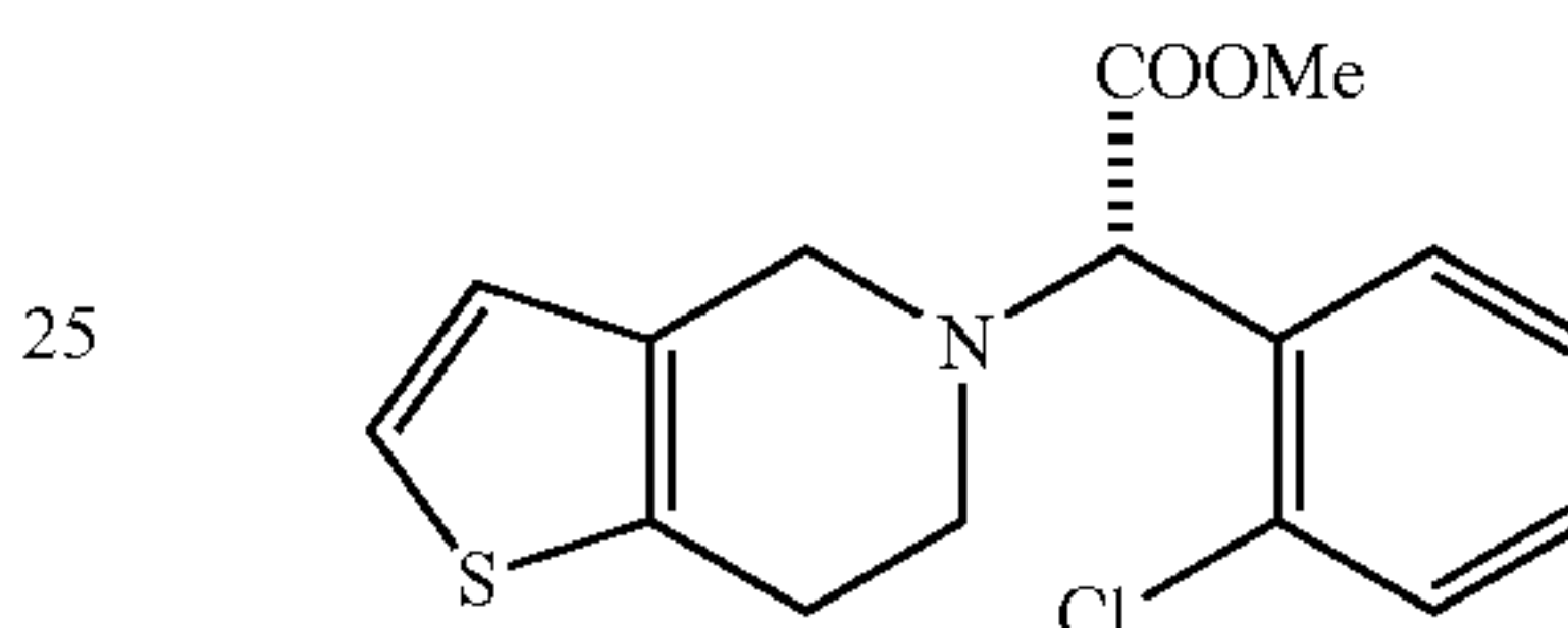
S-Plavix
