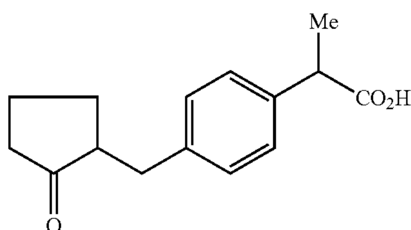
Loxoprofen
