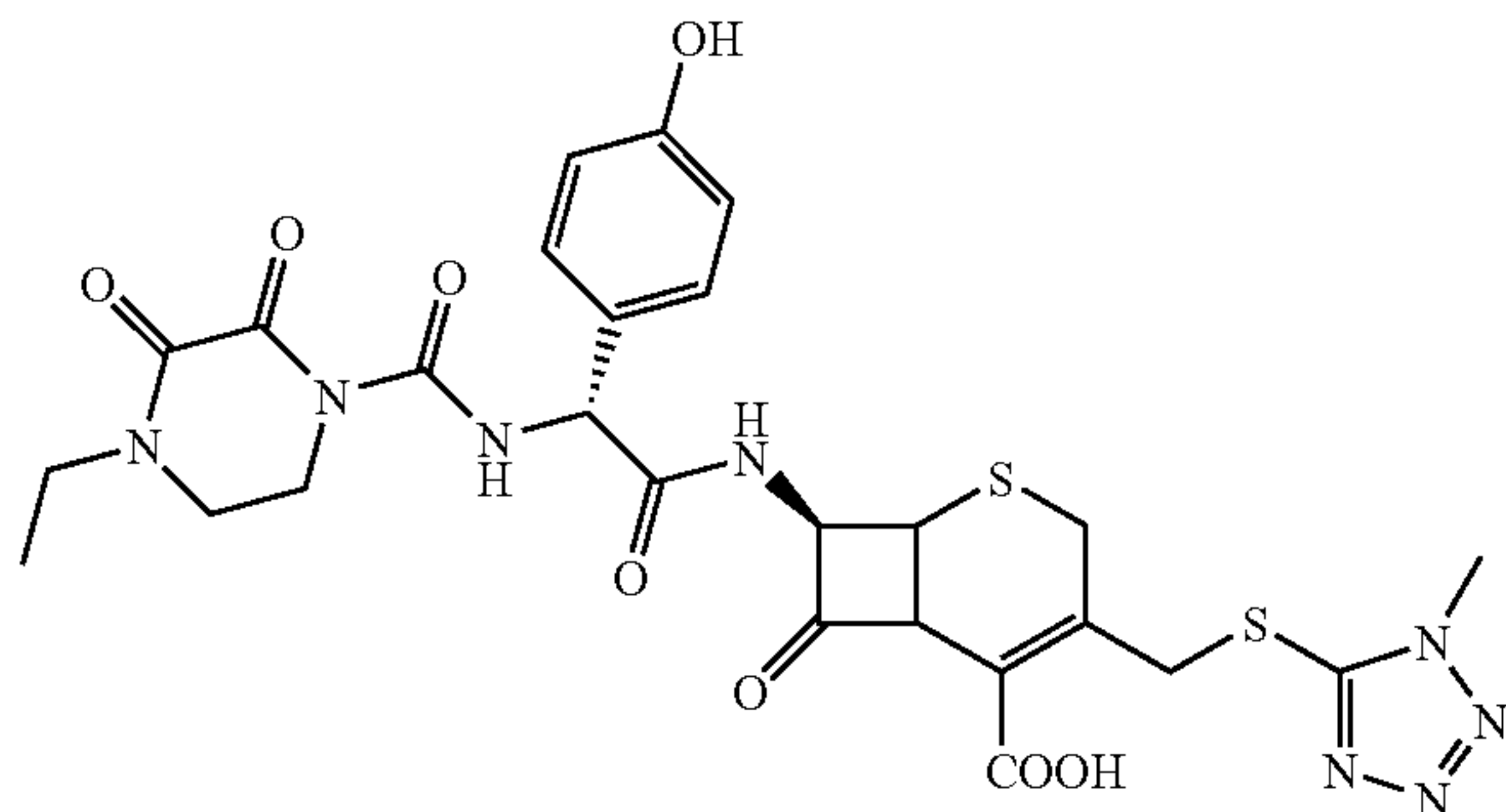
Cefobid
