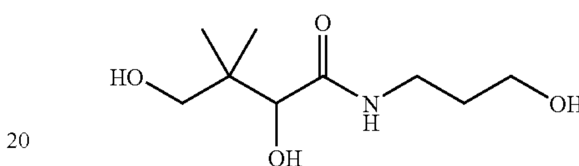
Pantenol
