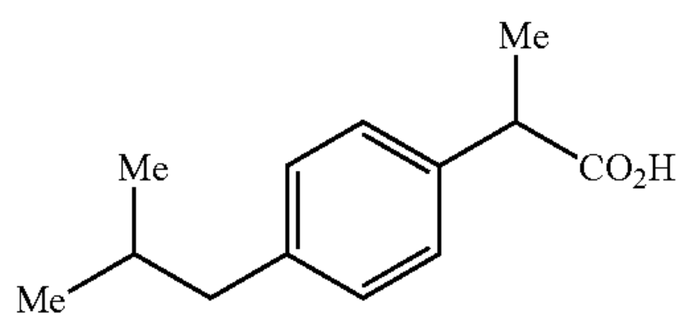
Ibuprofen
