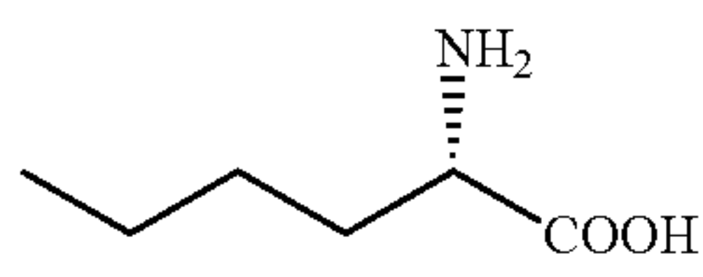
L-norleucine
