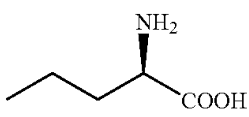
D-norvaline
