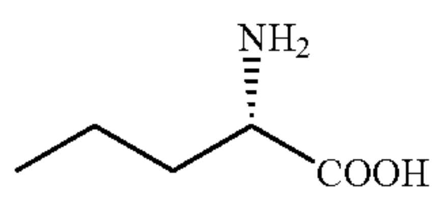
L-norvaline
