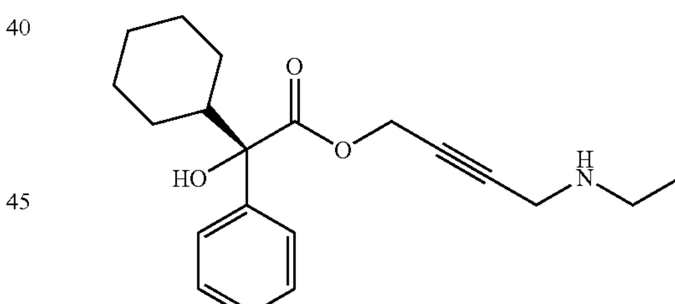
S-Ditropan
