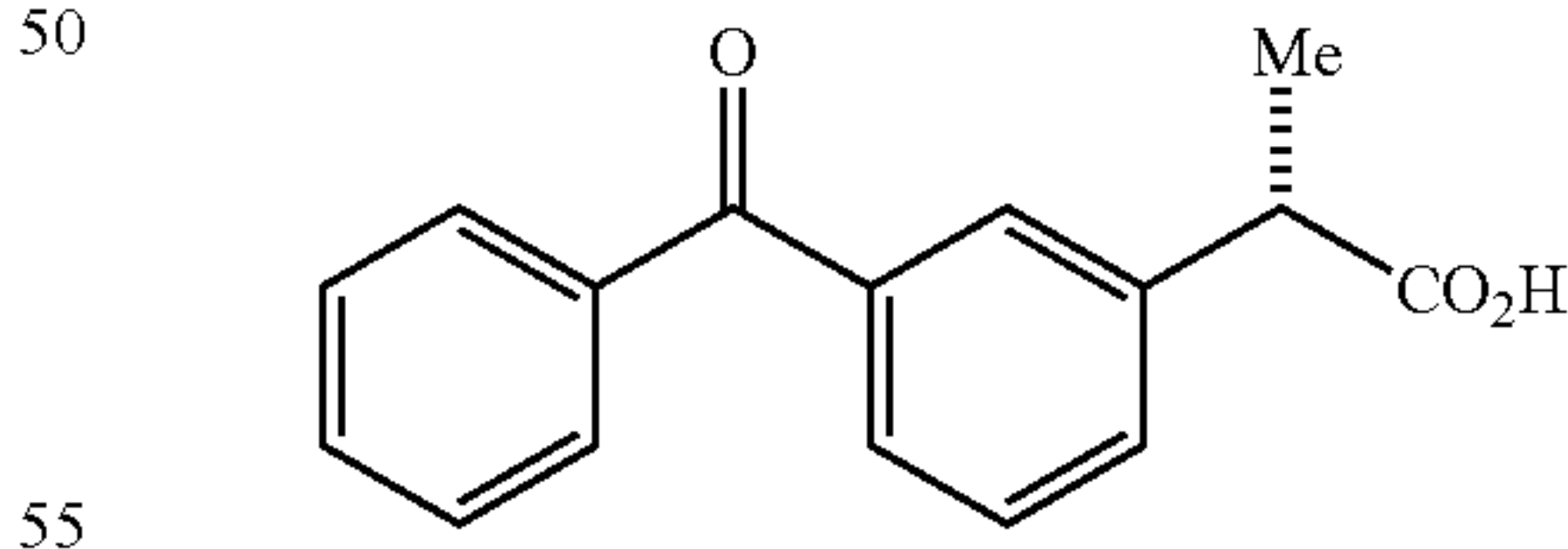
Dexketoprofen
