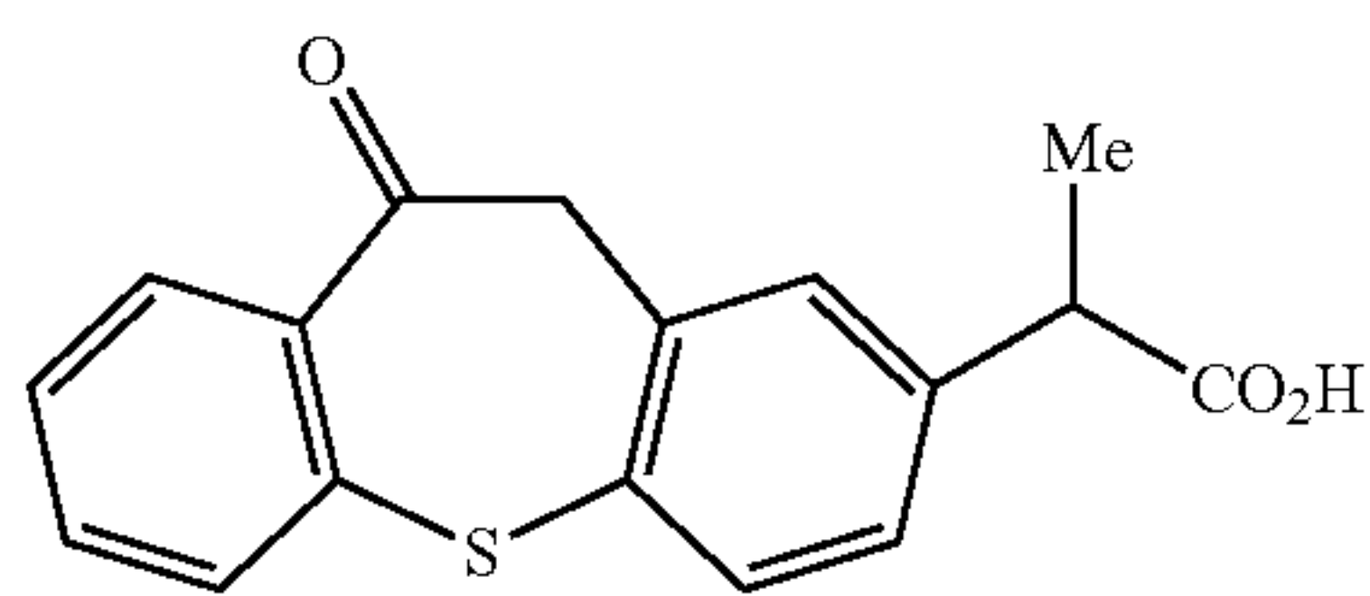
Zaltoprofen
