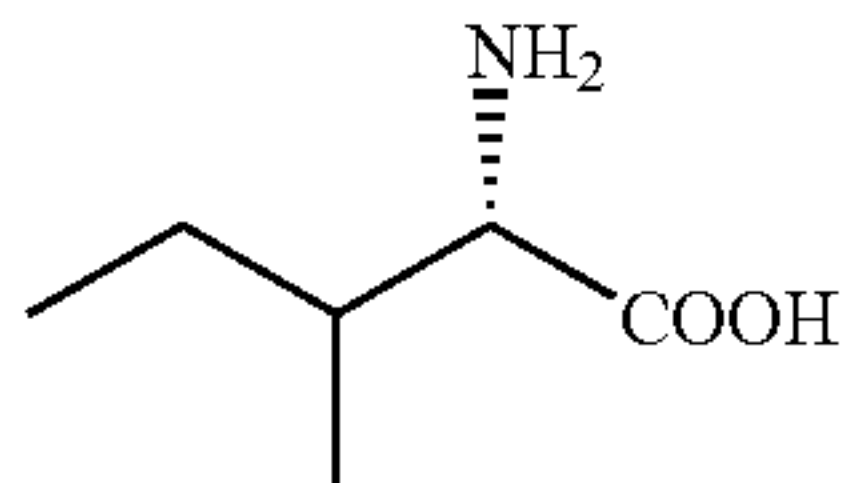
L-isoleucine
