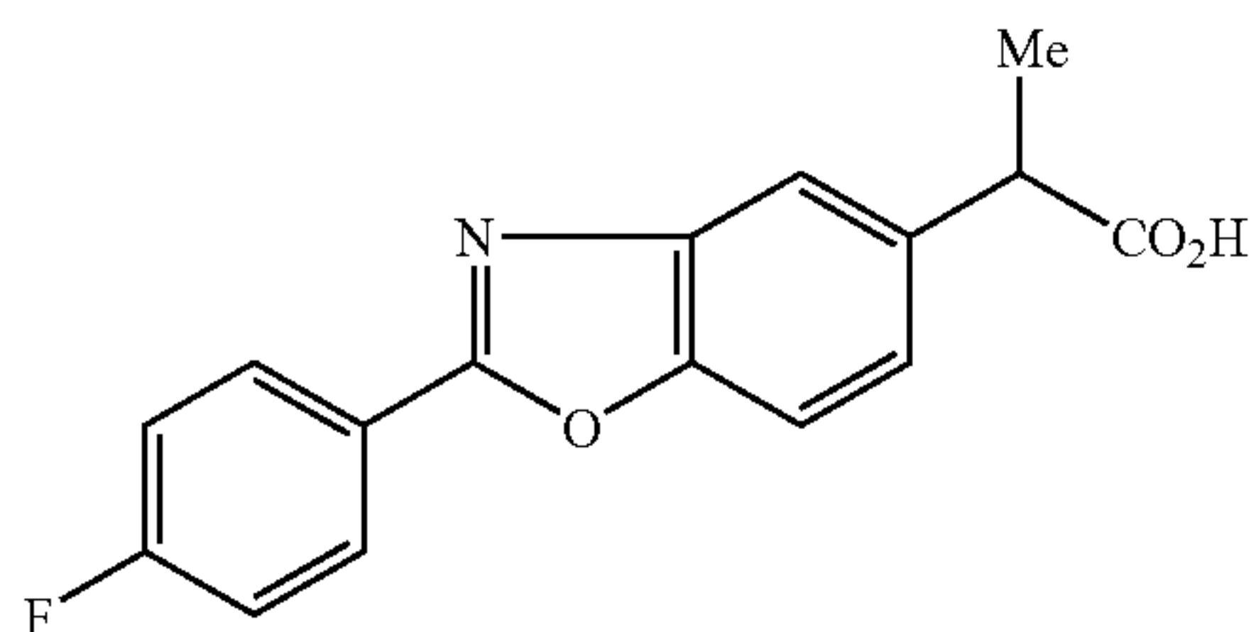
Flunoxaprofen
