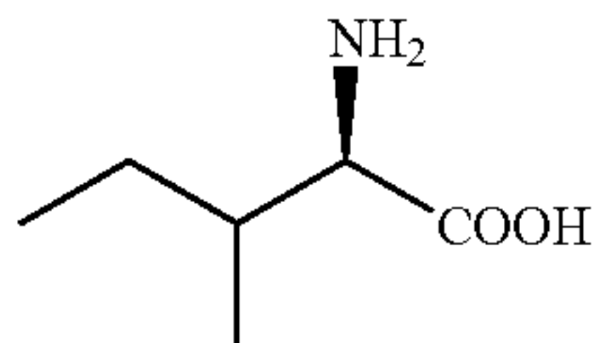
D-isoleucine
