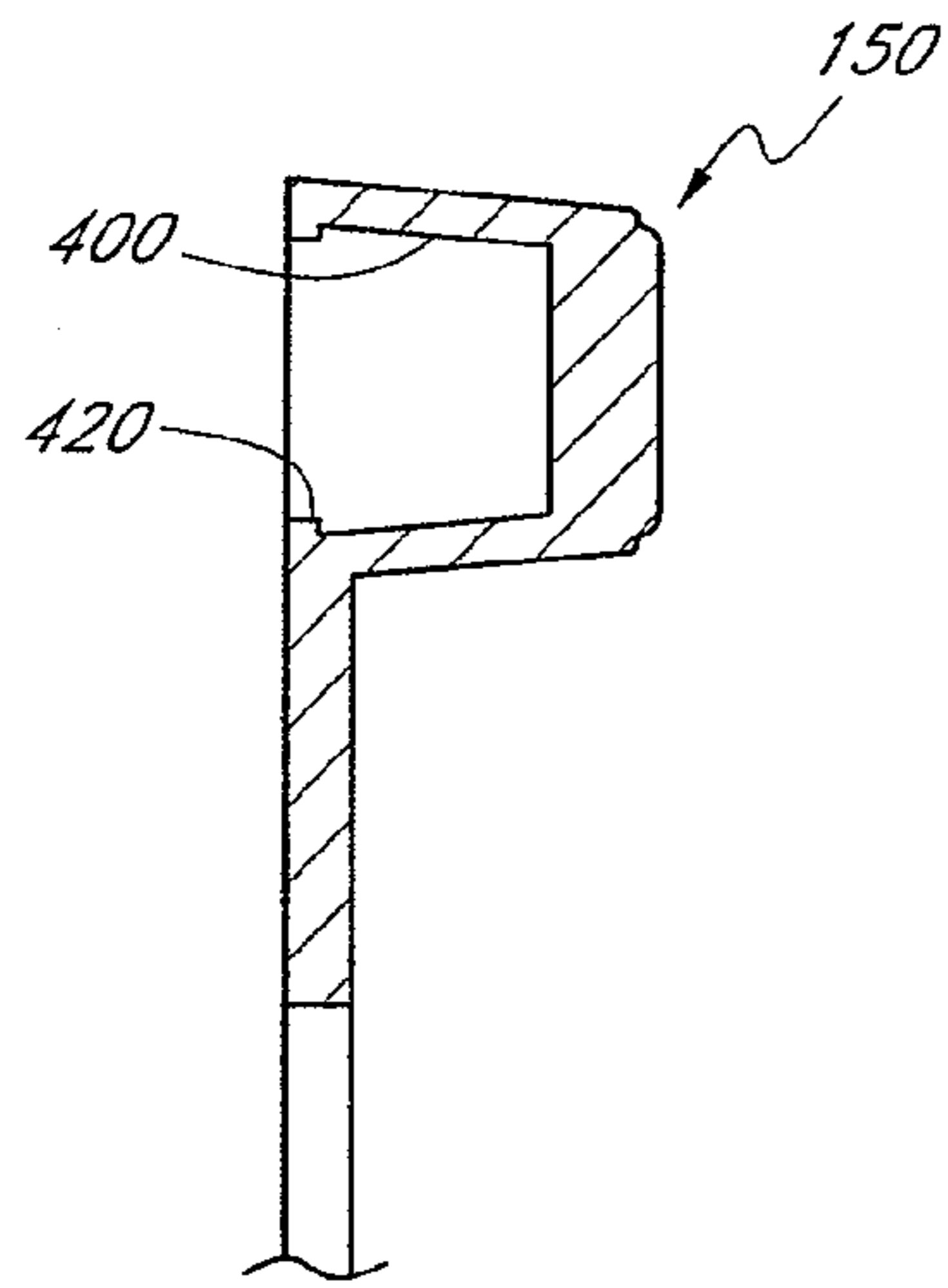
FIG. 6B
