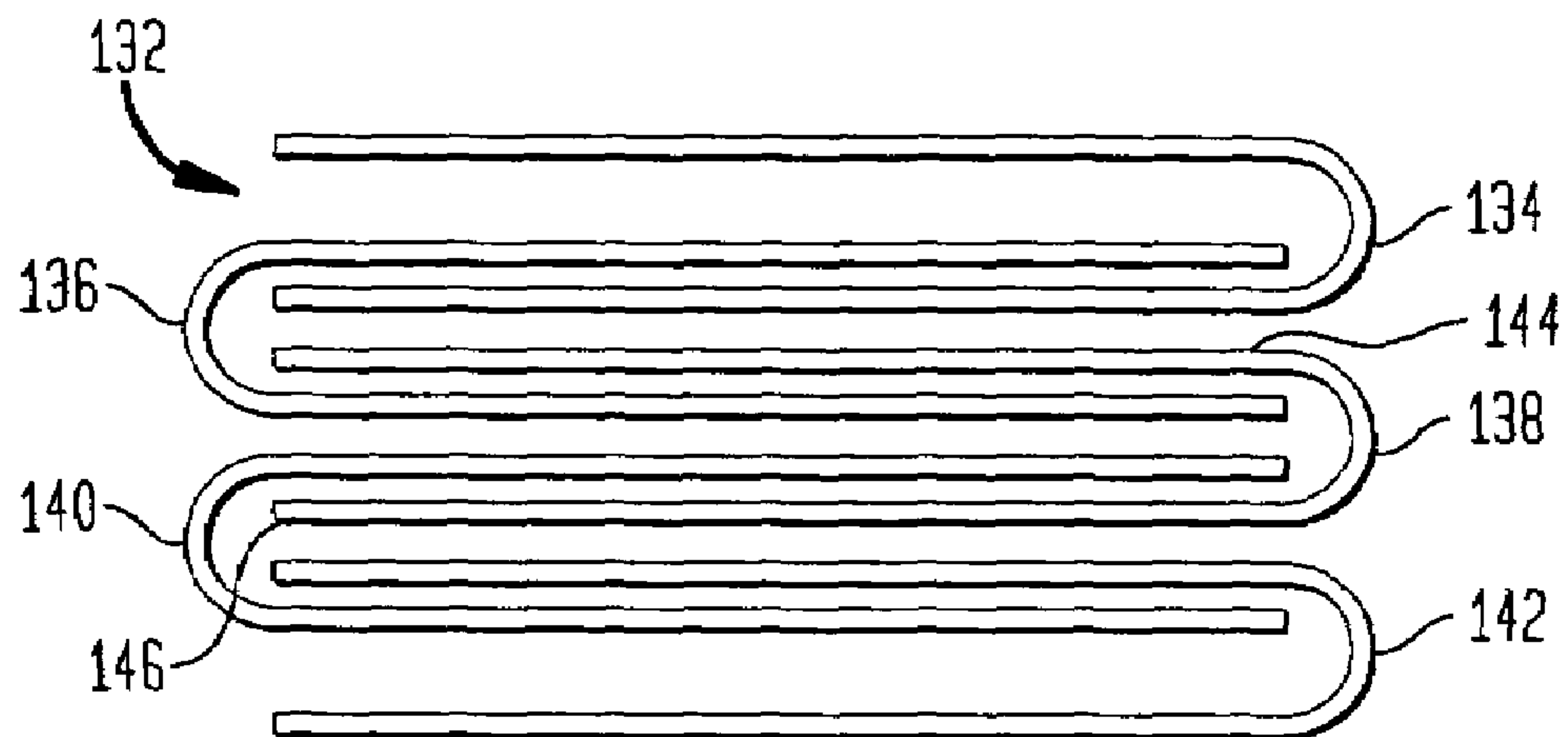
FIG. 9
