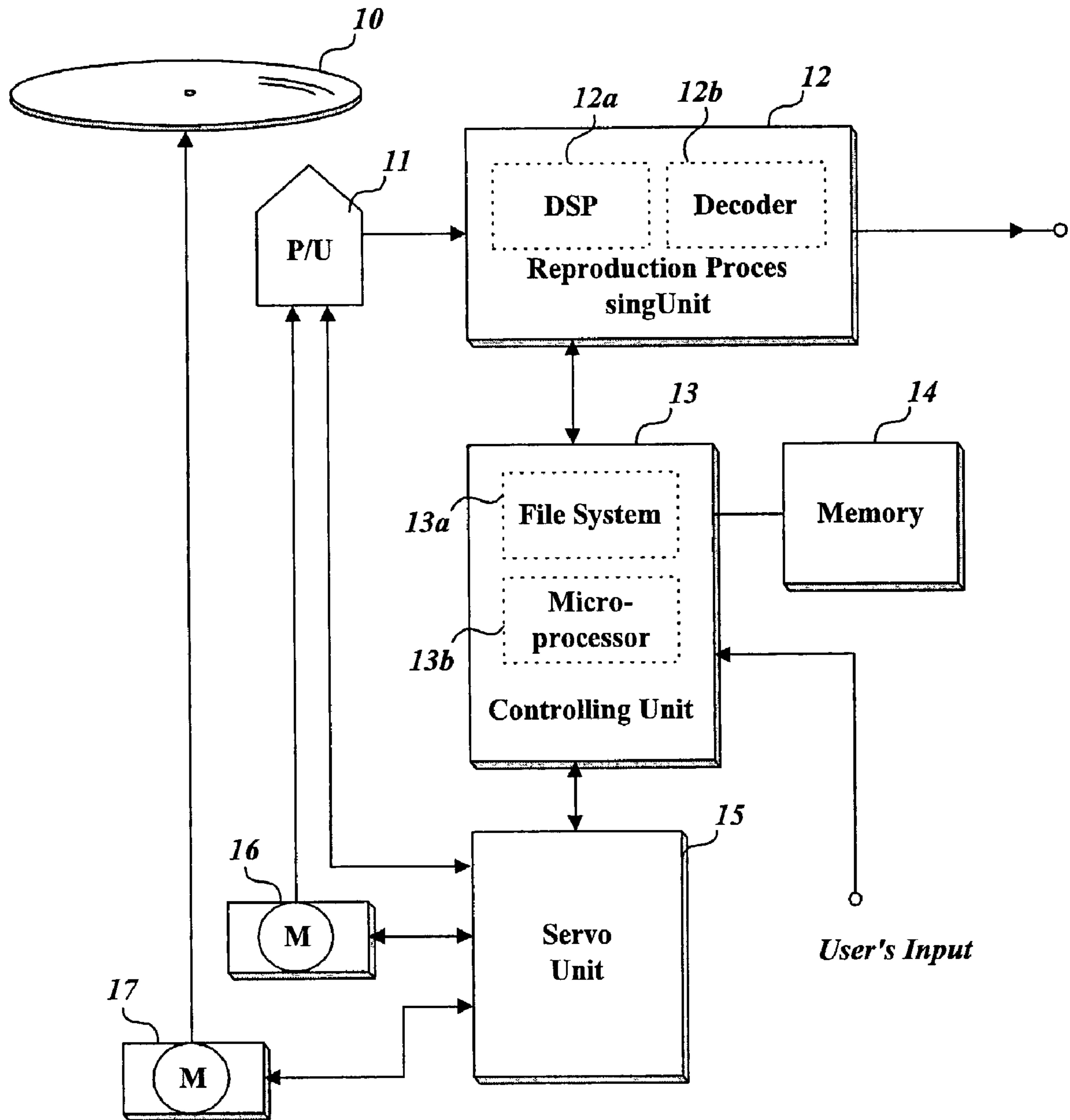
FIG. 10
