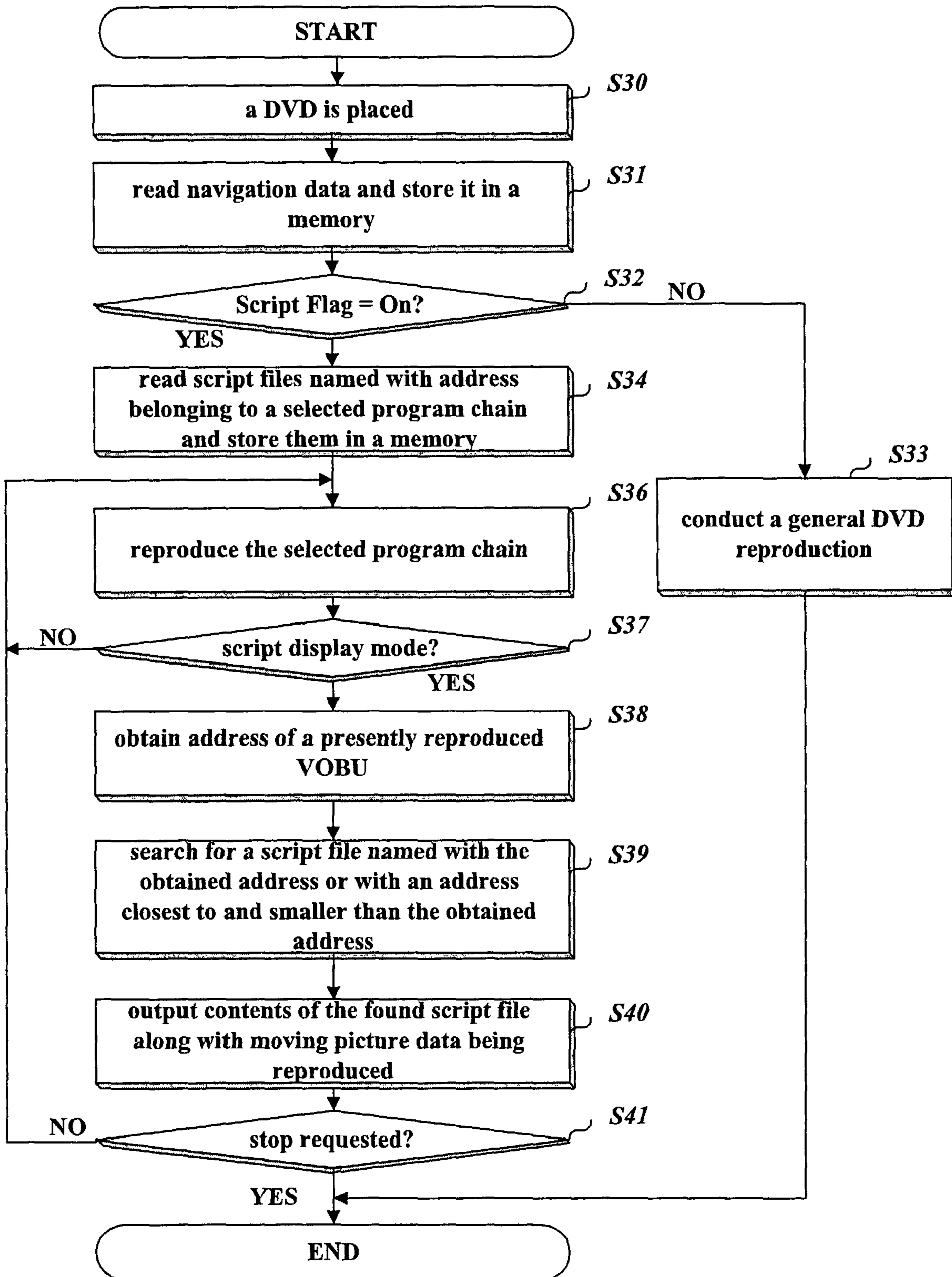
FIG. 13
