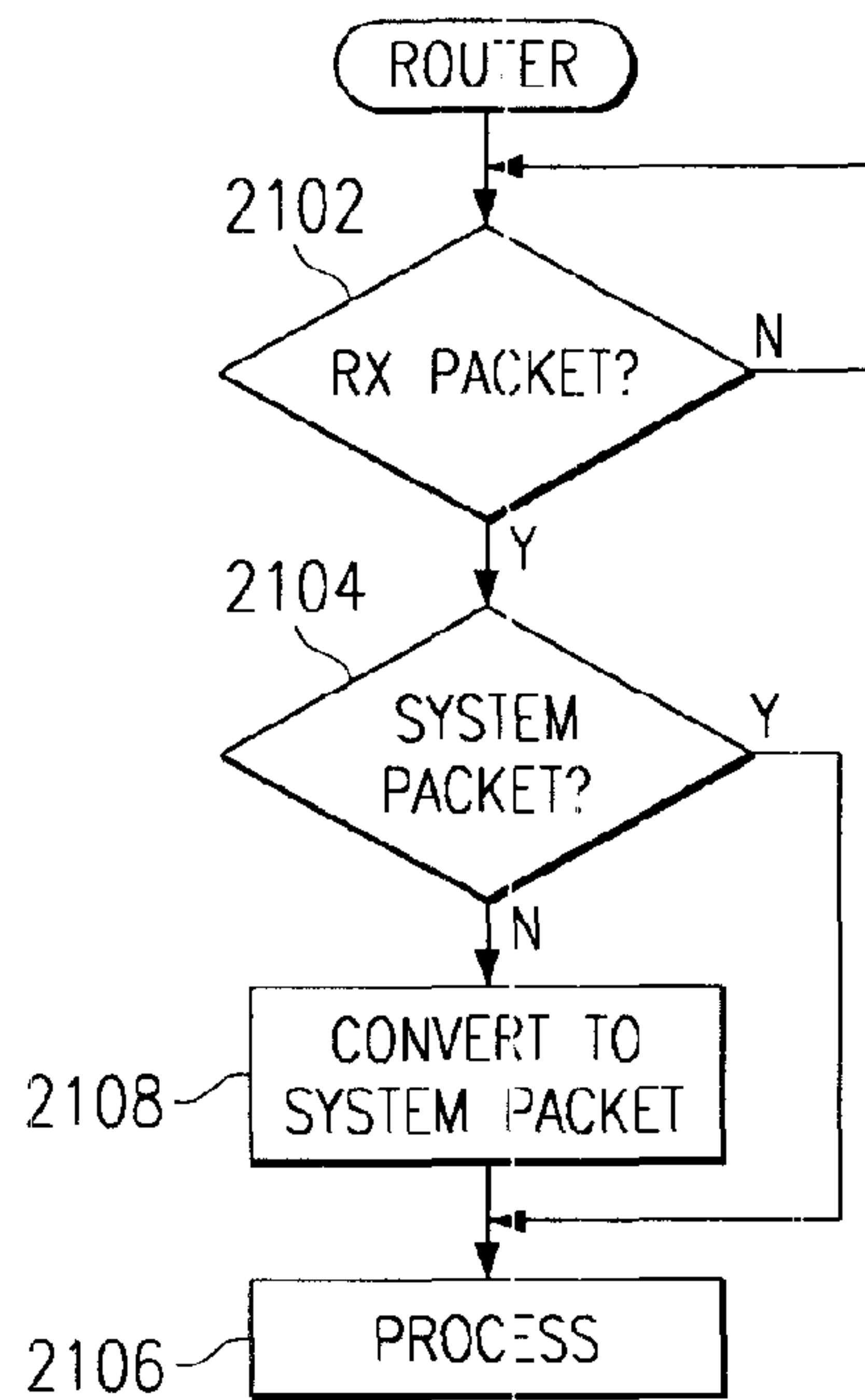
FIG. 21
