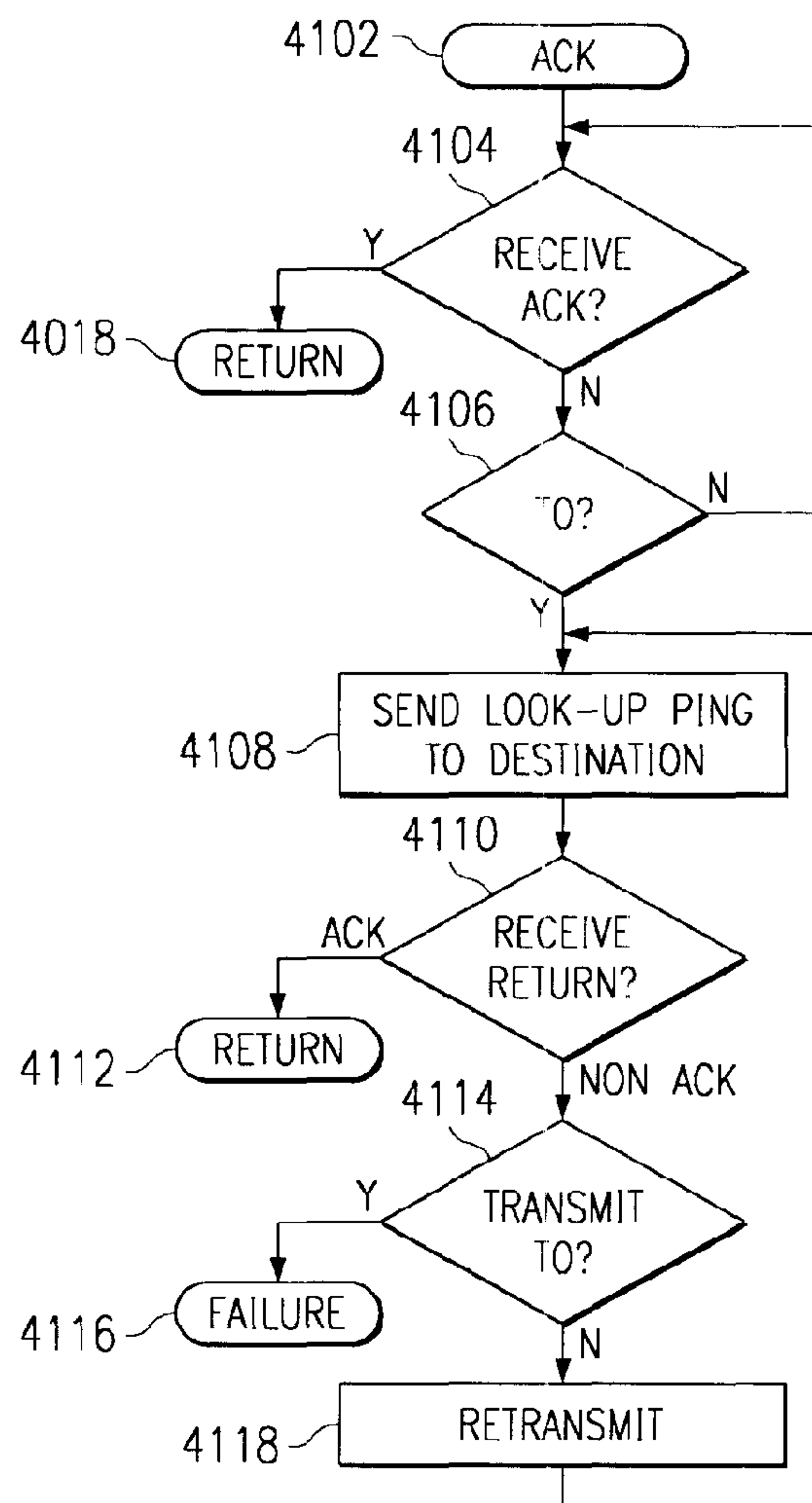
FIG. 41
