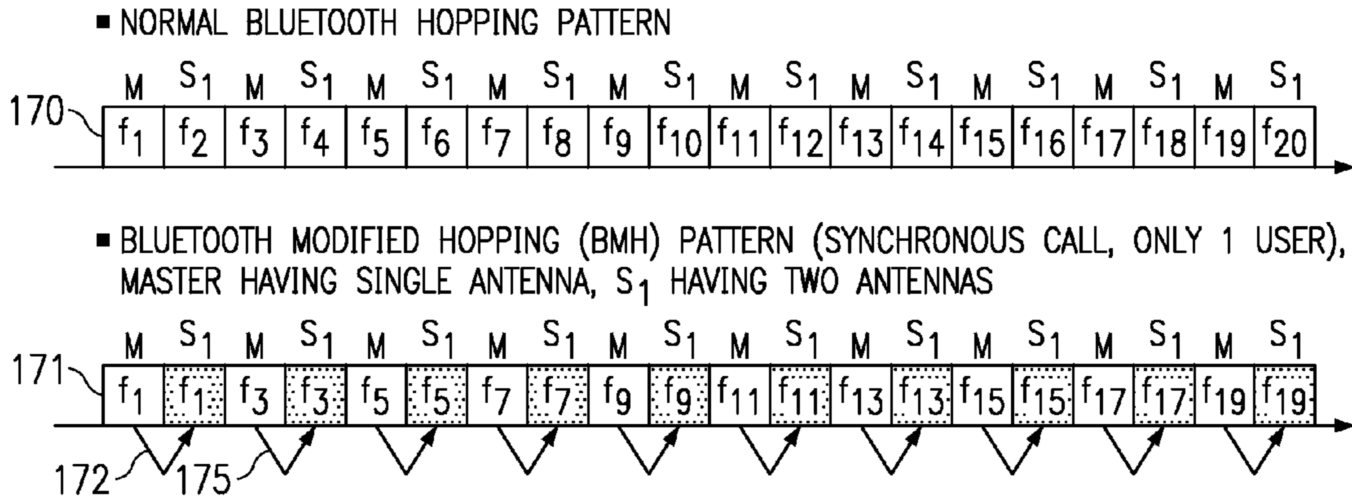
FIG. 17A
