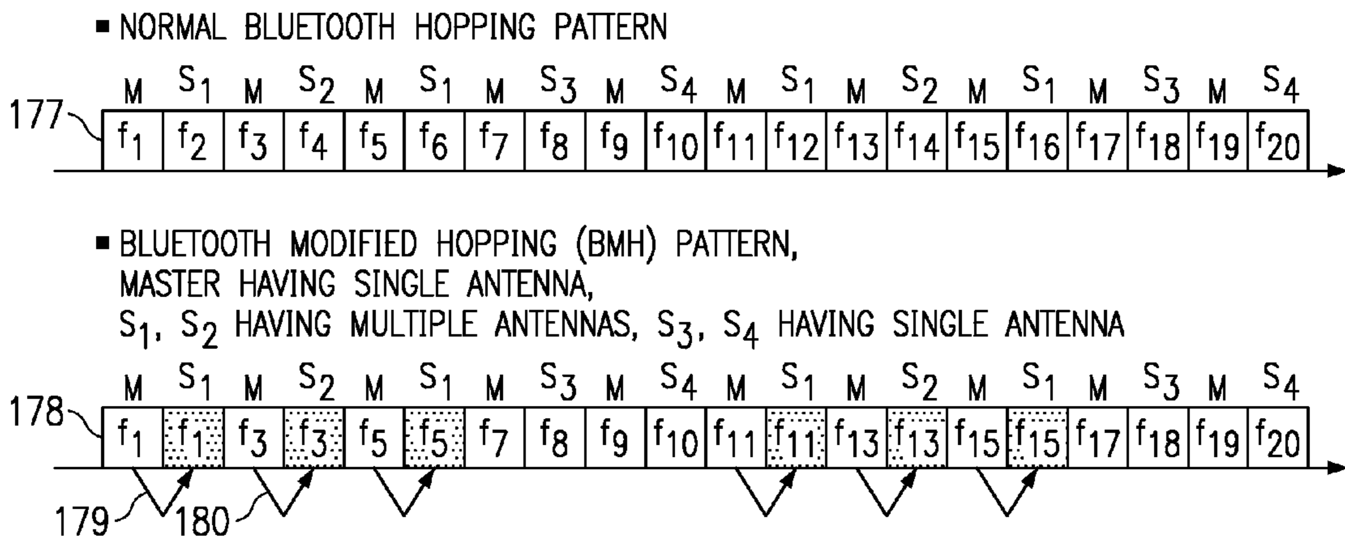
FIG. 17C
