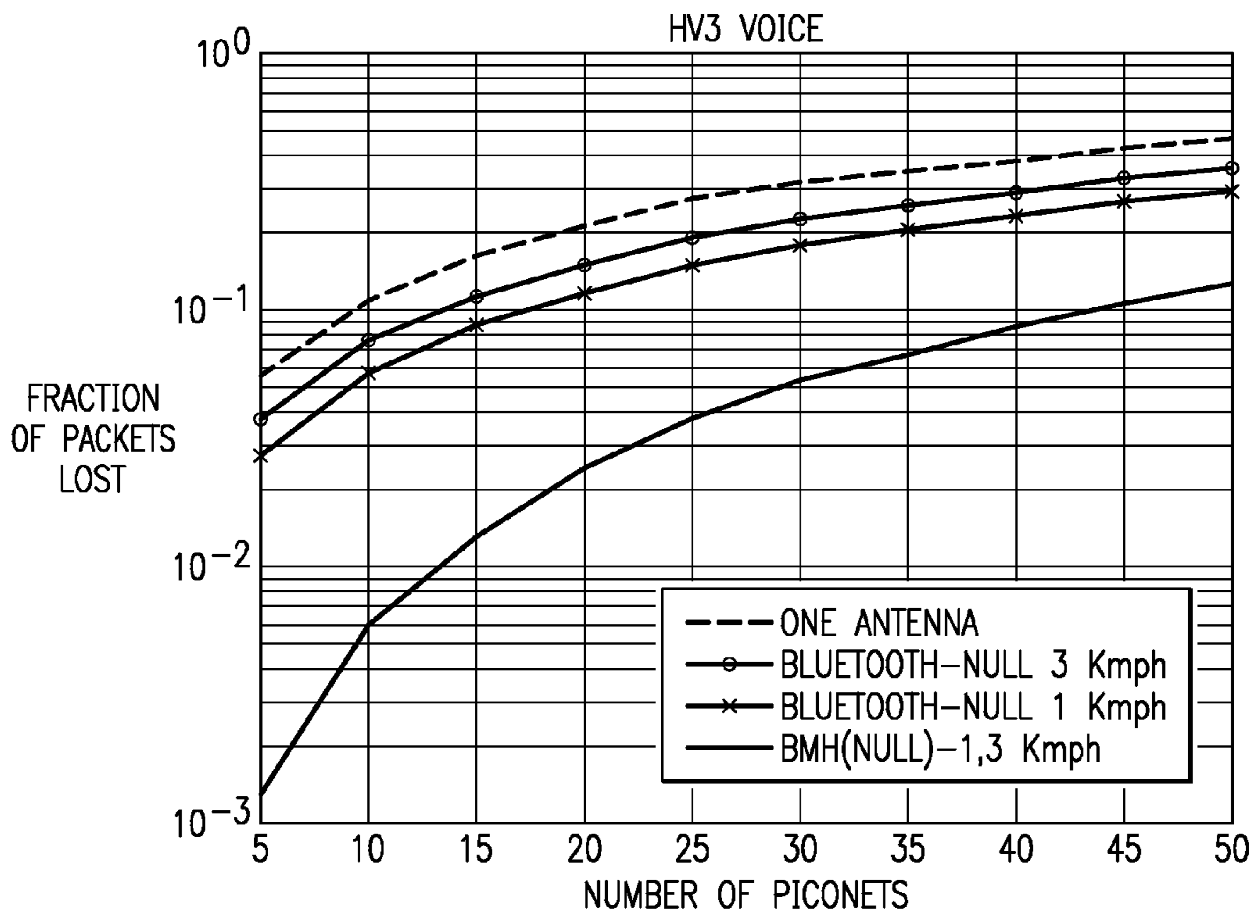
FIG. 16A
