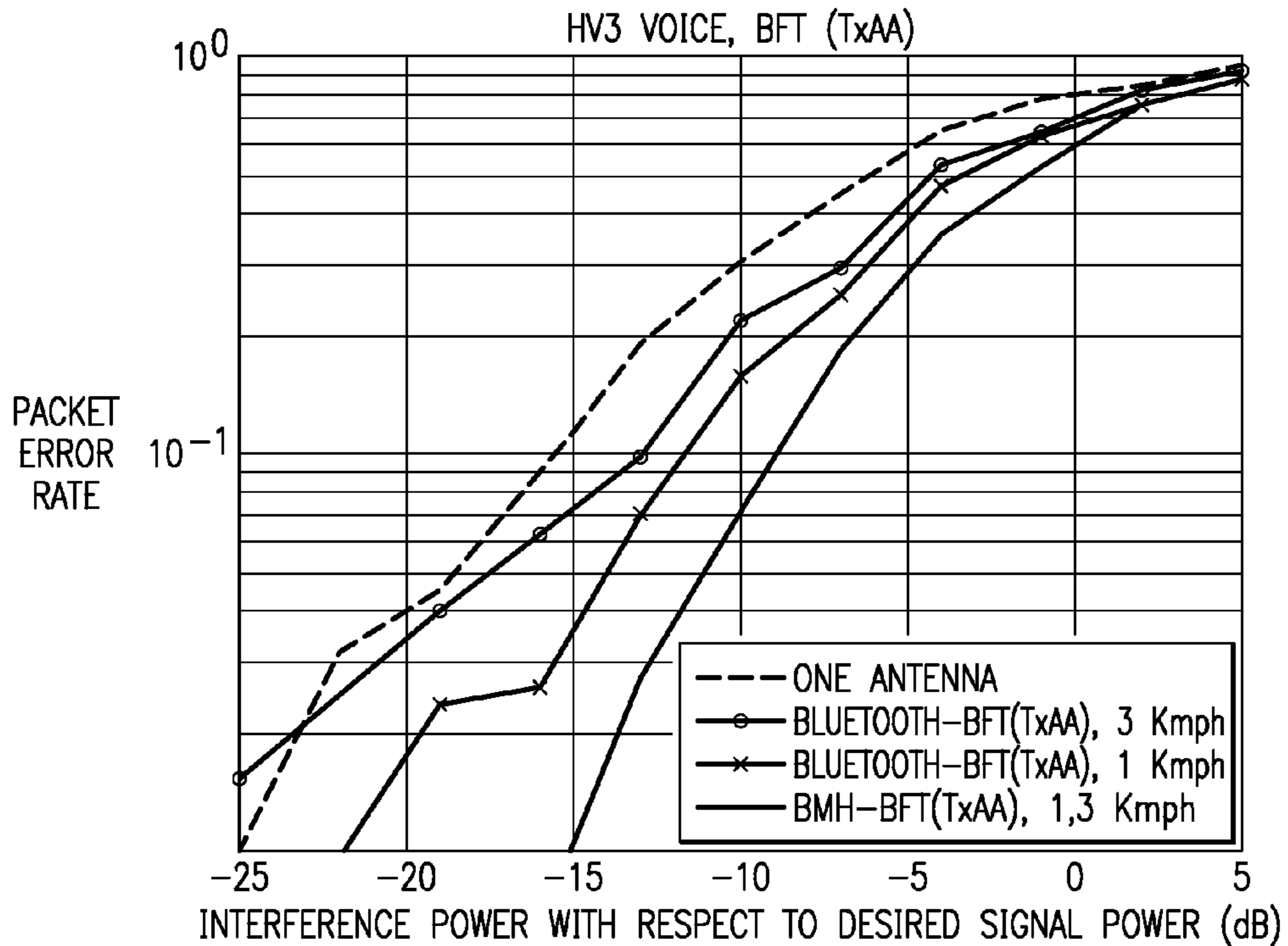
FIG. 13A
