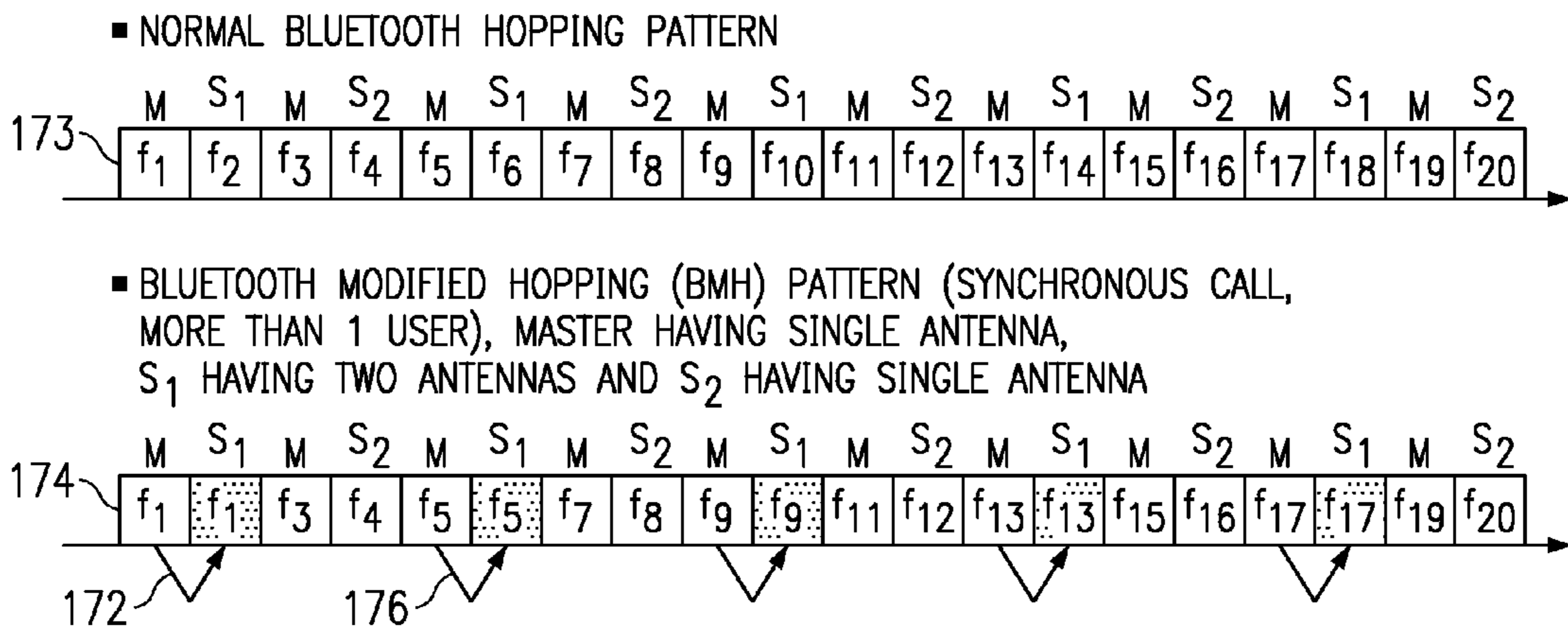
FIG. 17B
