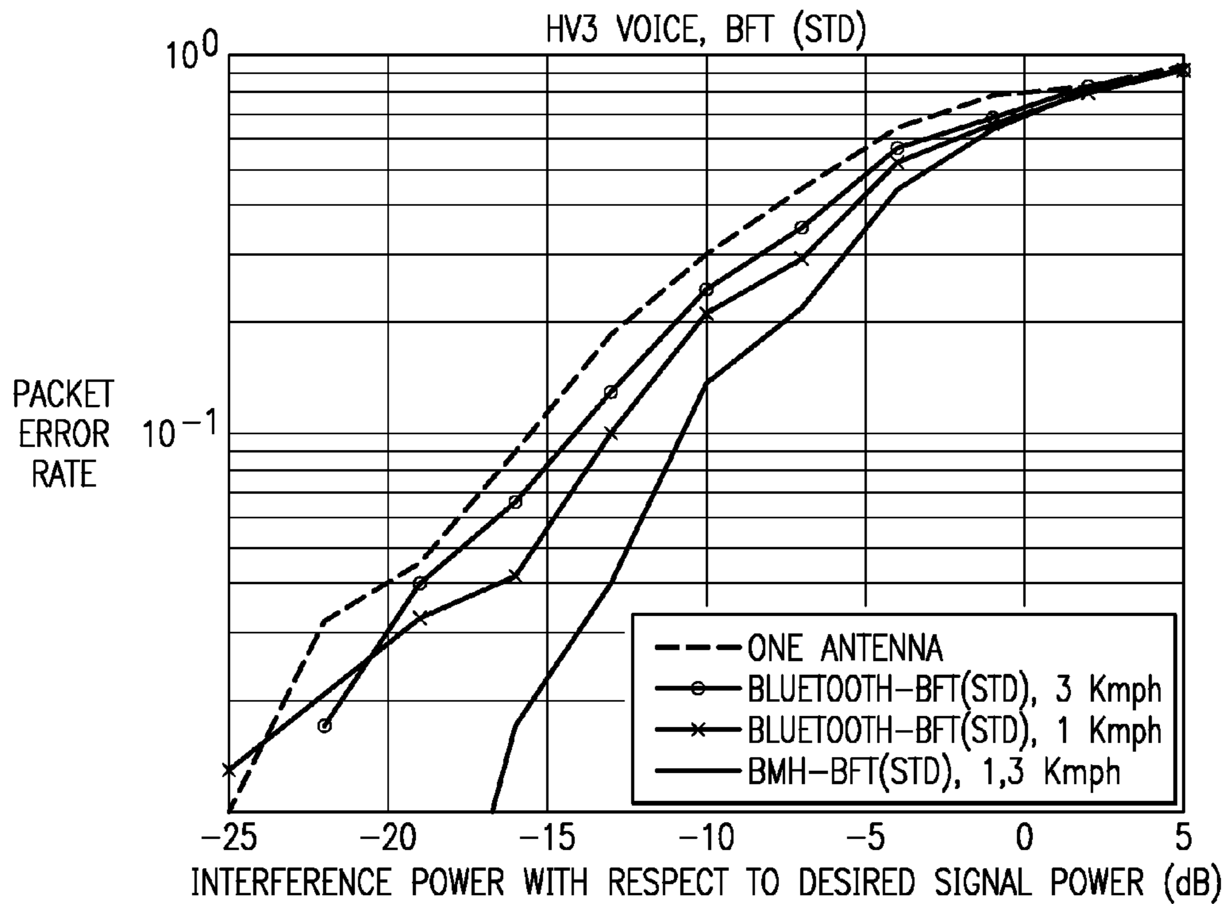
FIG. 14A
