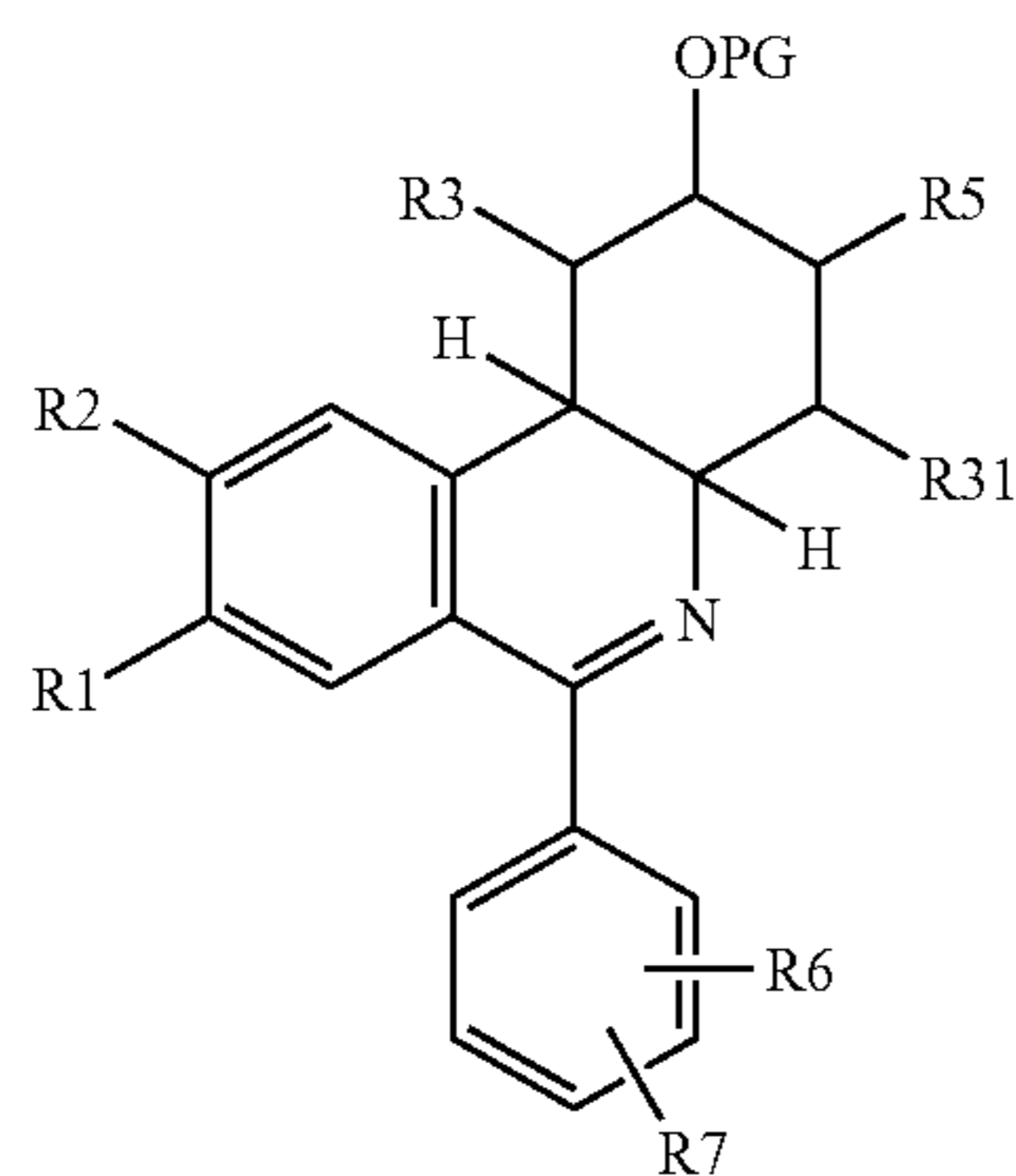
(Ia)
