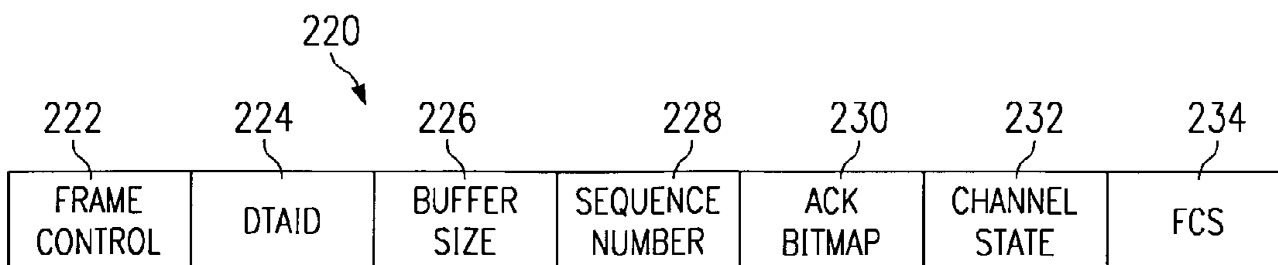
FIG. 13
