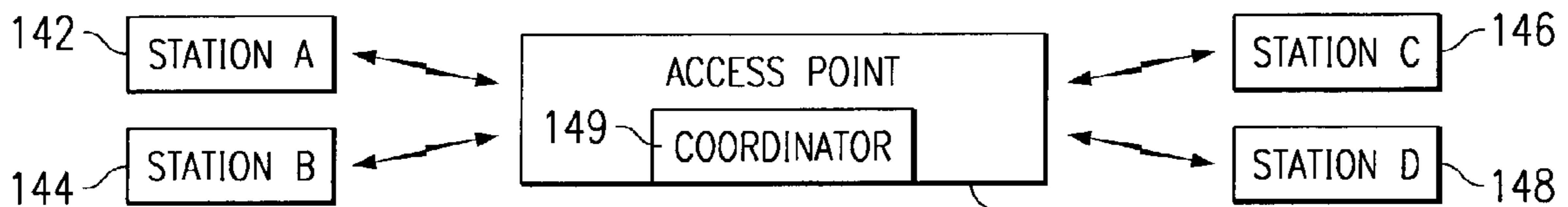
FIG. 7
