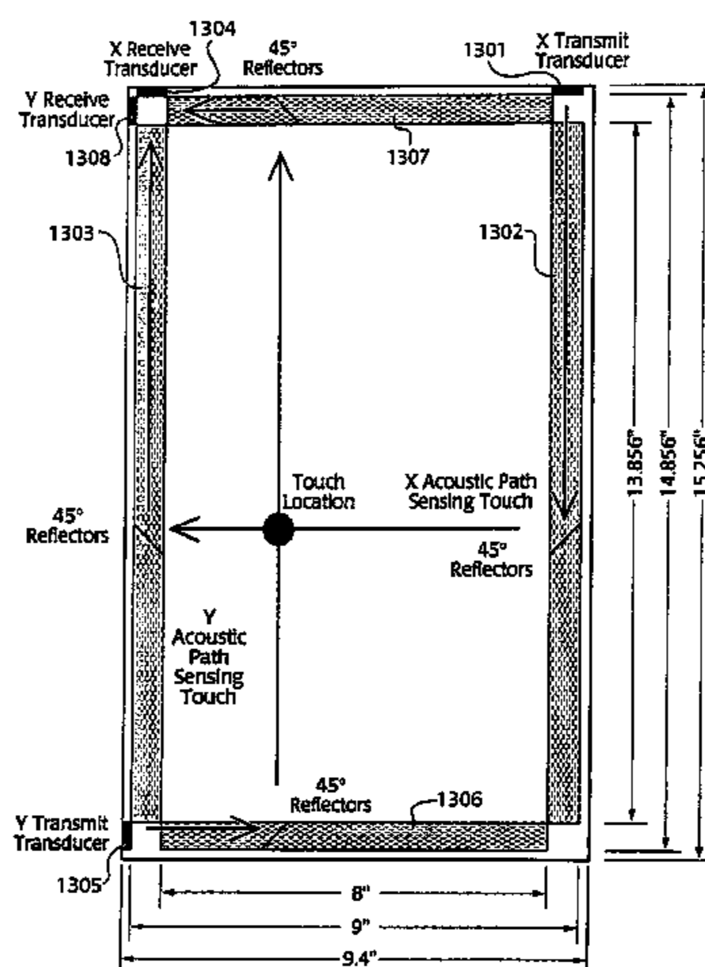
X, Y, 30° Sensor: (a) X & Y Subsystems
