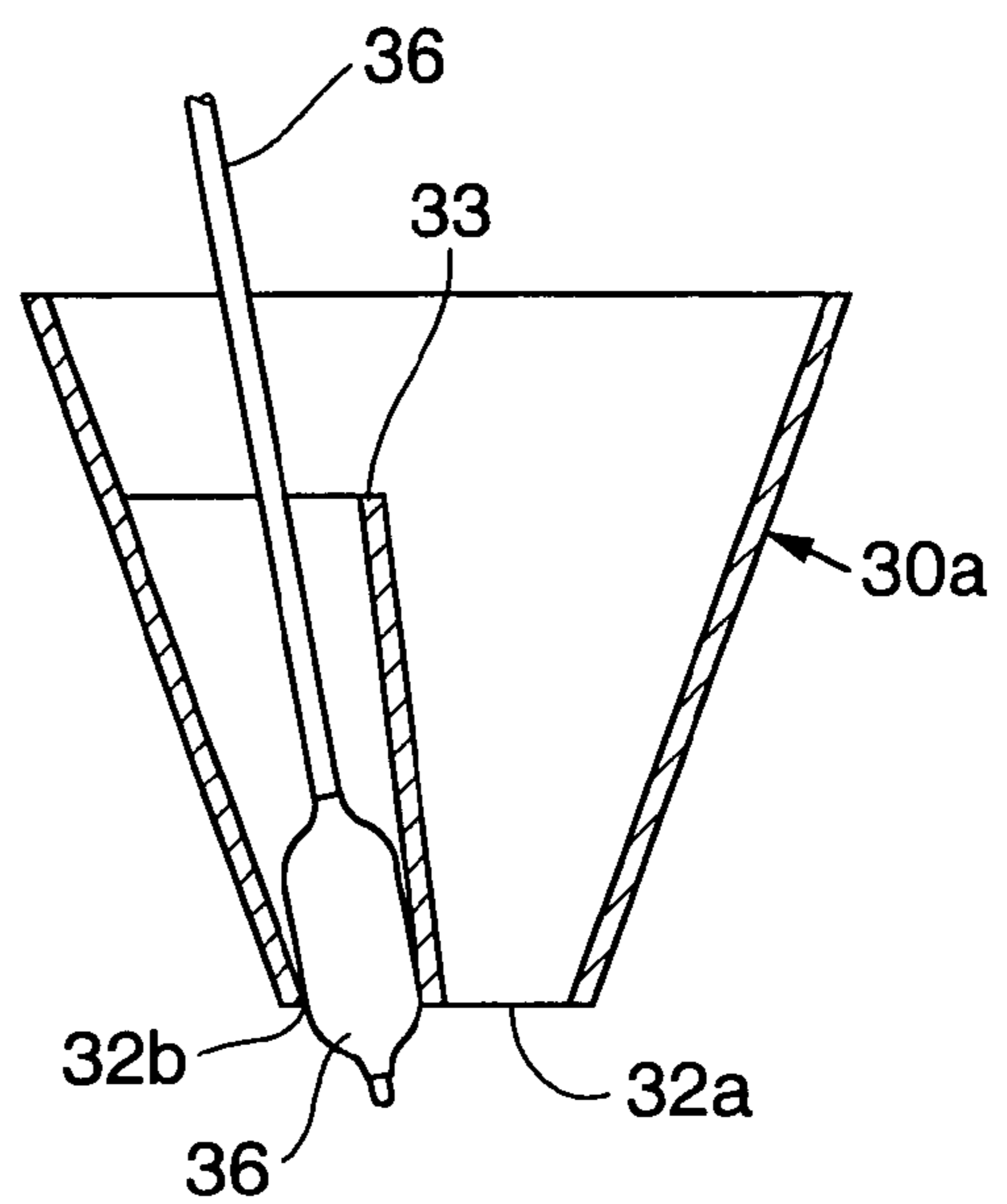
FIG. 20B
