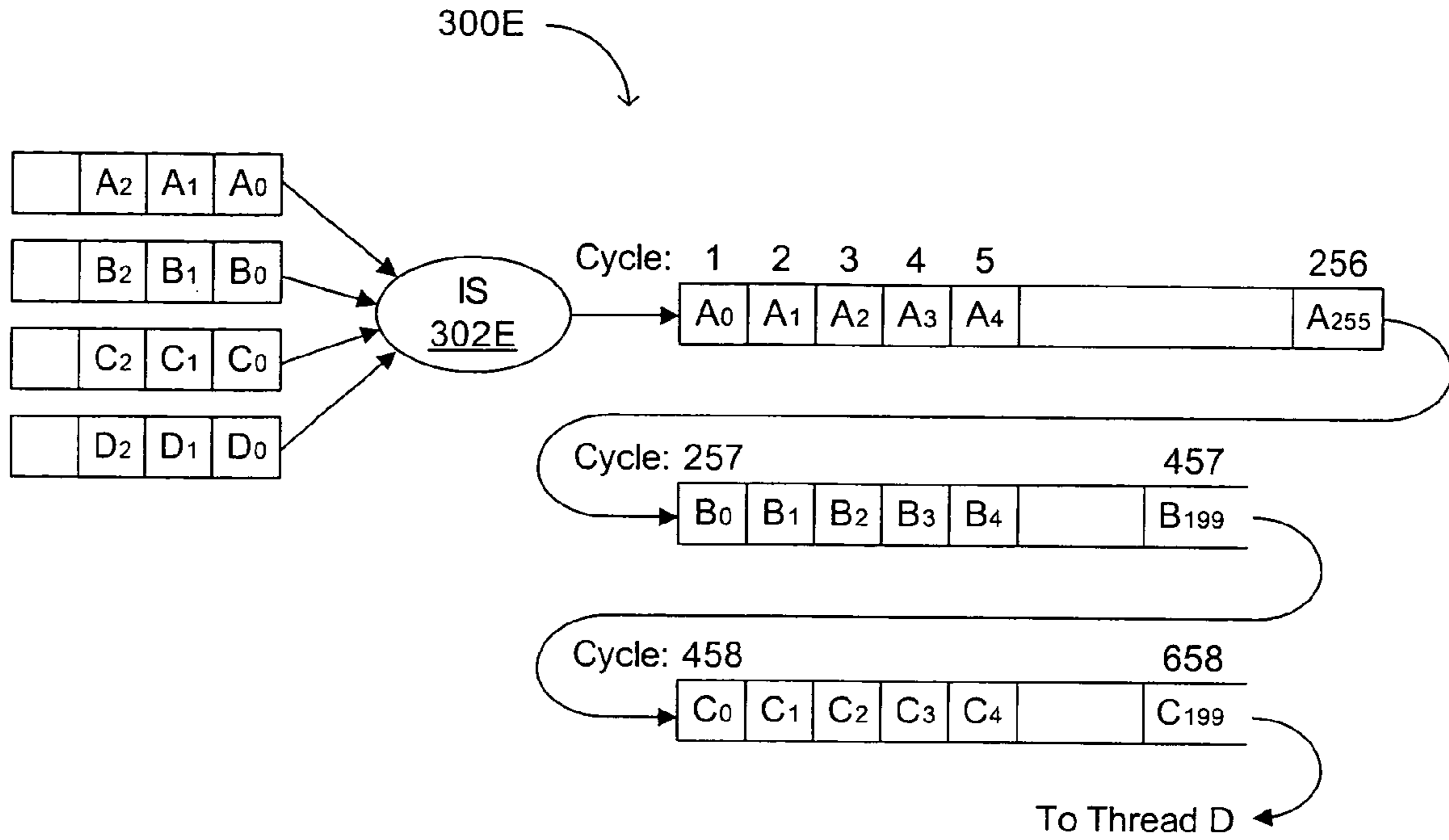
FIG. 3E
