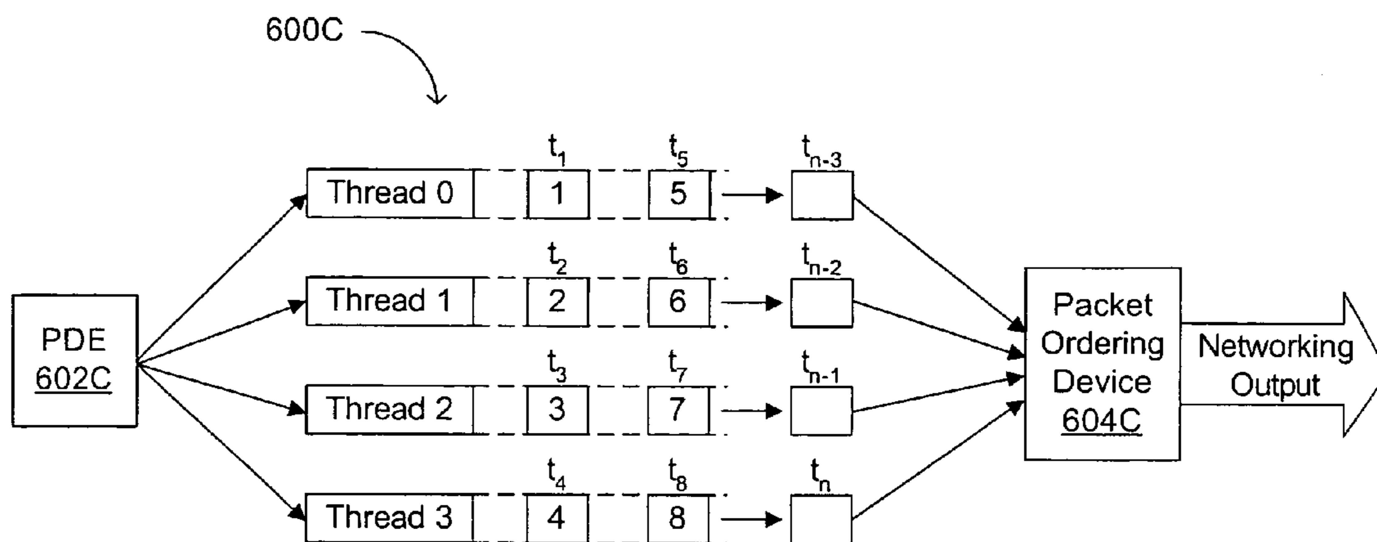
FIG. 6C
