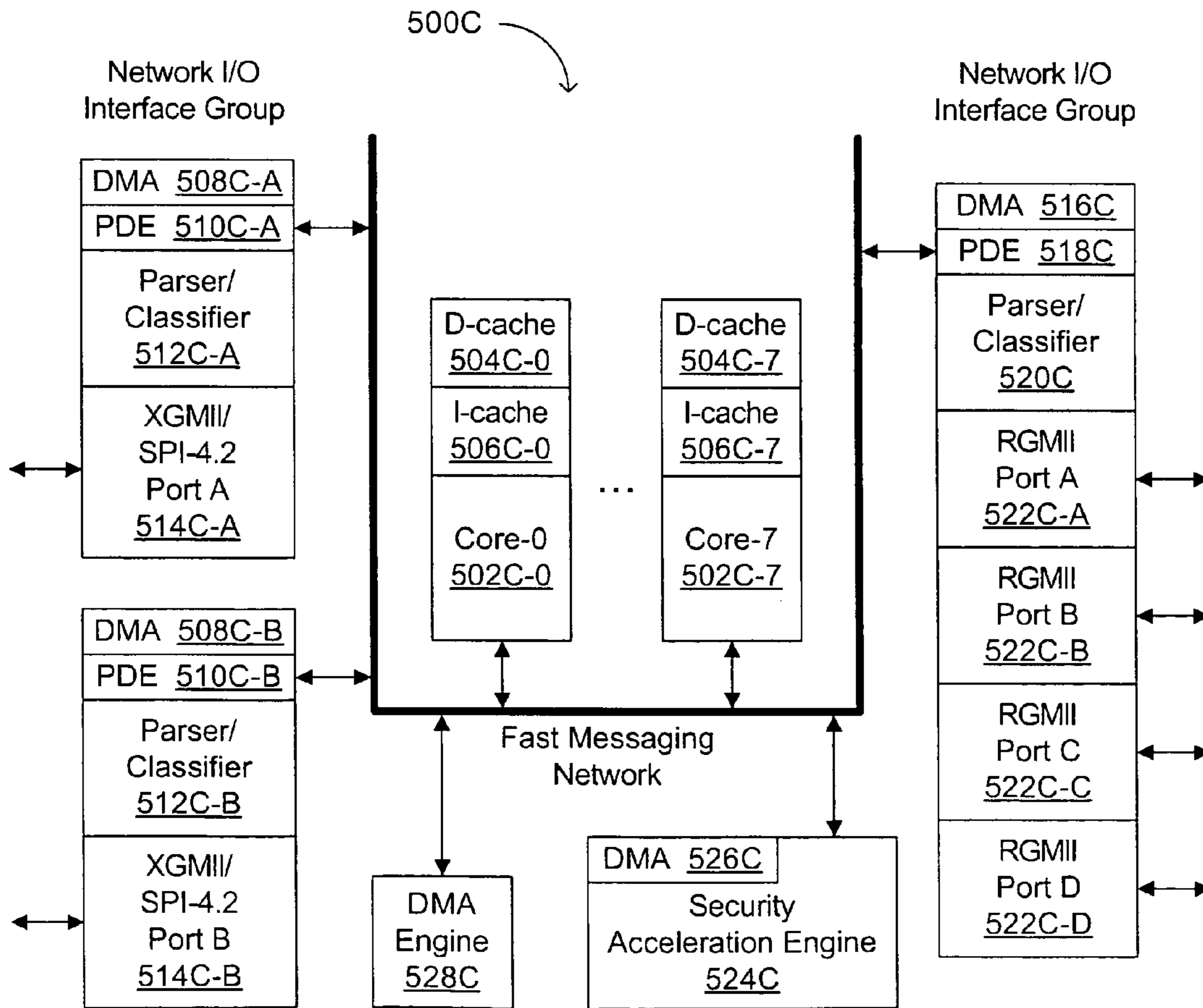
FIG. 5C
