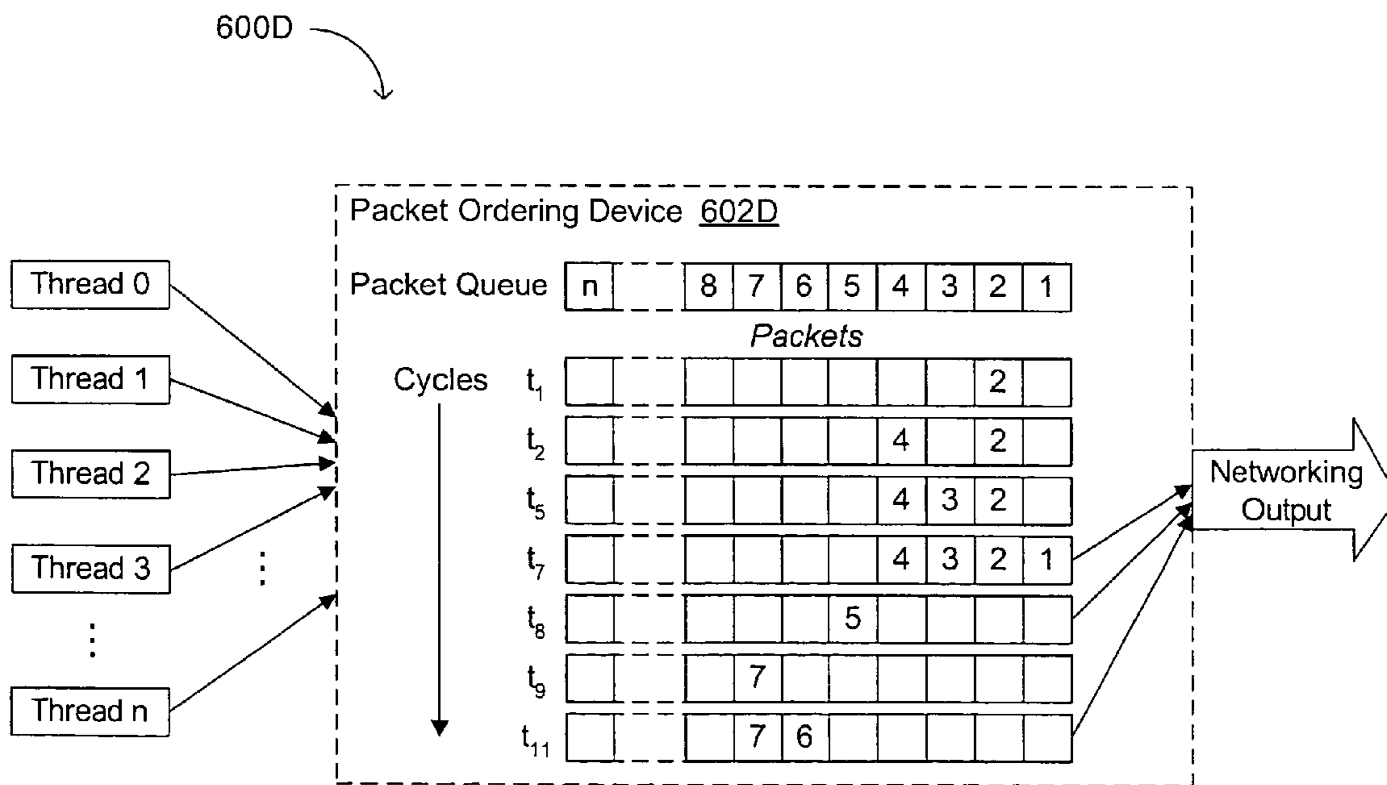
FIG. 6D
