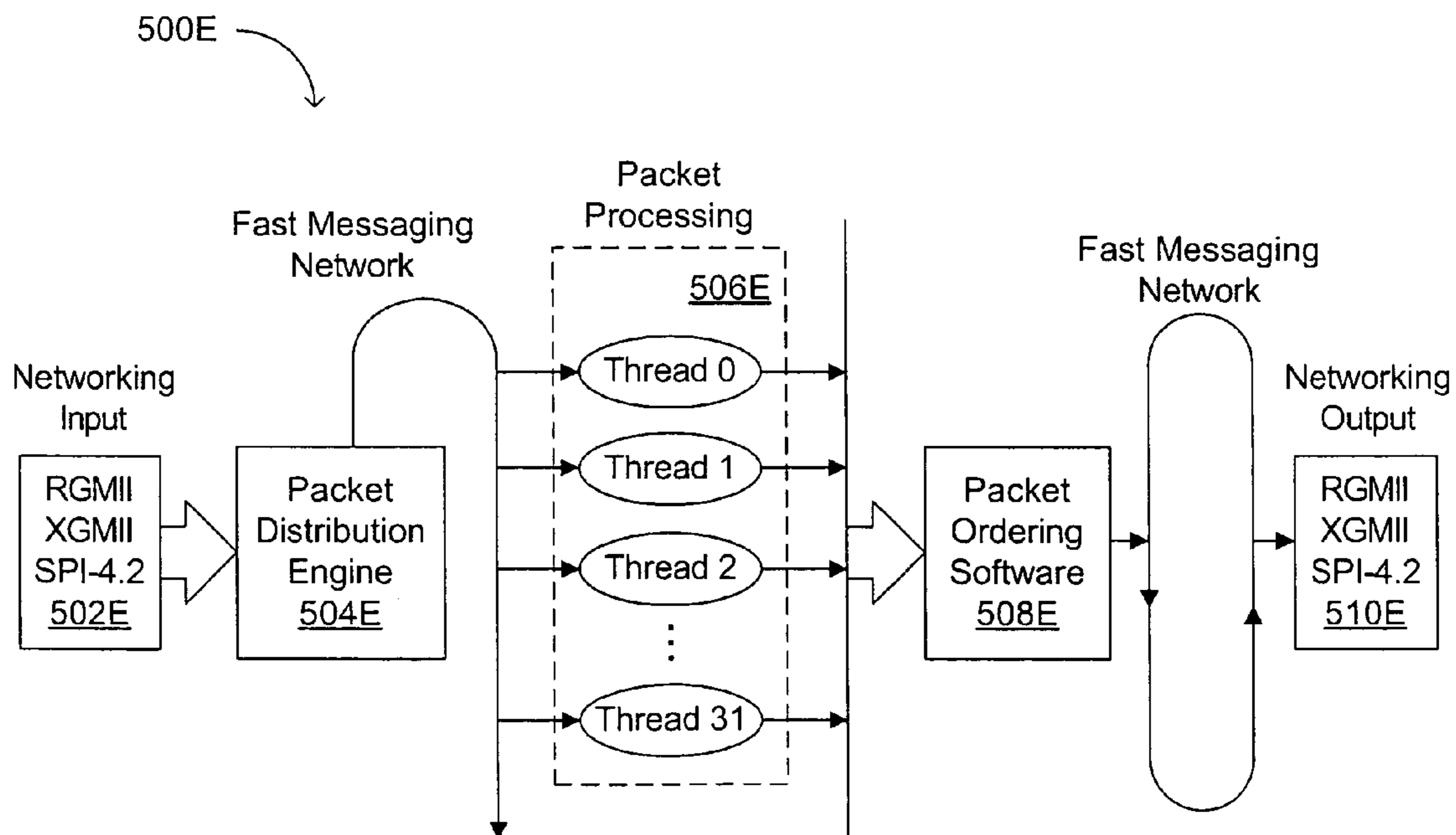
FIG. 5E
