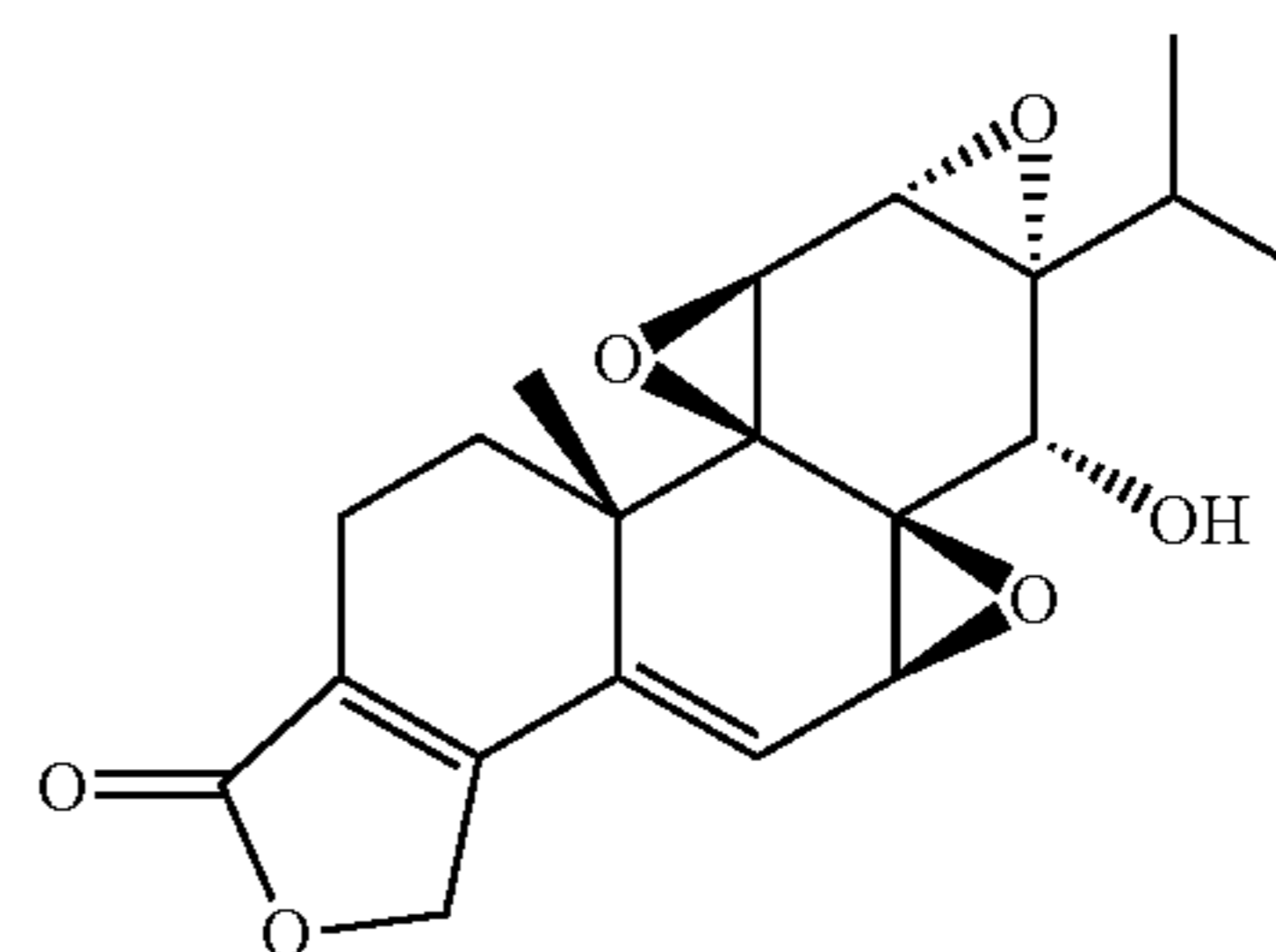
\Delta^{5,6} -dehydro-14-epitriptolide
