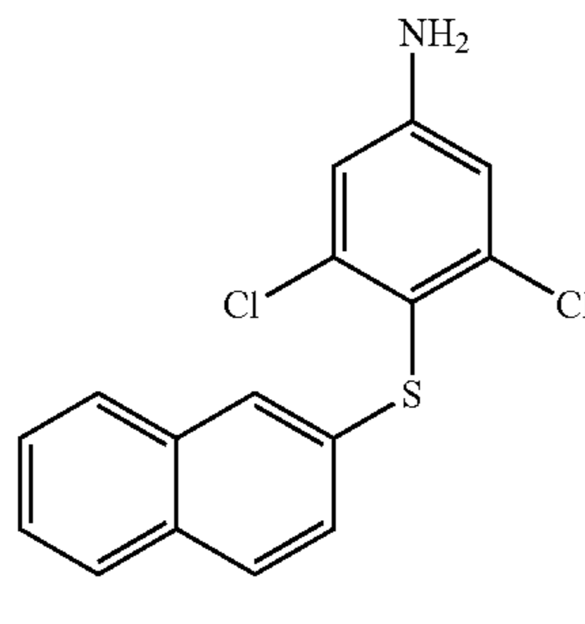
3,5-dichloro-4-(naphthalen-2-ylsulfanyl)-phenylamine (90)
