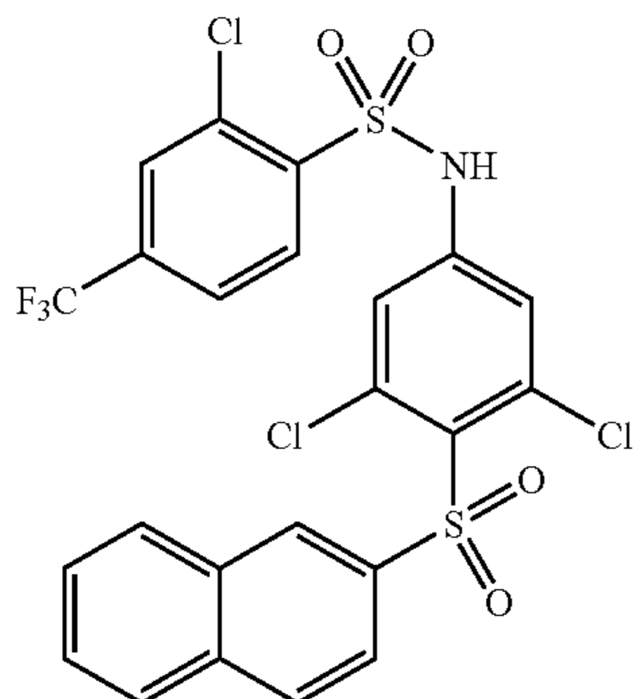
2-Chloro-N-[3,5-dichloro-4-(naphthalene-2-sulfonyl)-phenyl]-4-trifluoromethylbenzenesulfonamide (107)
