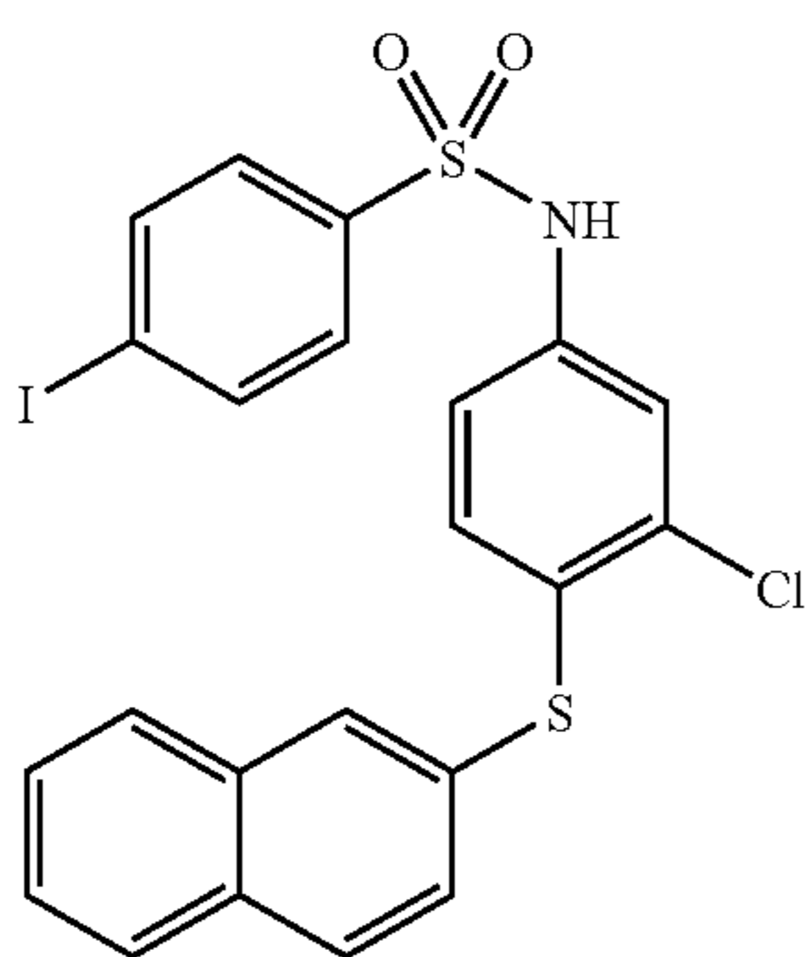
N-[3-Chloro-4-(naphthalen-2-ylsulfanyl)-phenyl]-4-iodobenzenesulfonamide (100)
