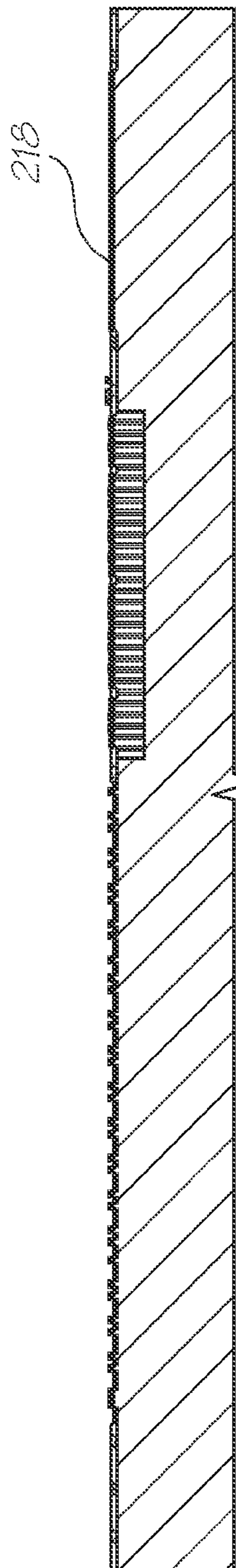
p+ implant
