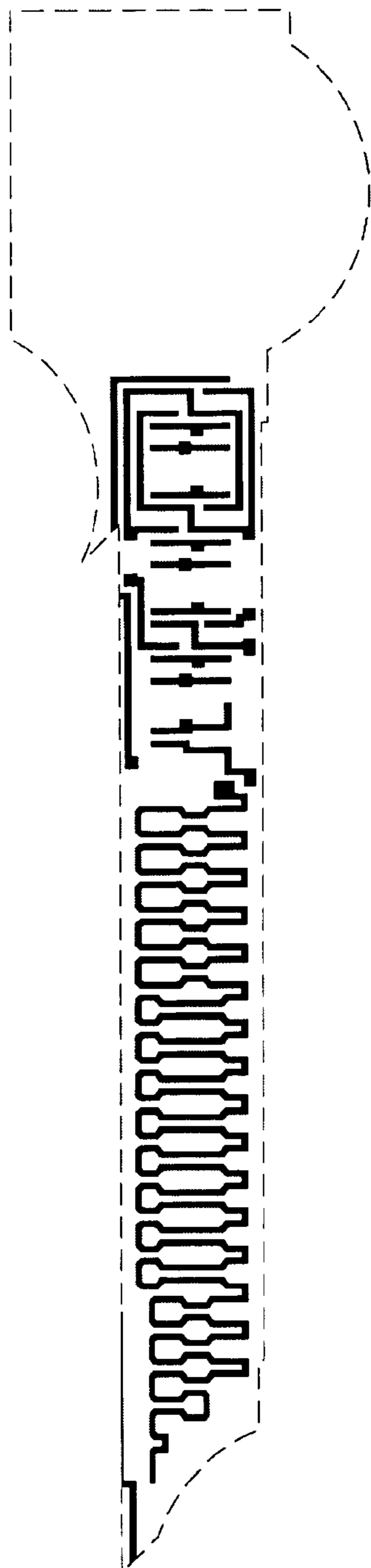
Poly mask
