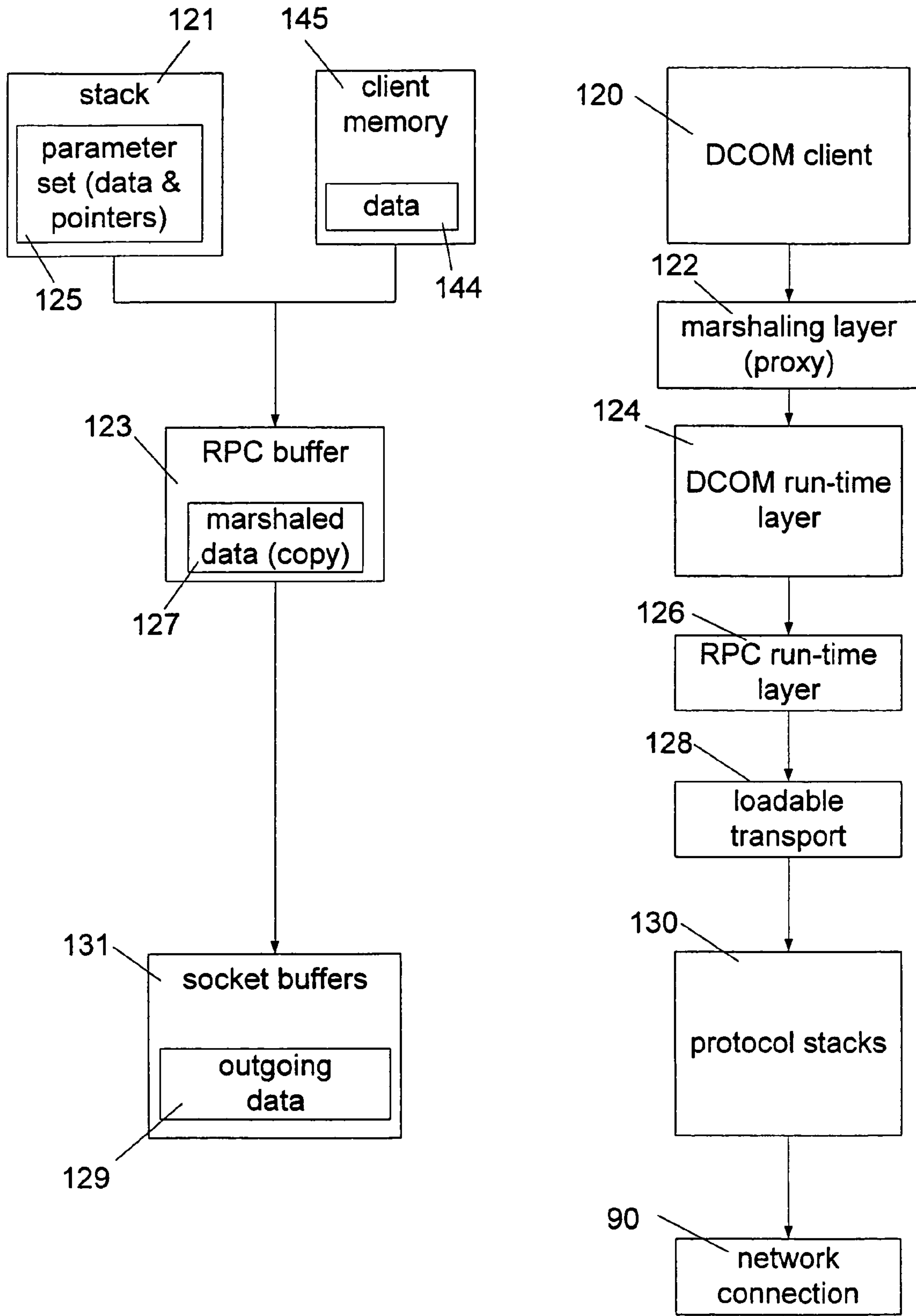
FIG. 3A
