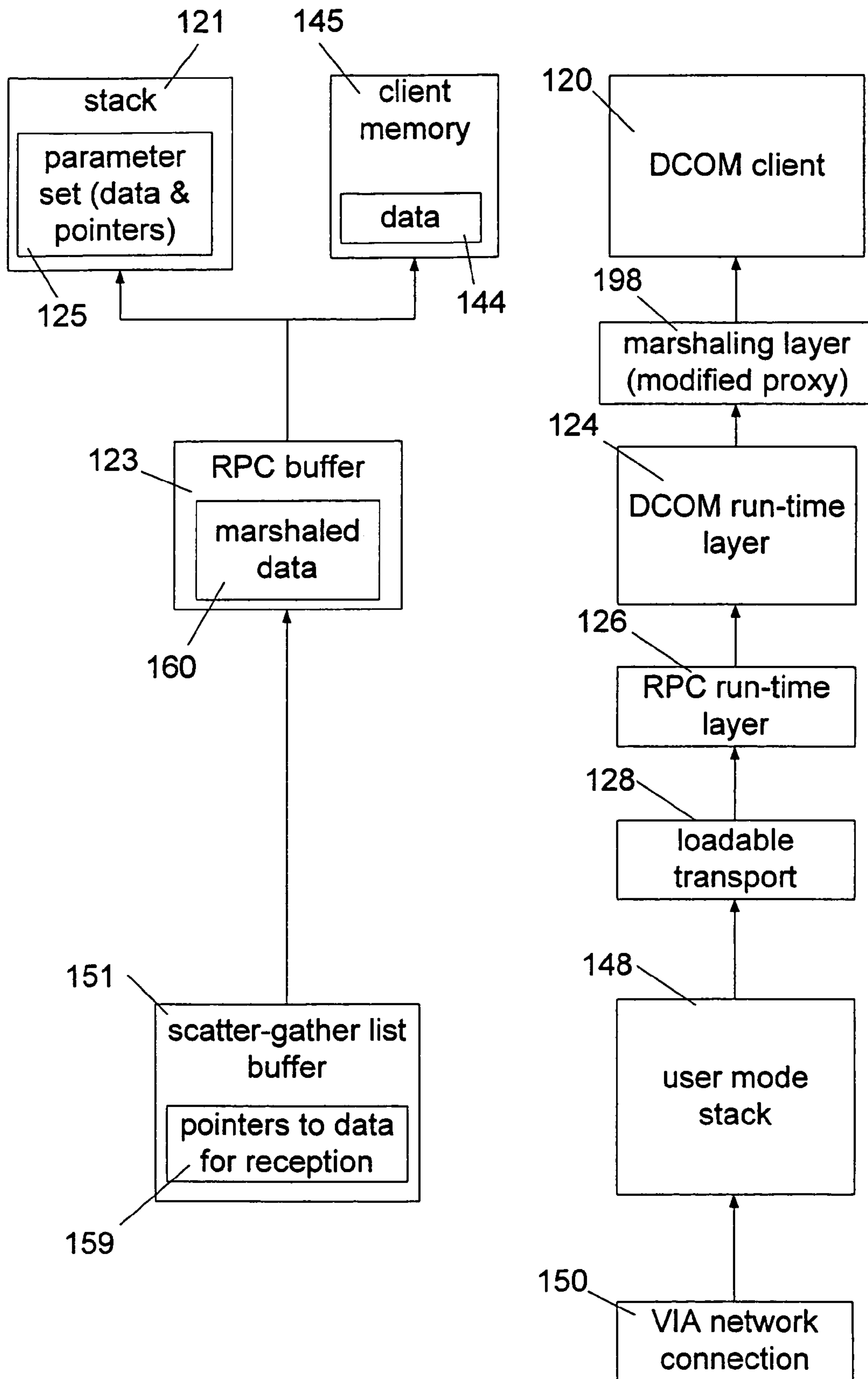
FIG. 5A
