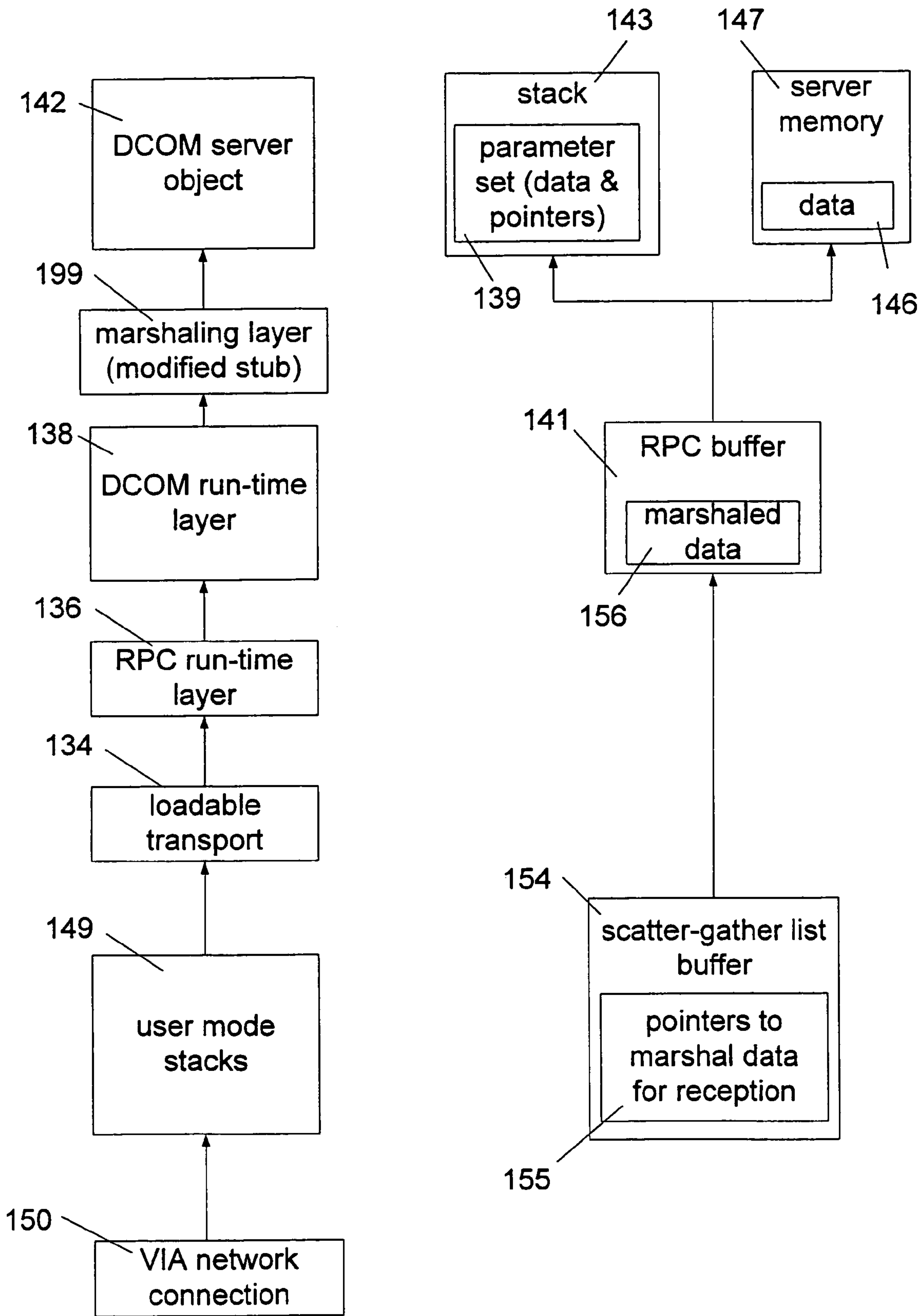
FIG. 4B
