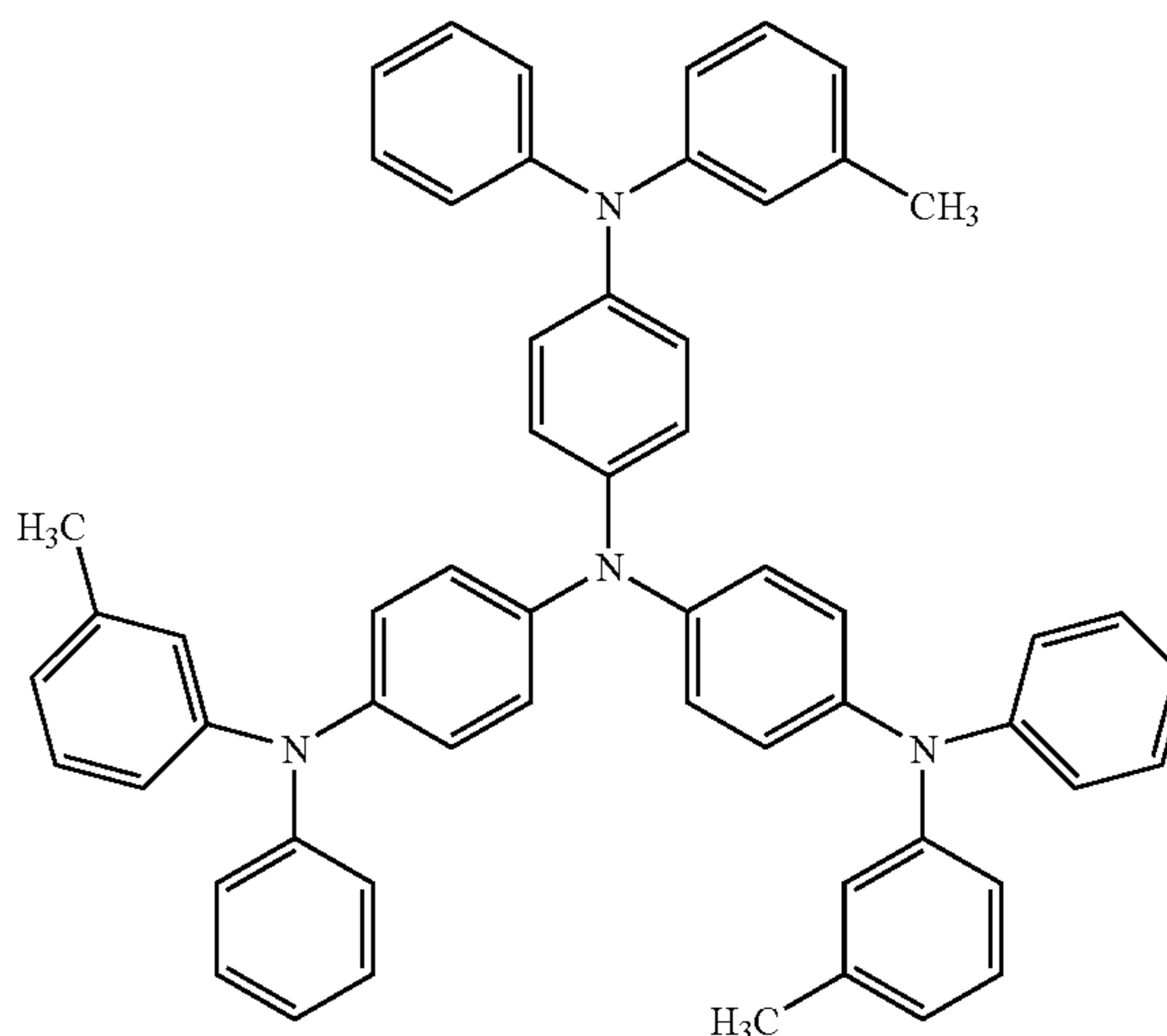
m-MTDATA
