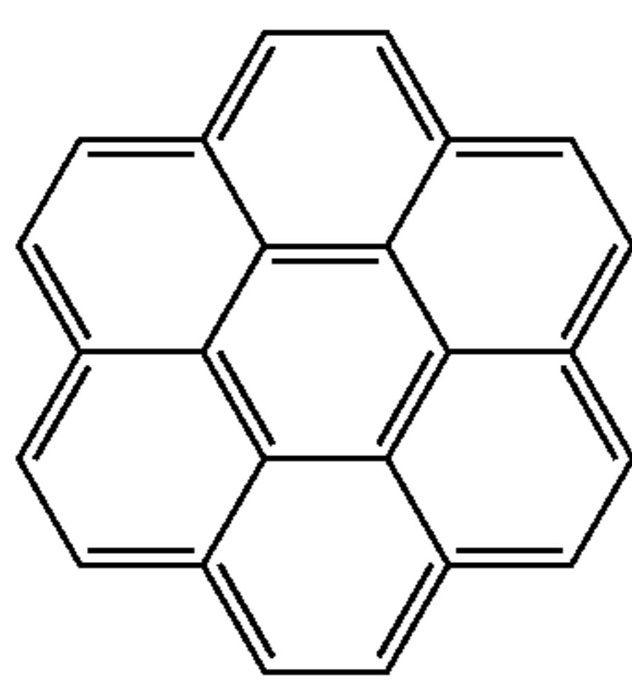
Coronene
