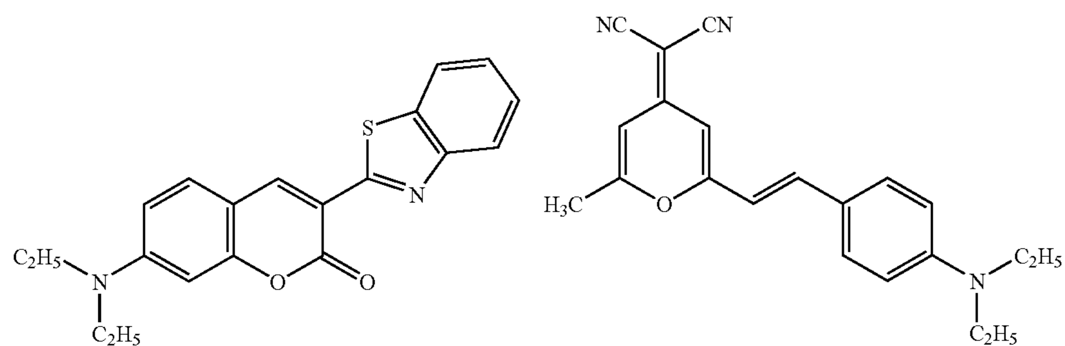
Coumarin 6
