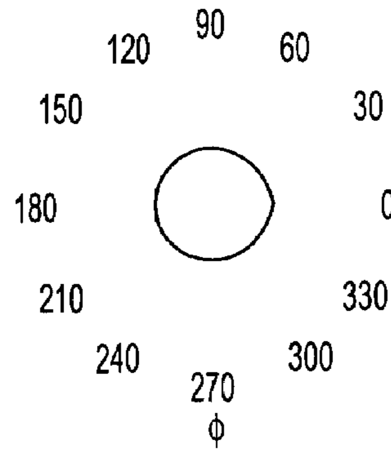
FIG. 2B m = 1 n = 1
