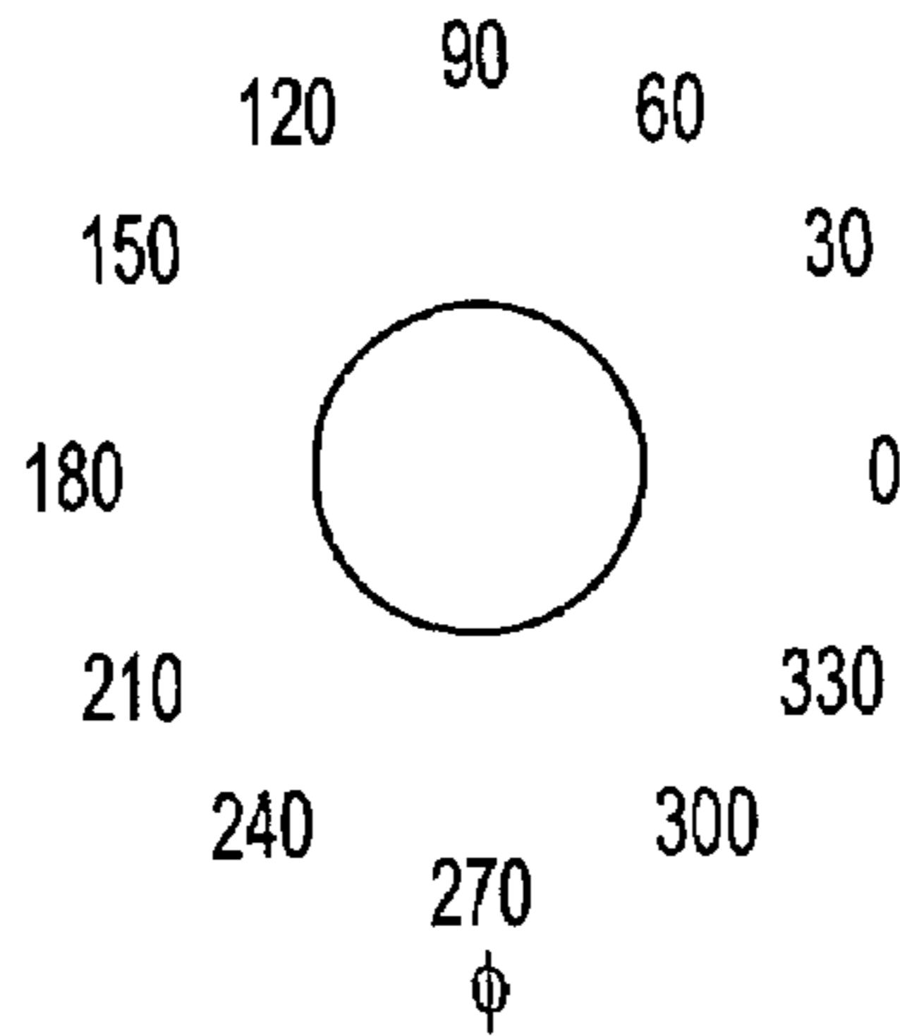
FIG. 2A m = 0 n = 1
