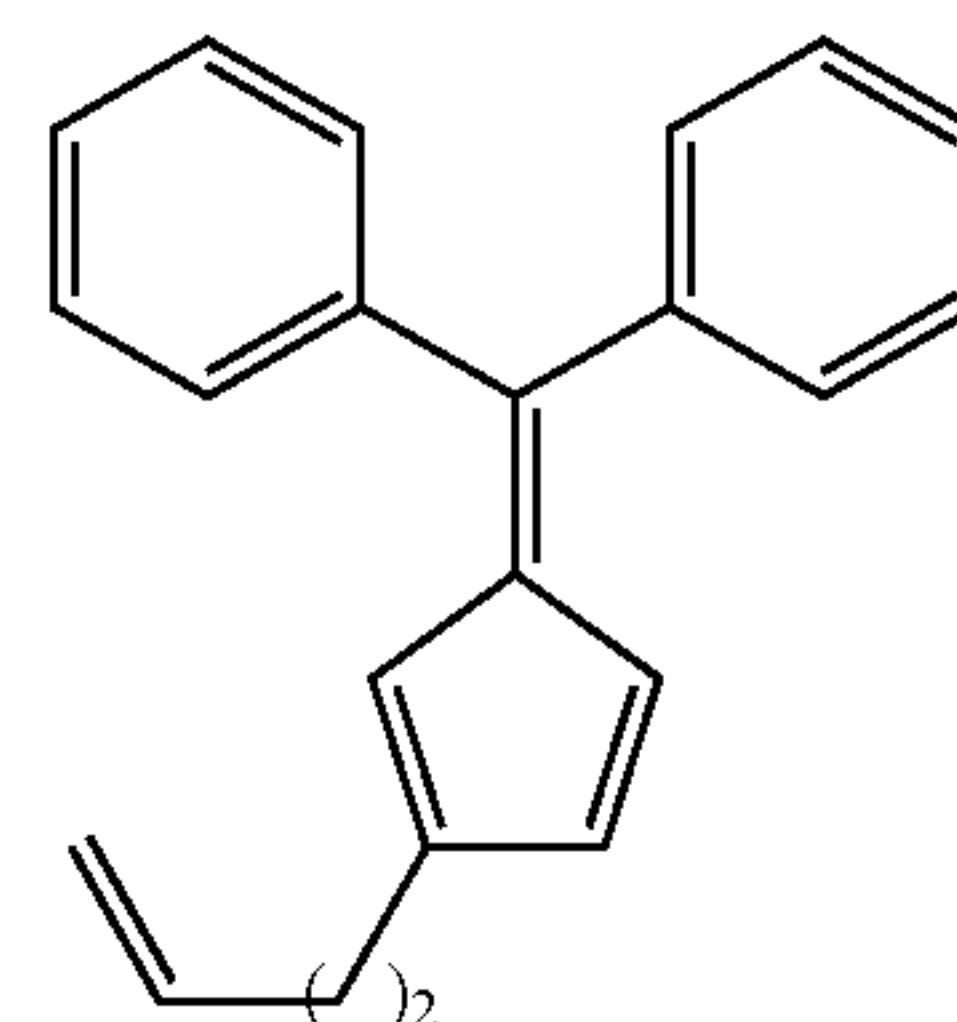
2-(but-3-enyl)-6,6-diphenylpentafulvene
