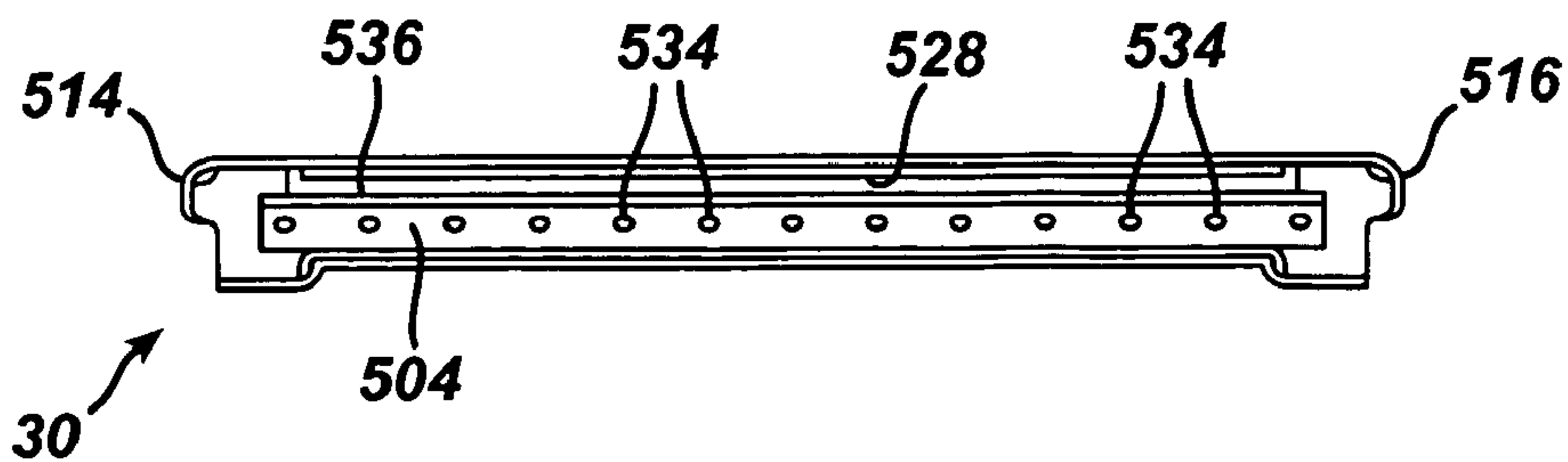
FIG. 7
