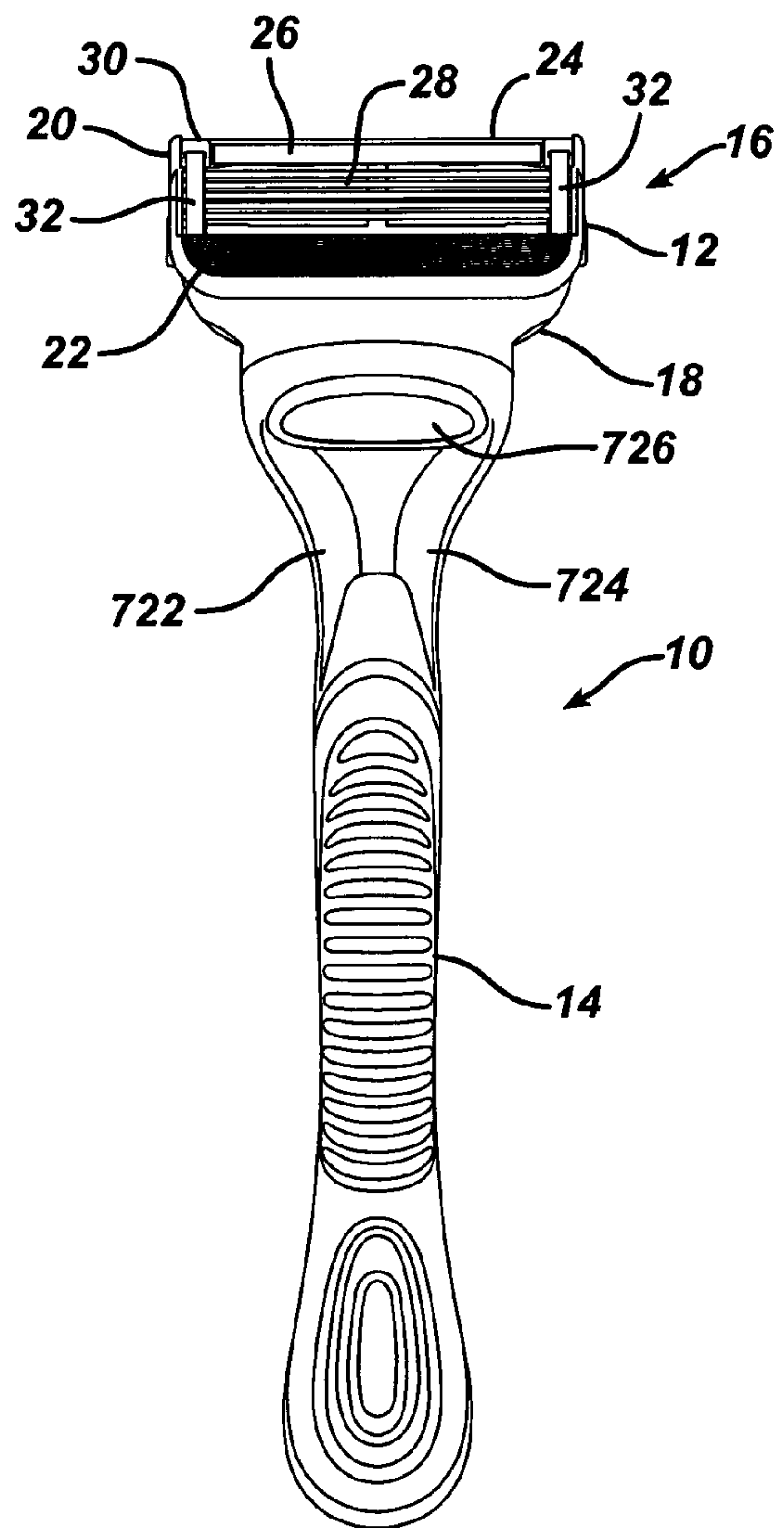
FIG. 15
