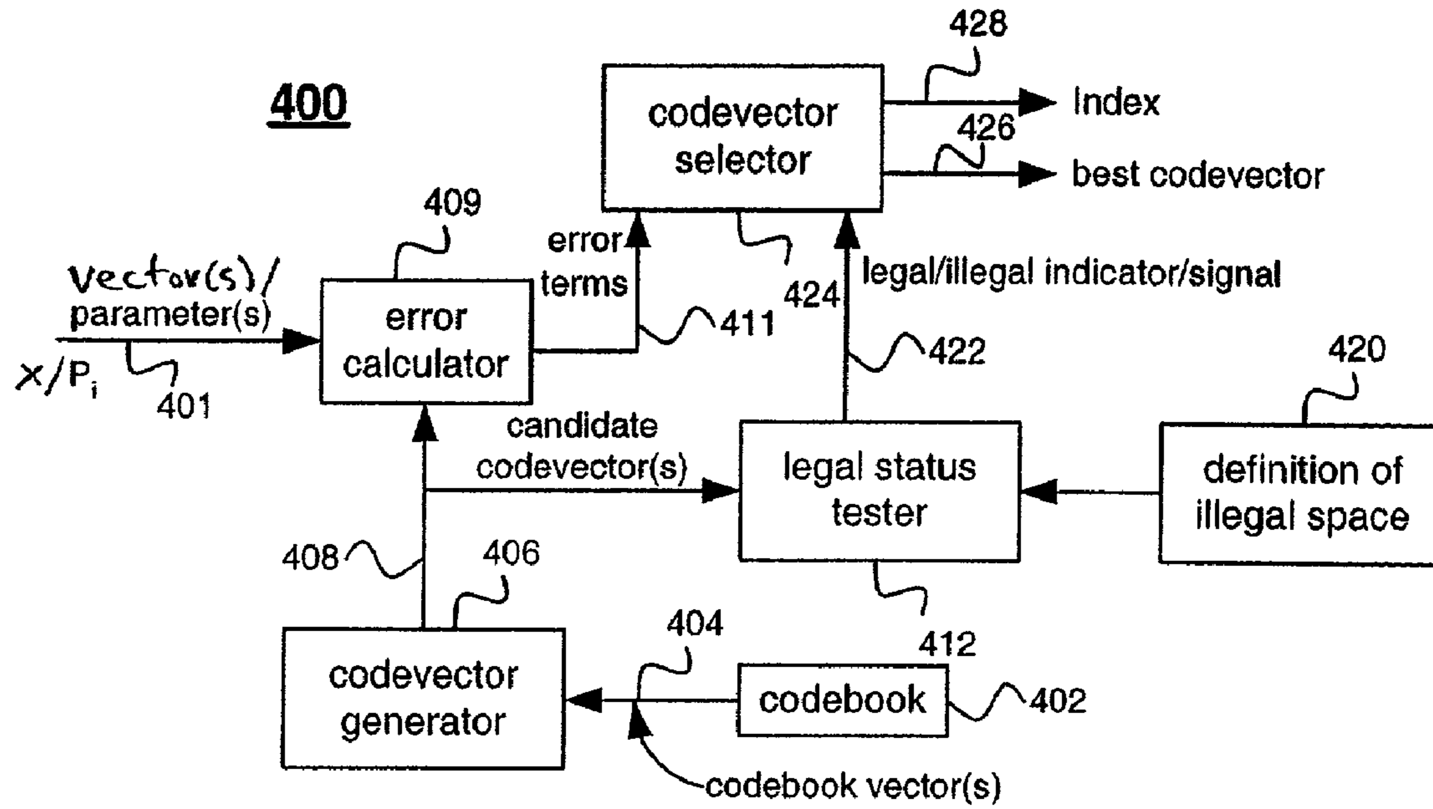
FIG. 4A: Quantizer (Encoder)
