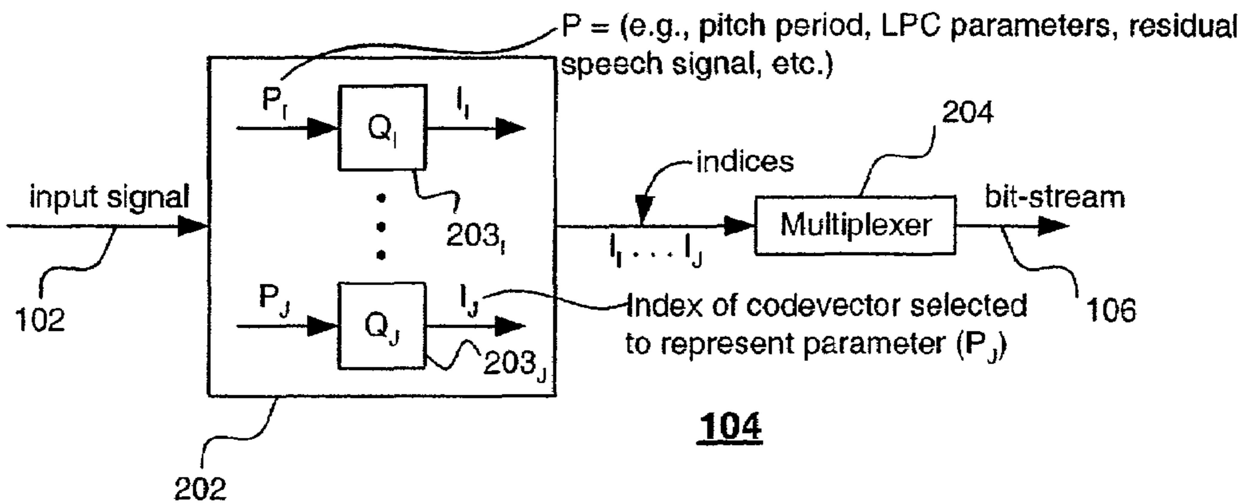
FIG. 2: Encoder
