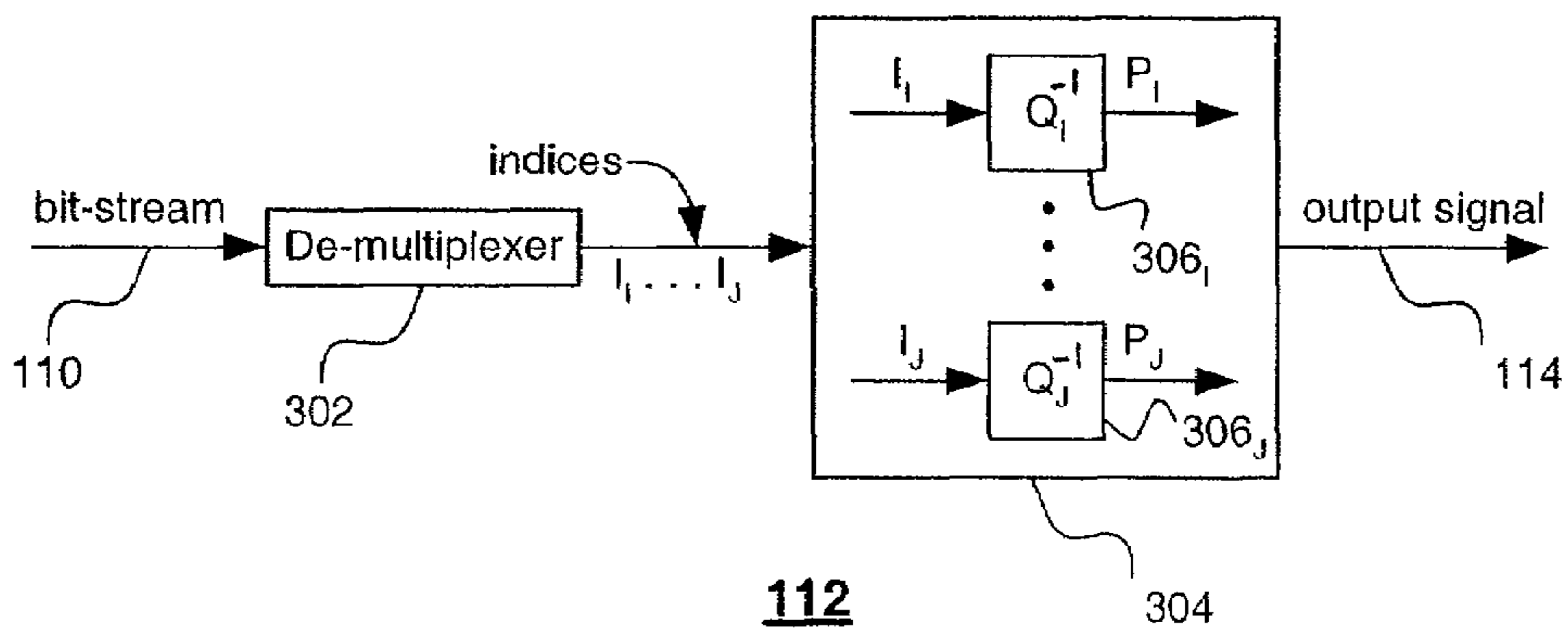
FIG. 3: Decoder
