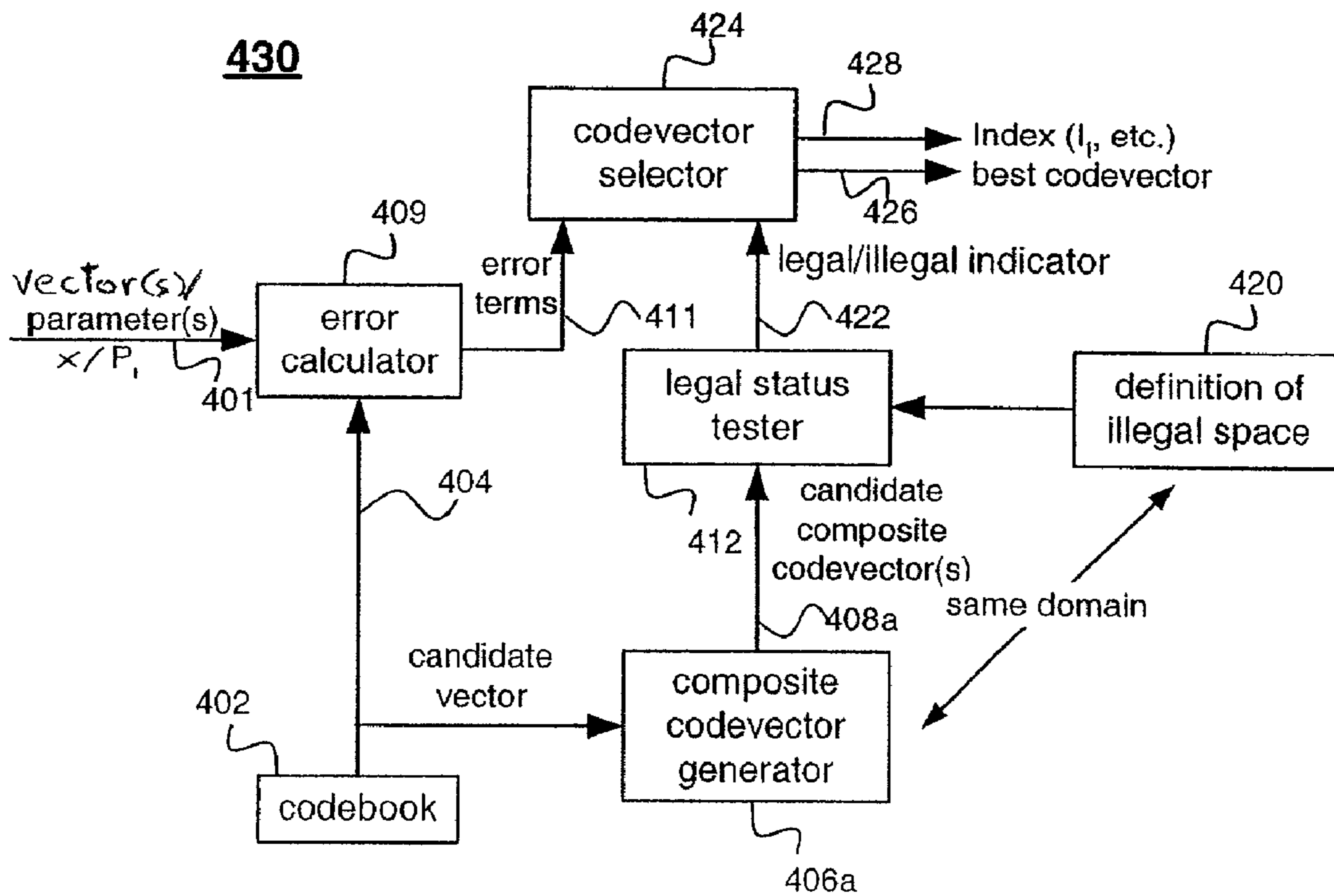
FIG. 4B: Quantizer (Encoder)
