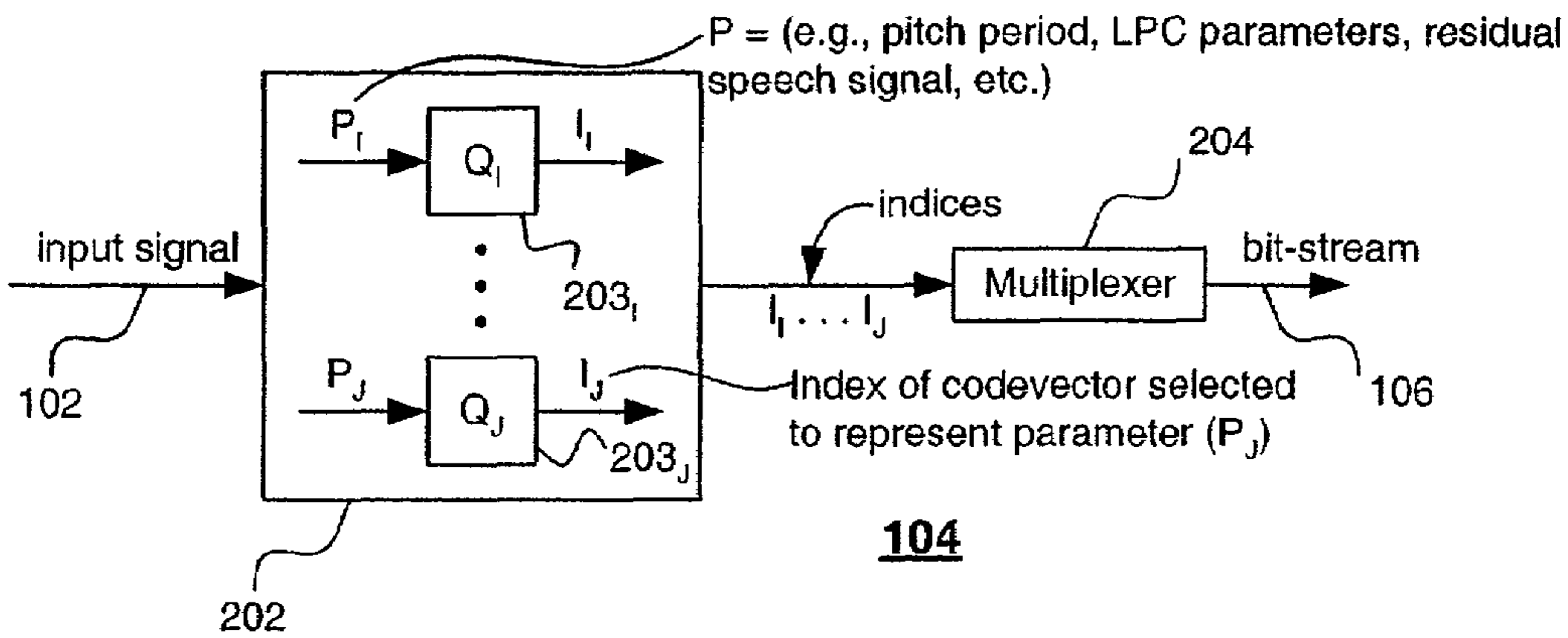
FIG. 2: Encoder
