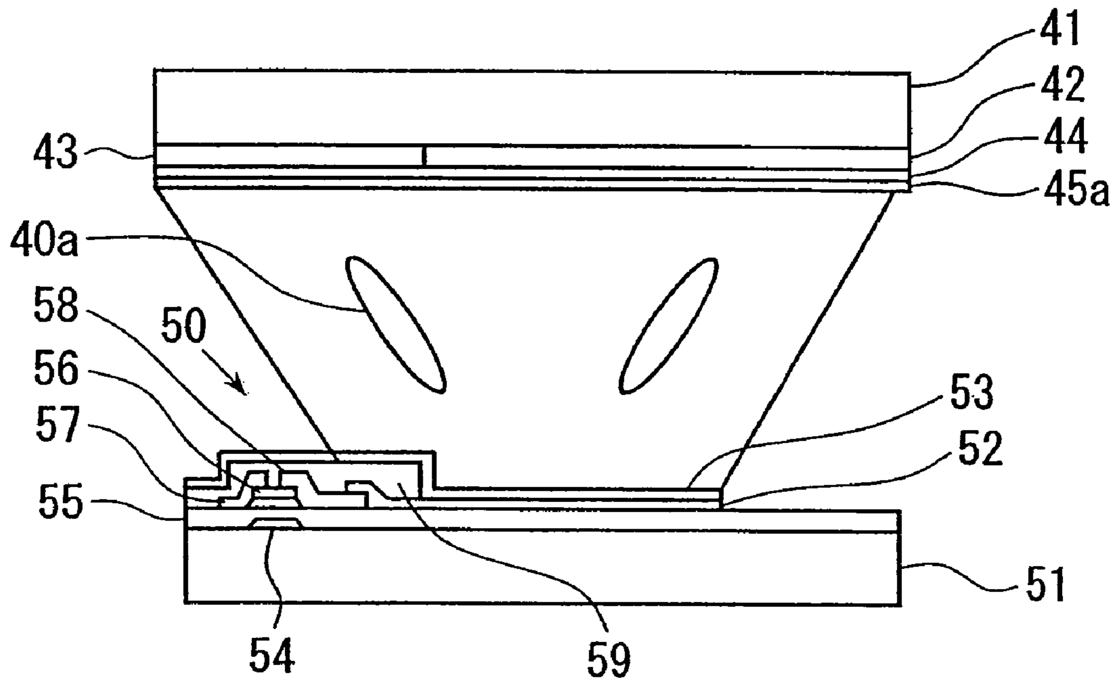
FIG. 25A
