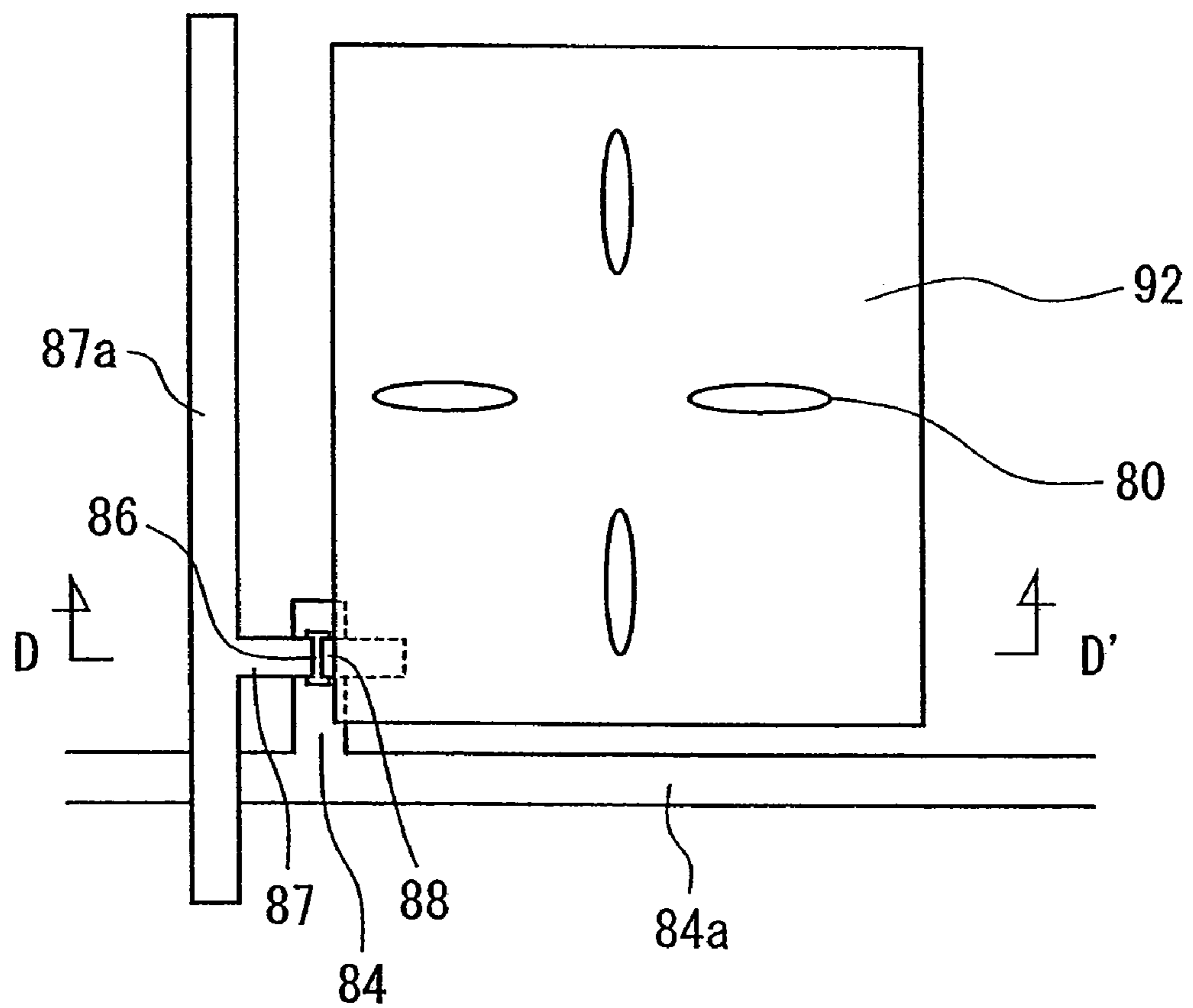
FIG. 27B
