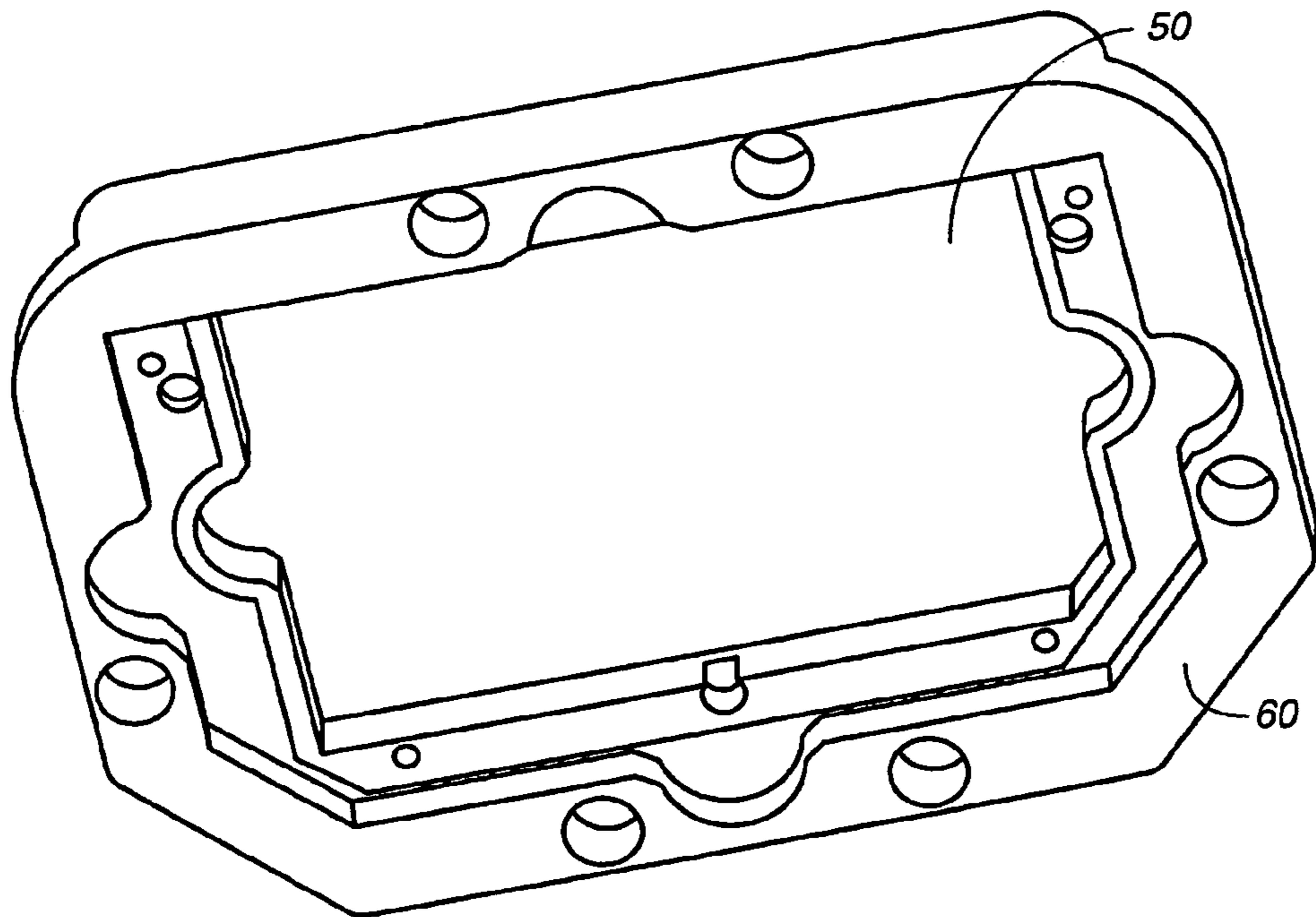
FIG. 7B
