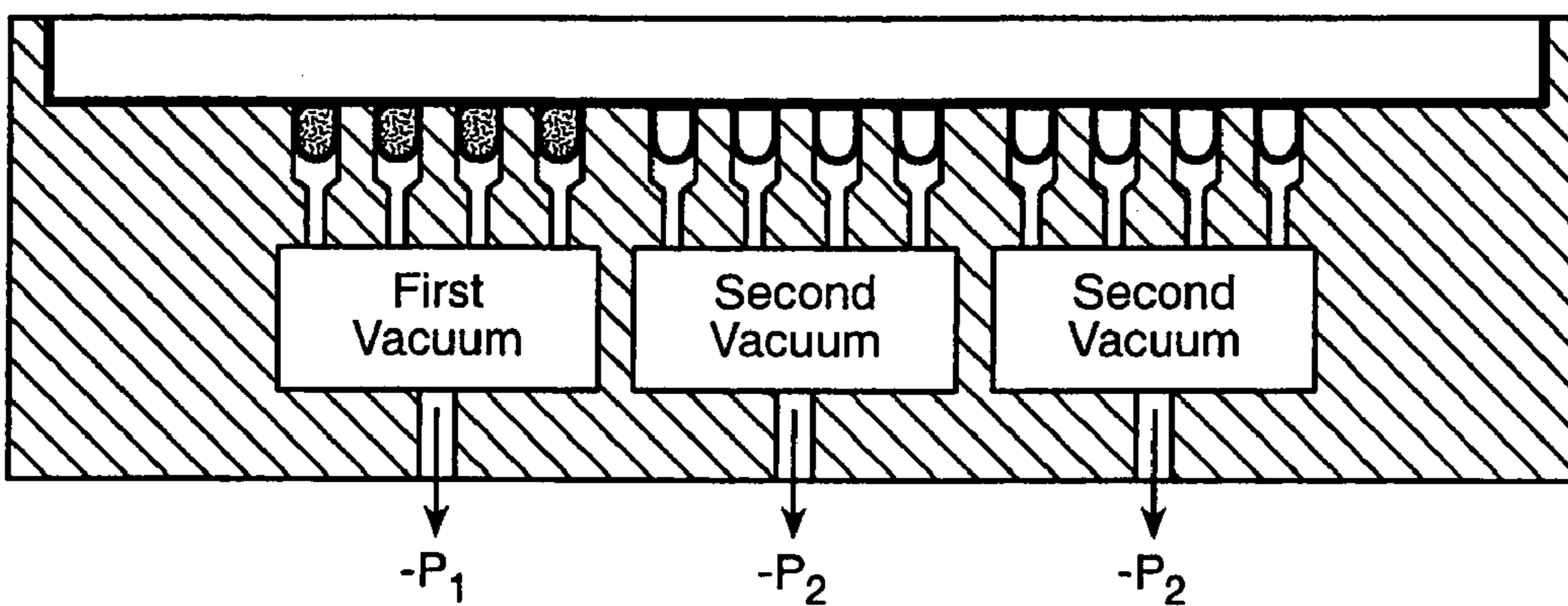
FIG. 10C
