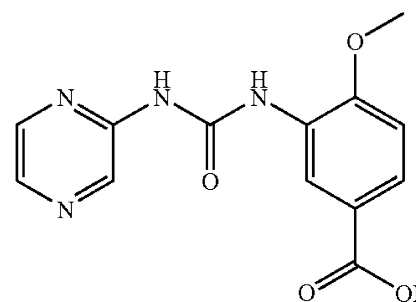
4-Methoxy-3-(3-pyrazin-2-yl-ureido)-benzoic acid
