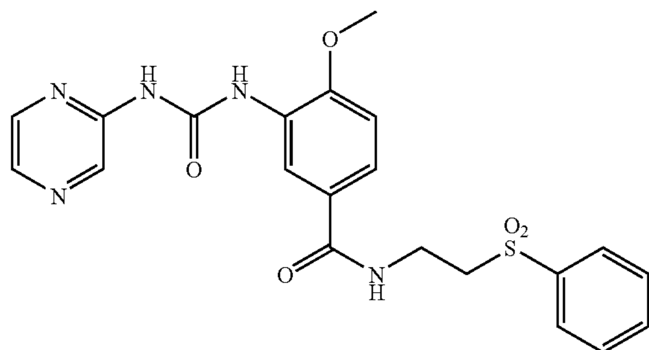
N-(2-Benzenesulfonyl-ethyl)-4-methoxy-3-(3-pyrazin-2-yl-ureido)-benzamide
