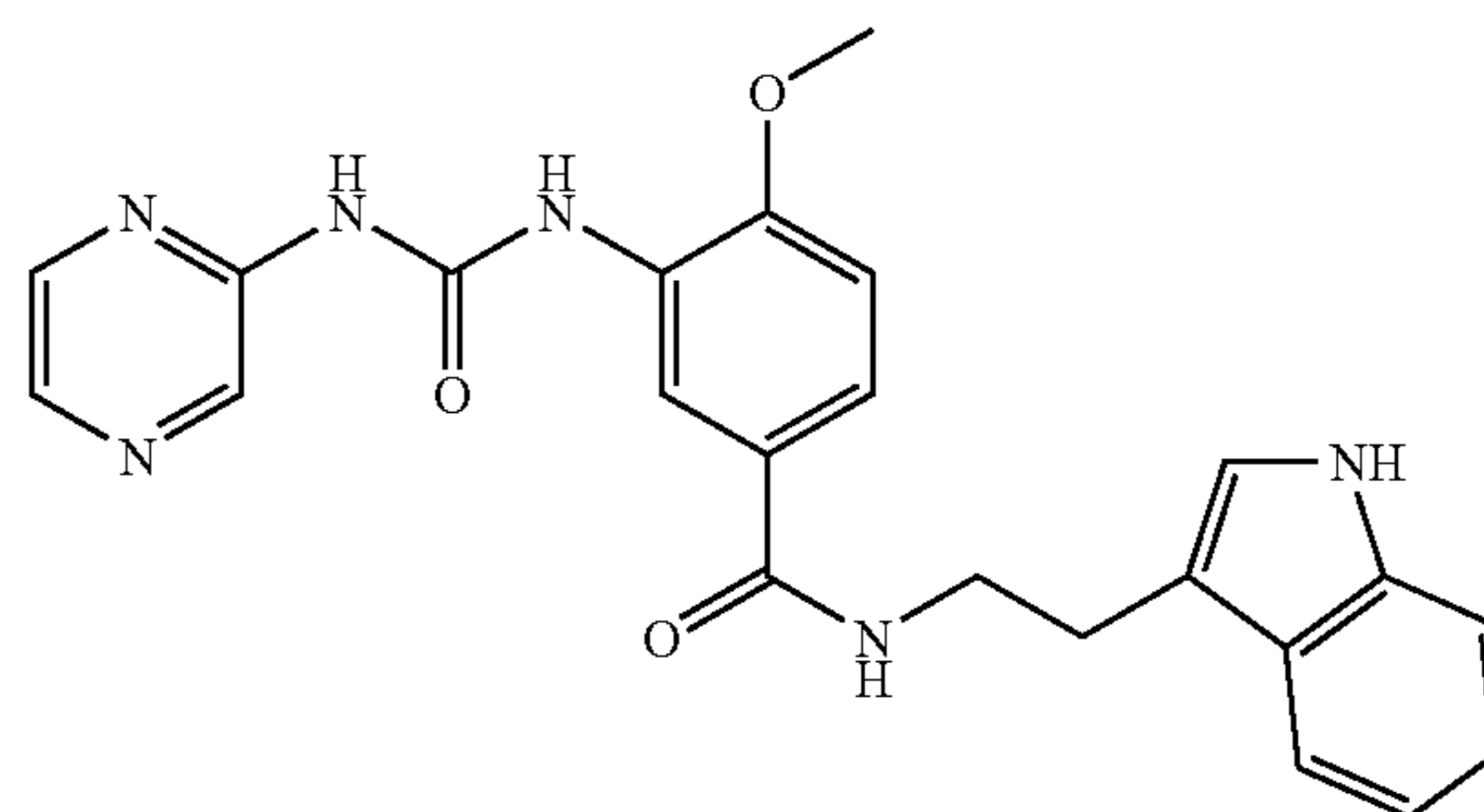
N-[2-(1H-Indol-3-yl)-ethyl]-4-methoxy-3-(3-pyrazin-2-yl-ureido)-benzamide
