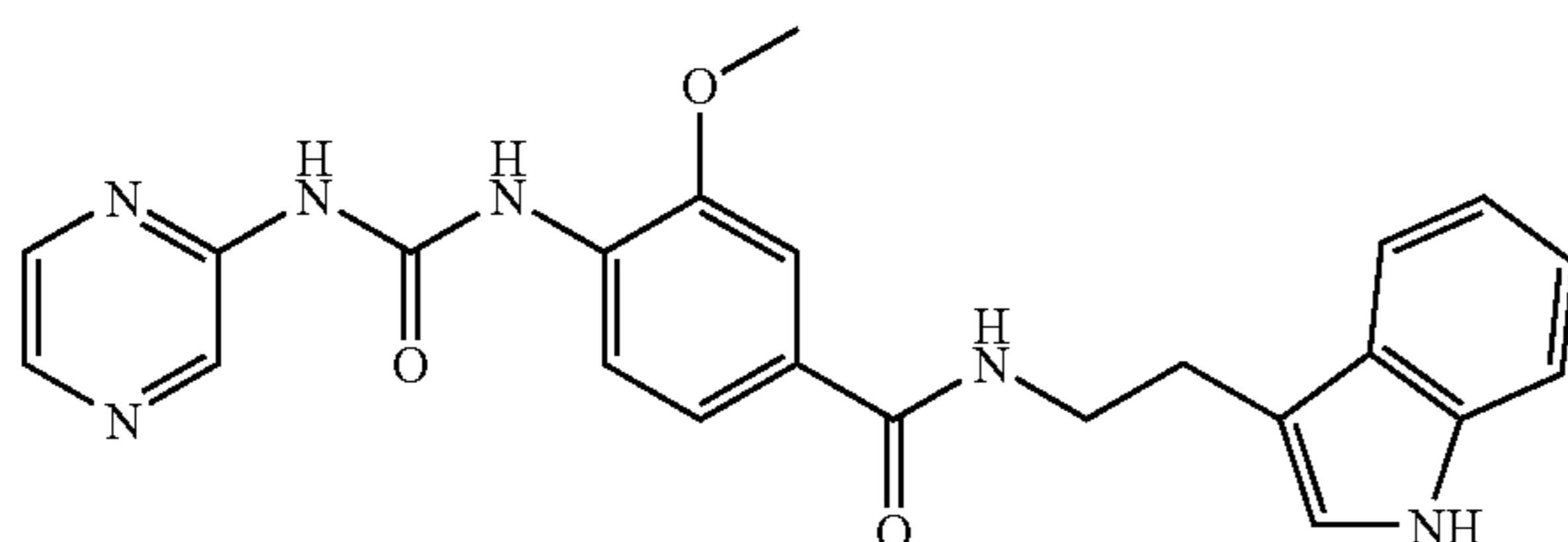
N-[2-(1H-Indol-3-yl)-ethyl]-3-methoxy-4-(3-pyrazin-2-yl-ureido)-benzamide
