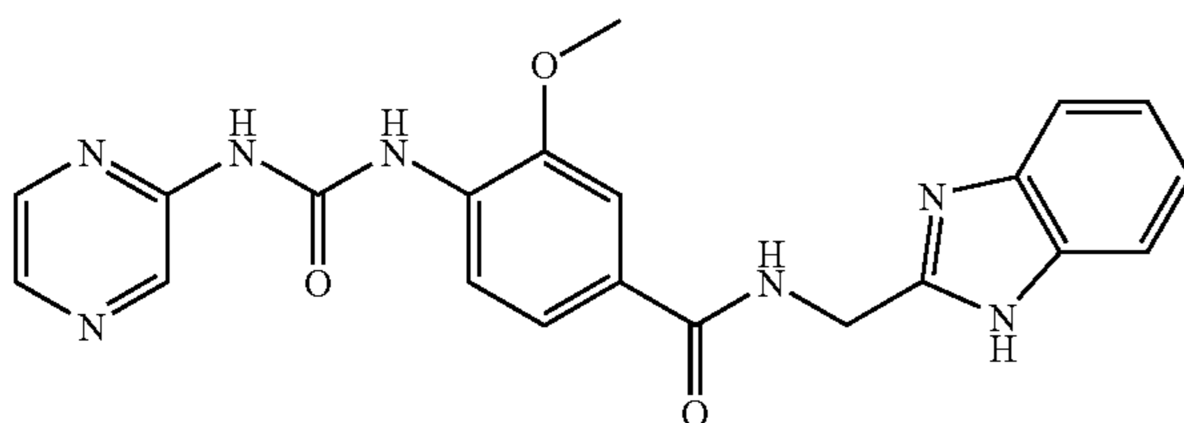
N-(1H-Benzoimidazol-2-ylmethyl)-3-methoxy-4-(3-pyrazin-2-yl-ureido)-benzamide
