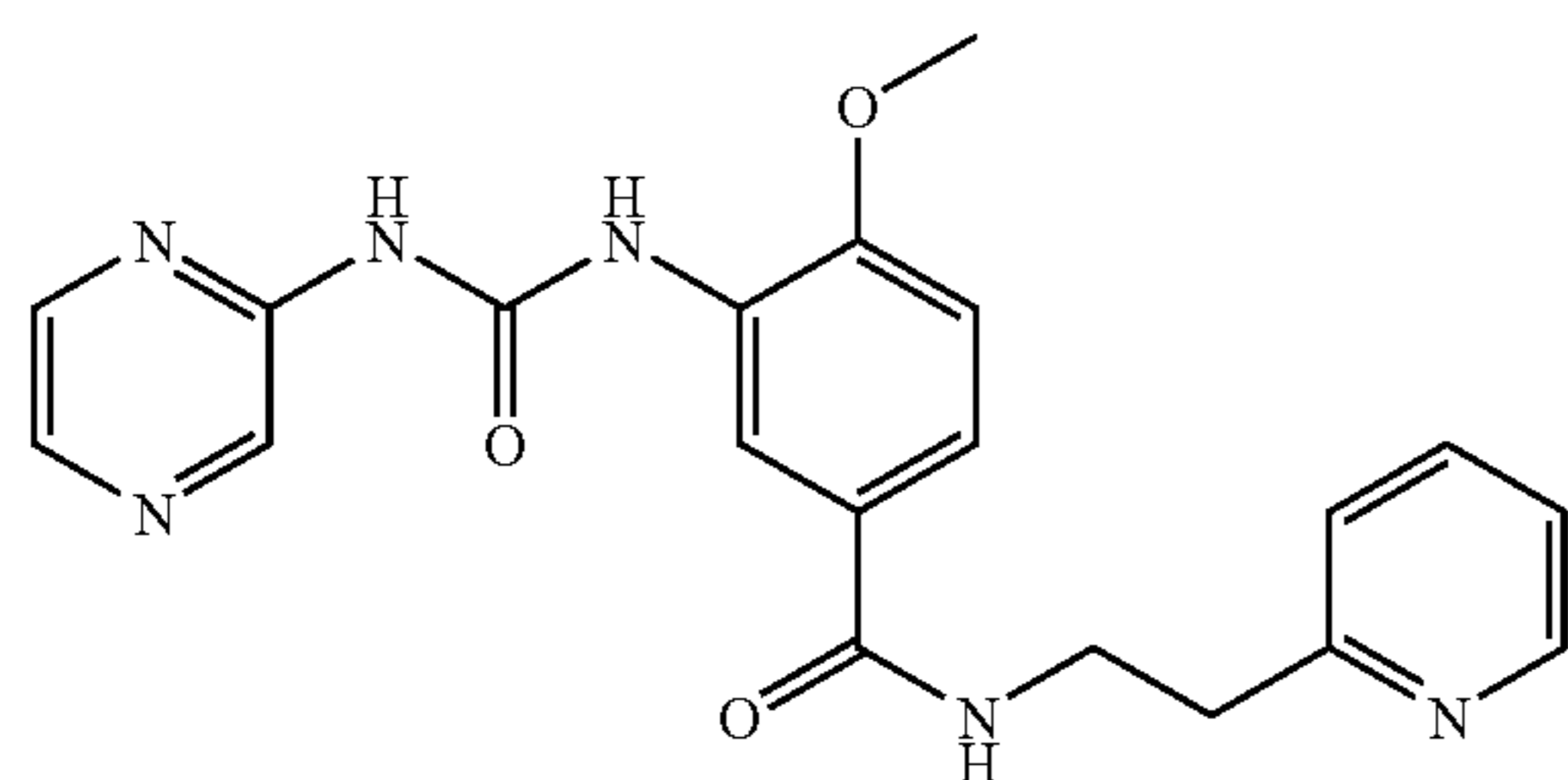
4-Methoxy-3-(3-pyrazin-2-yl-ureido)-N-(2-pyridin-2-yl-ethyl)-benzamide
