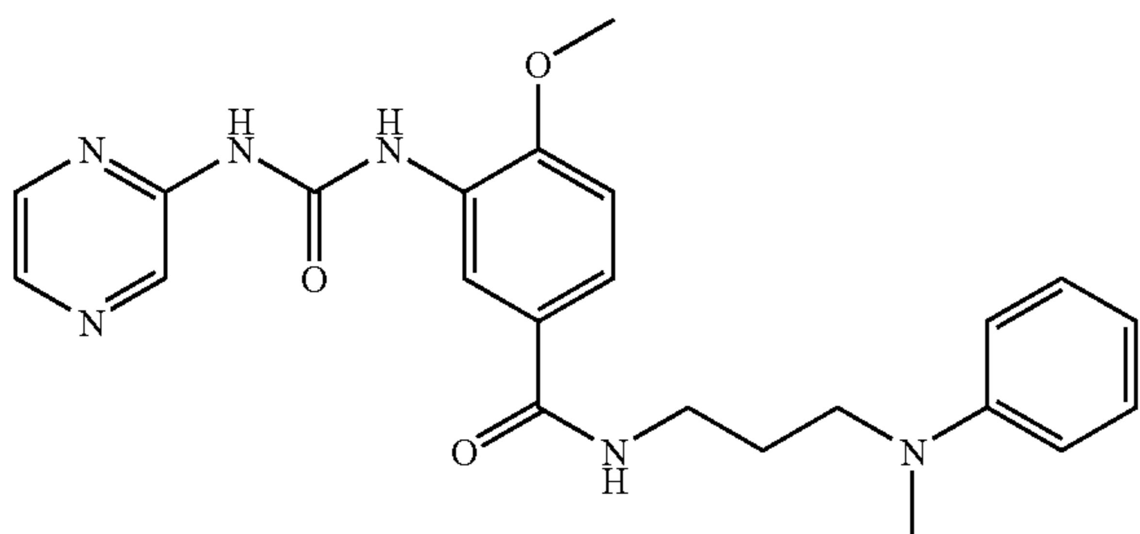
4-Methoxy-N-[3-(methyl-phenyl-amino)-propyl]-3-(3-pyrazin-2-yl-ureido)-benzamide
