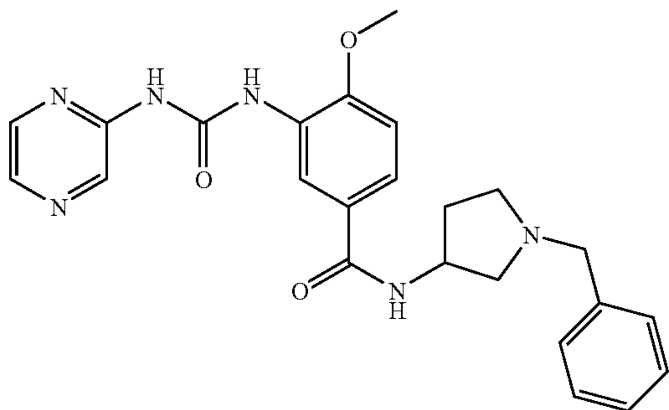
N-(1-Benzyl-pyrrolidin-3-yl)-4-methoxy-3-(3-pyrazin-2-yl-ureido)-benzamide
