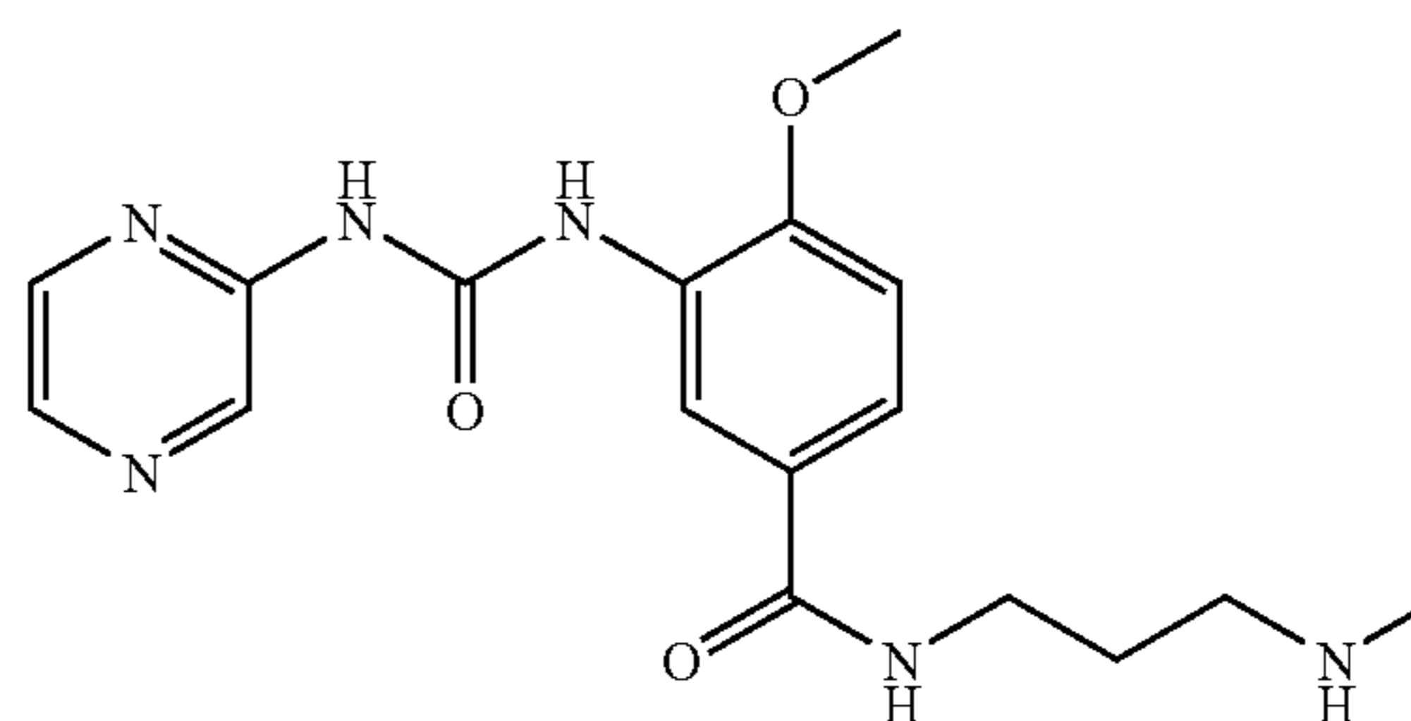
4-Methoxy-N-(3-methylamino-propyl)-3-(3-pyrazin-2-yl-ureido)-benzamide
