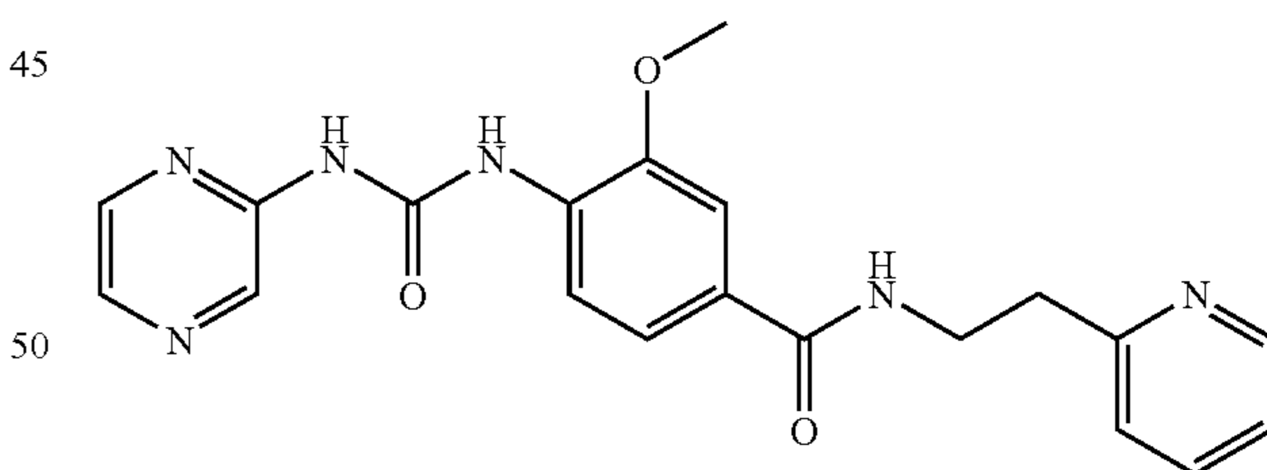
3-Methoxy-4-(3-pyrazin-2-yl-ureido)-N-(2-pyridin-2-yl-ethyl)-benzamide
