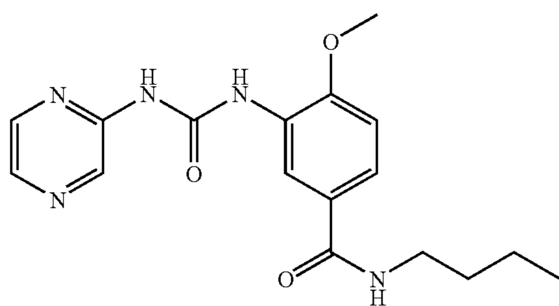
N-Butyl-4-methoxy-3-(3-pyrazin-2-yl-ureido)-benzamide
