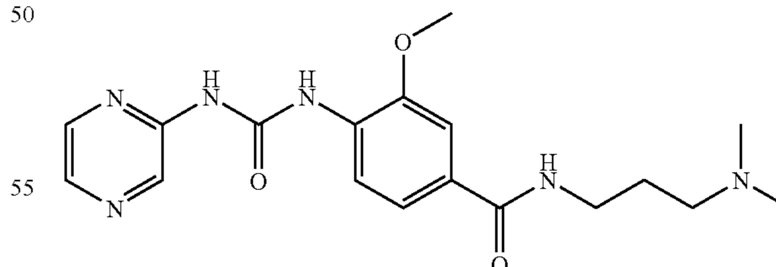
N-(3-Dimethylamino-propyl)-3-methoxy-4-(3-pyrazin-2-yl-ureido)-benzamide
