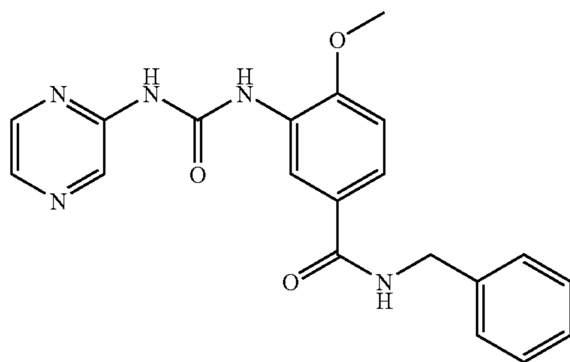
N-Benzyl-4-methoxy-3-(3-pyrazin-2-yl-ureido)-benzamide
