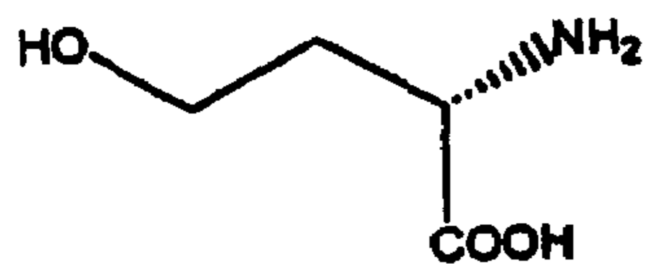
L-homoserine
