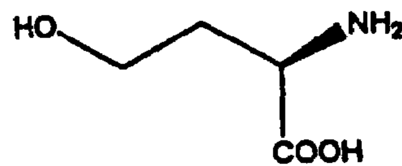
D-homoserine
