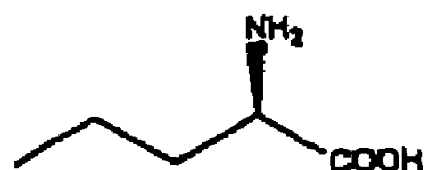
D-norvaline
