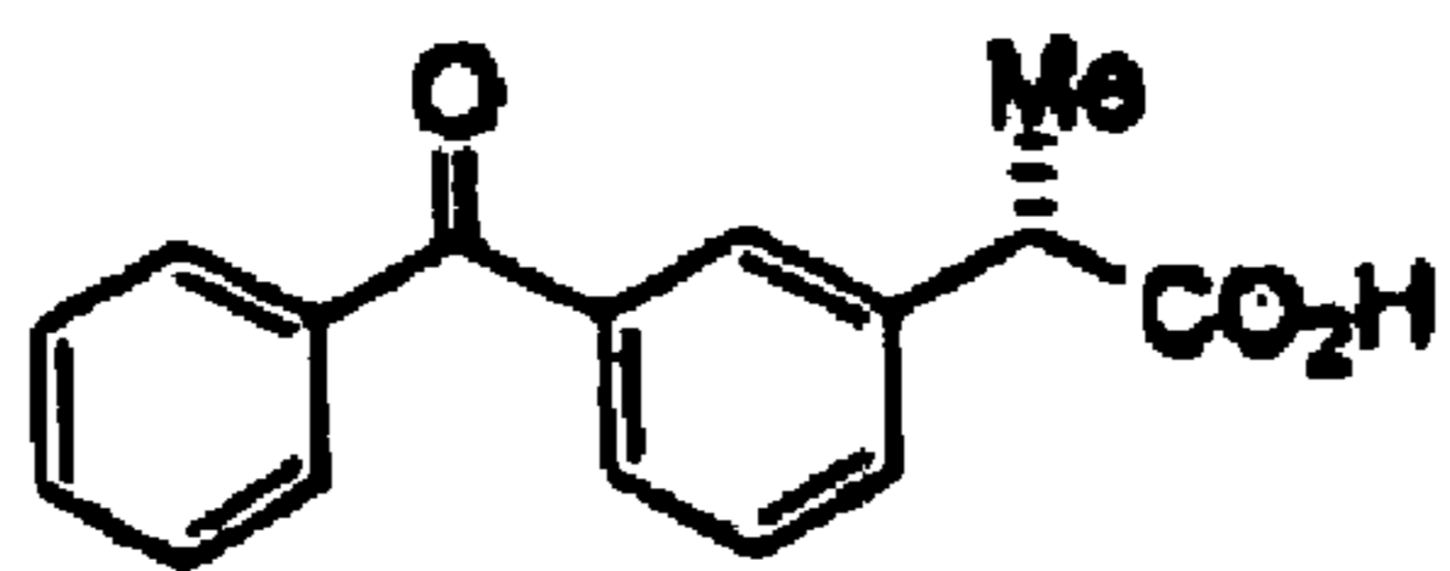
Dexketoprofen
