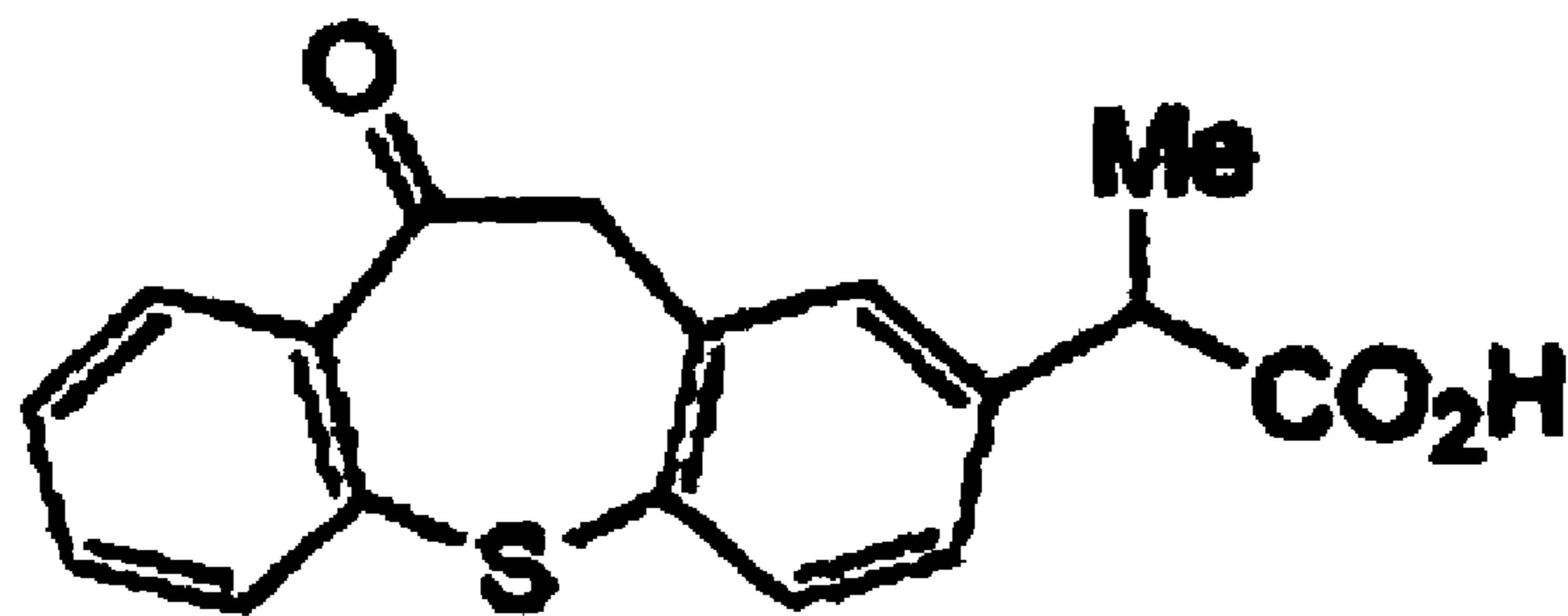
Zaltoprofen
