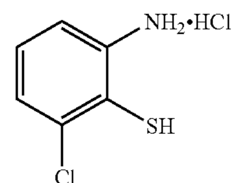
2-Amino-6-chlorobenzenethiol hydrochloride (205)
