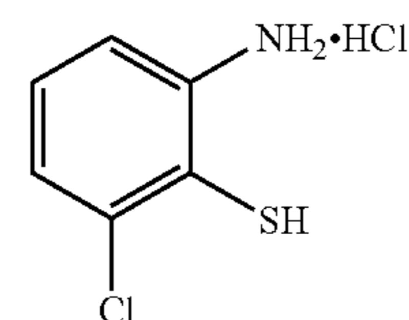
2-Amino-6-chlorobenzenethiol hydrochloride (205)
