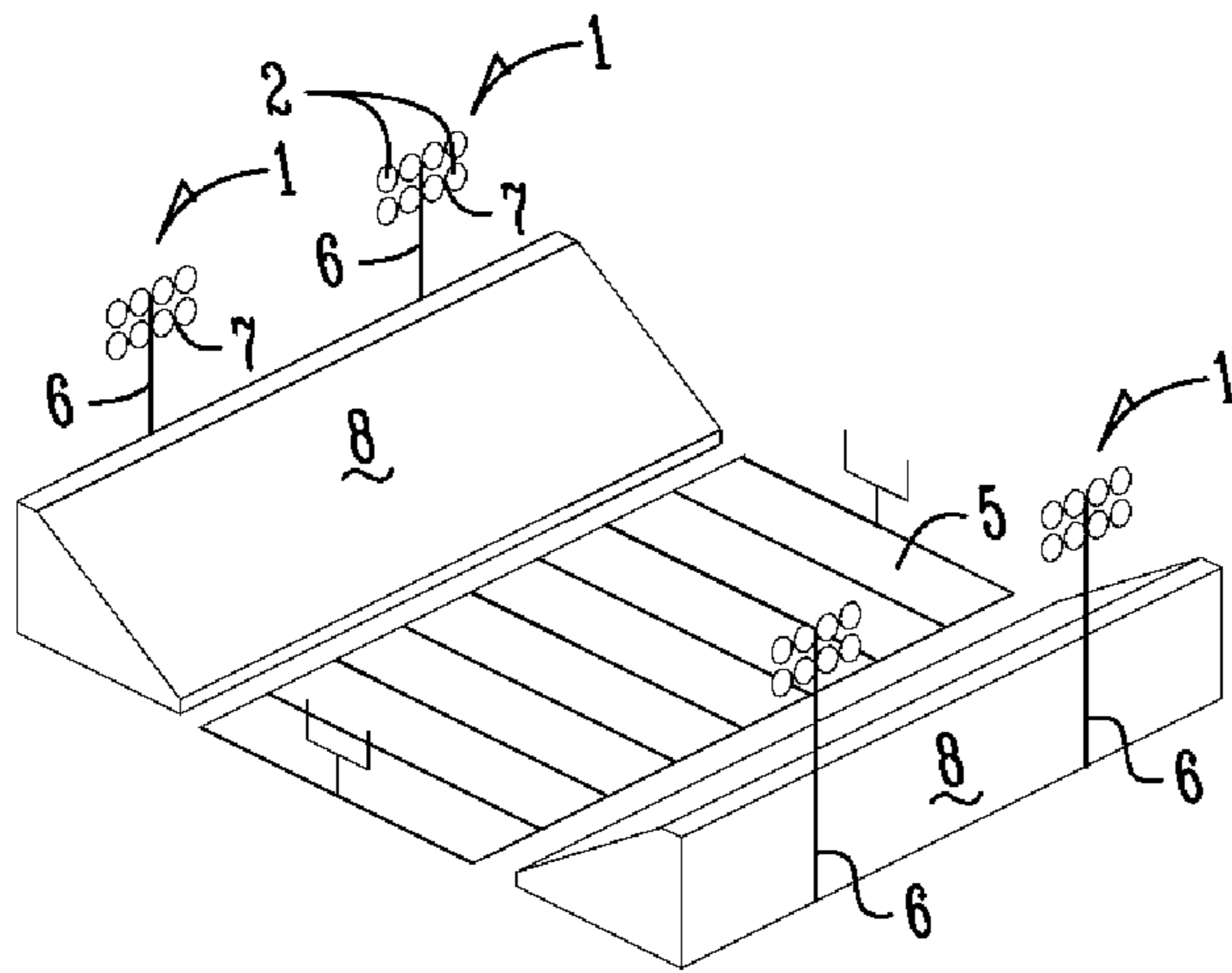
Fig. 1A
