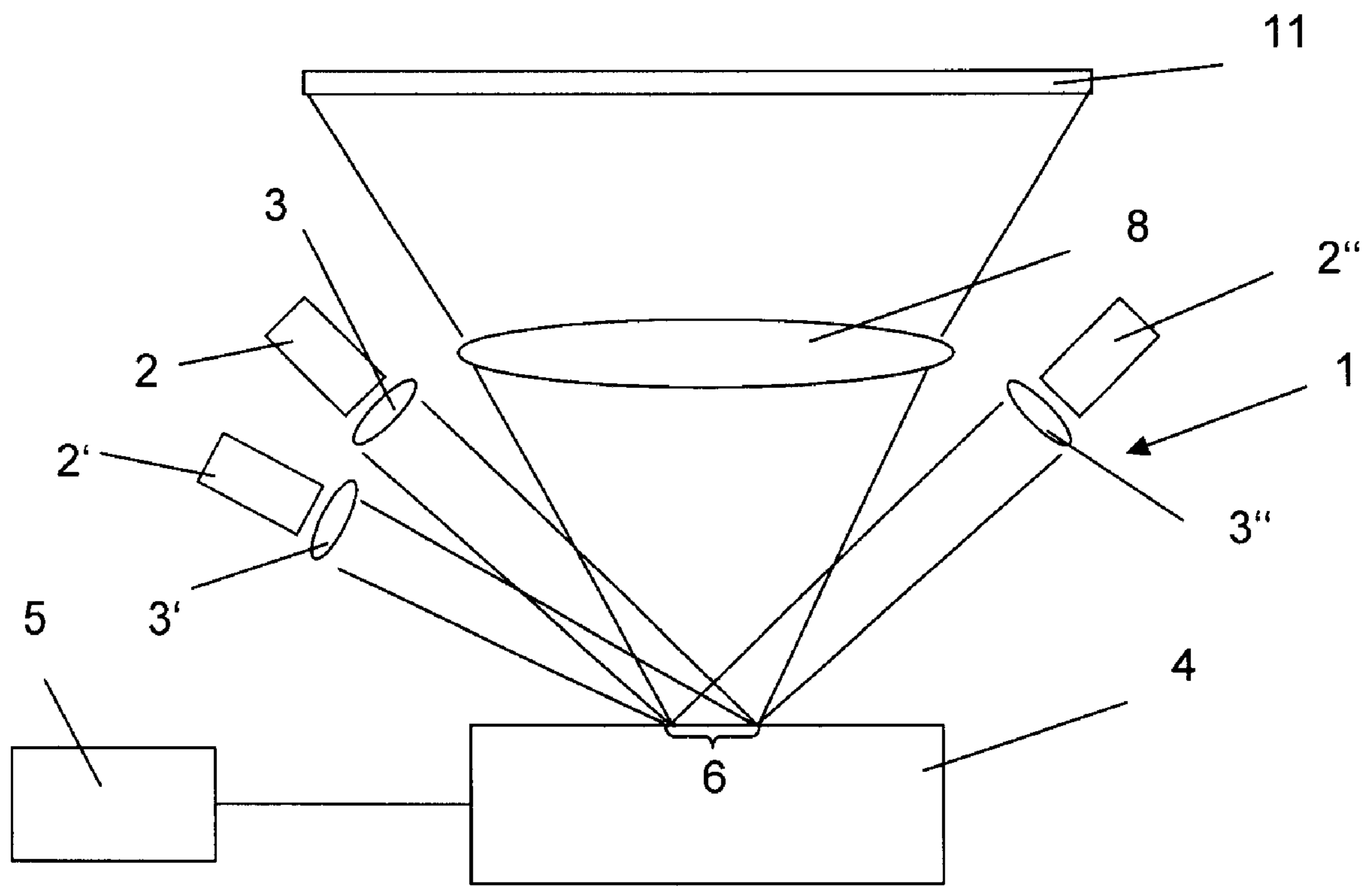
Fig. 3
