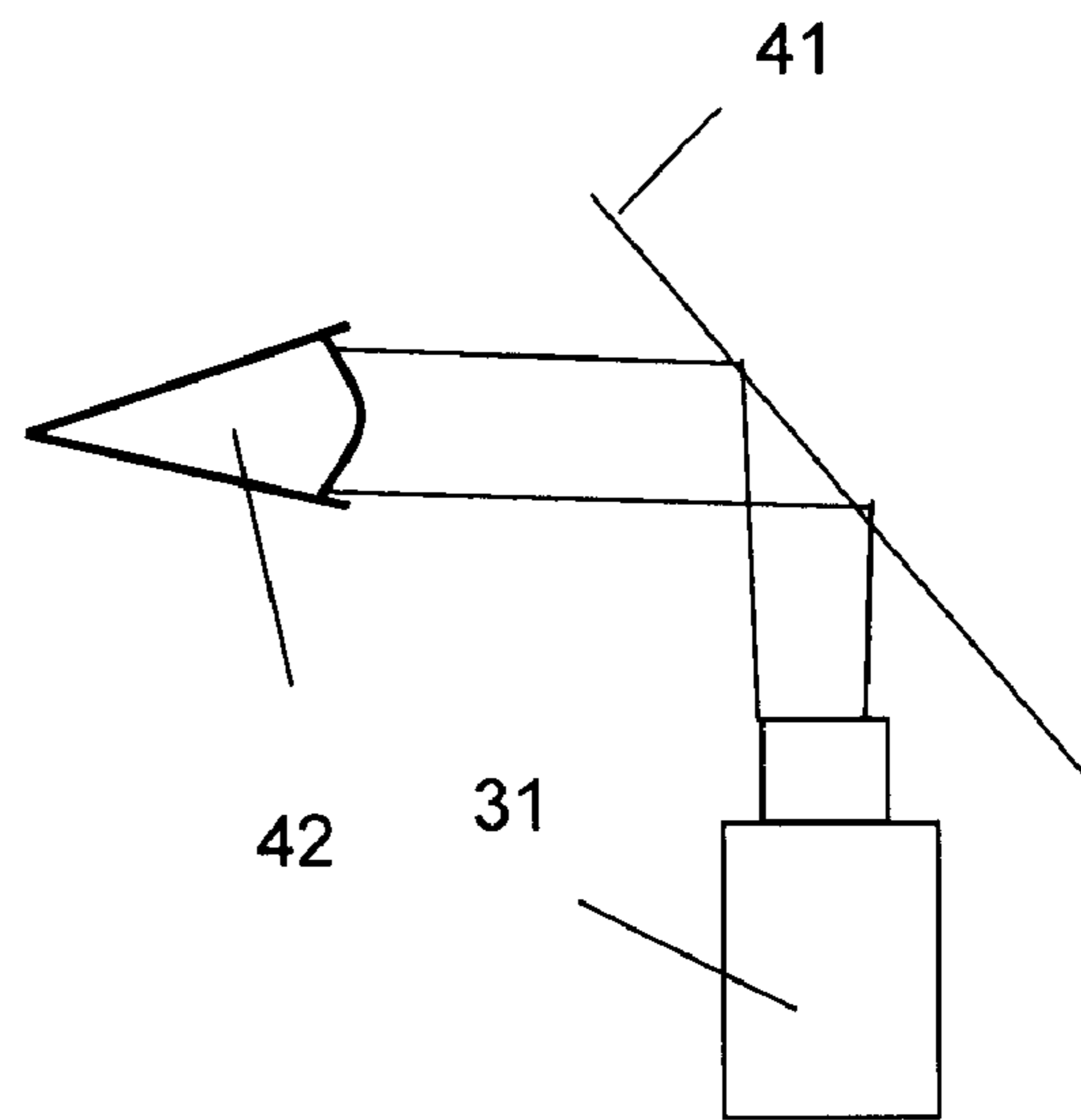
Fig. 9
