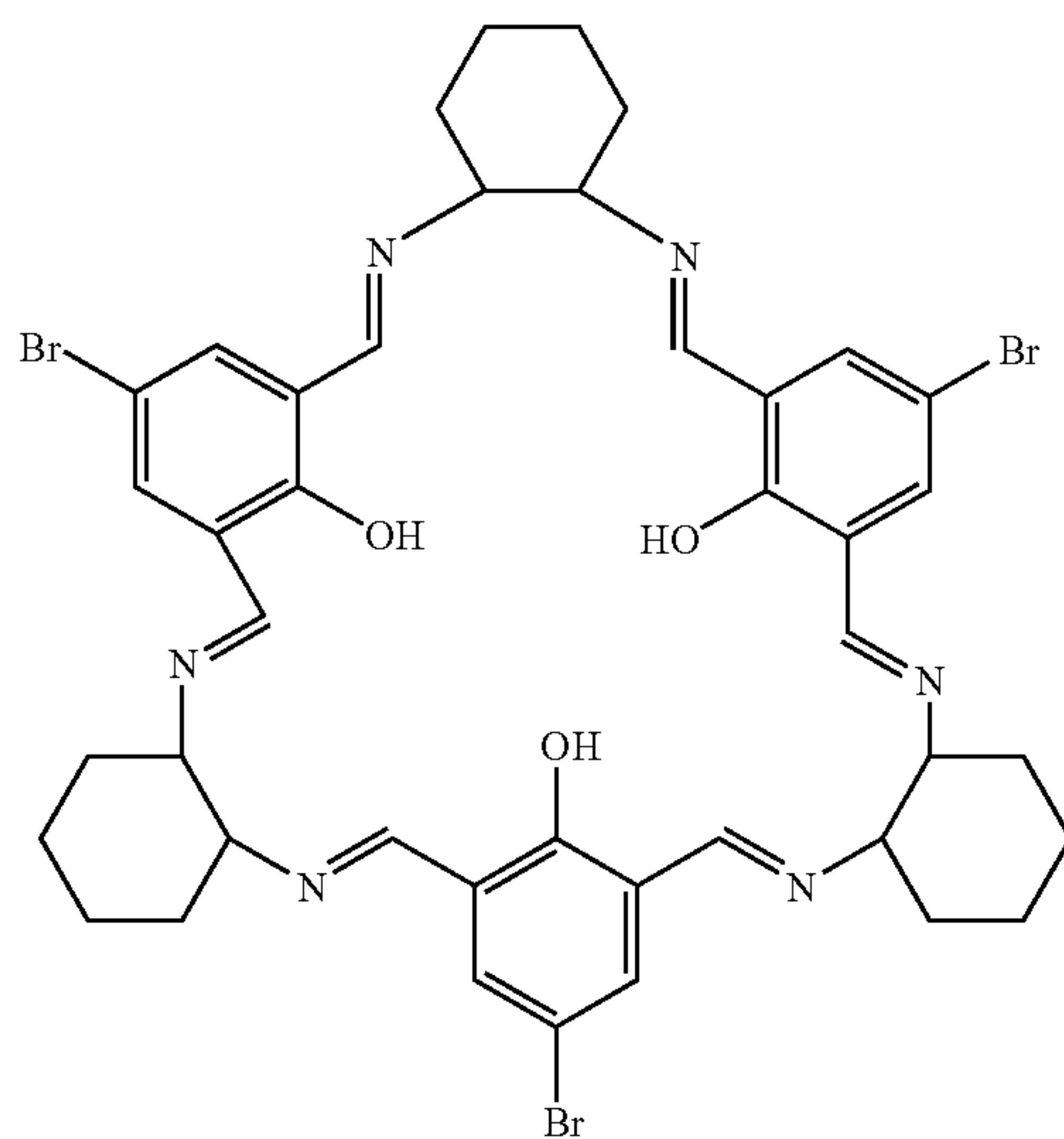
Hexamer 1a-Br
