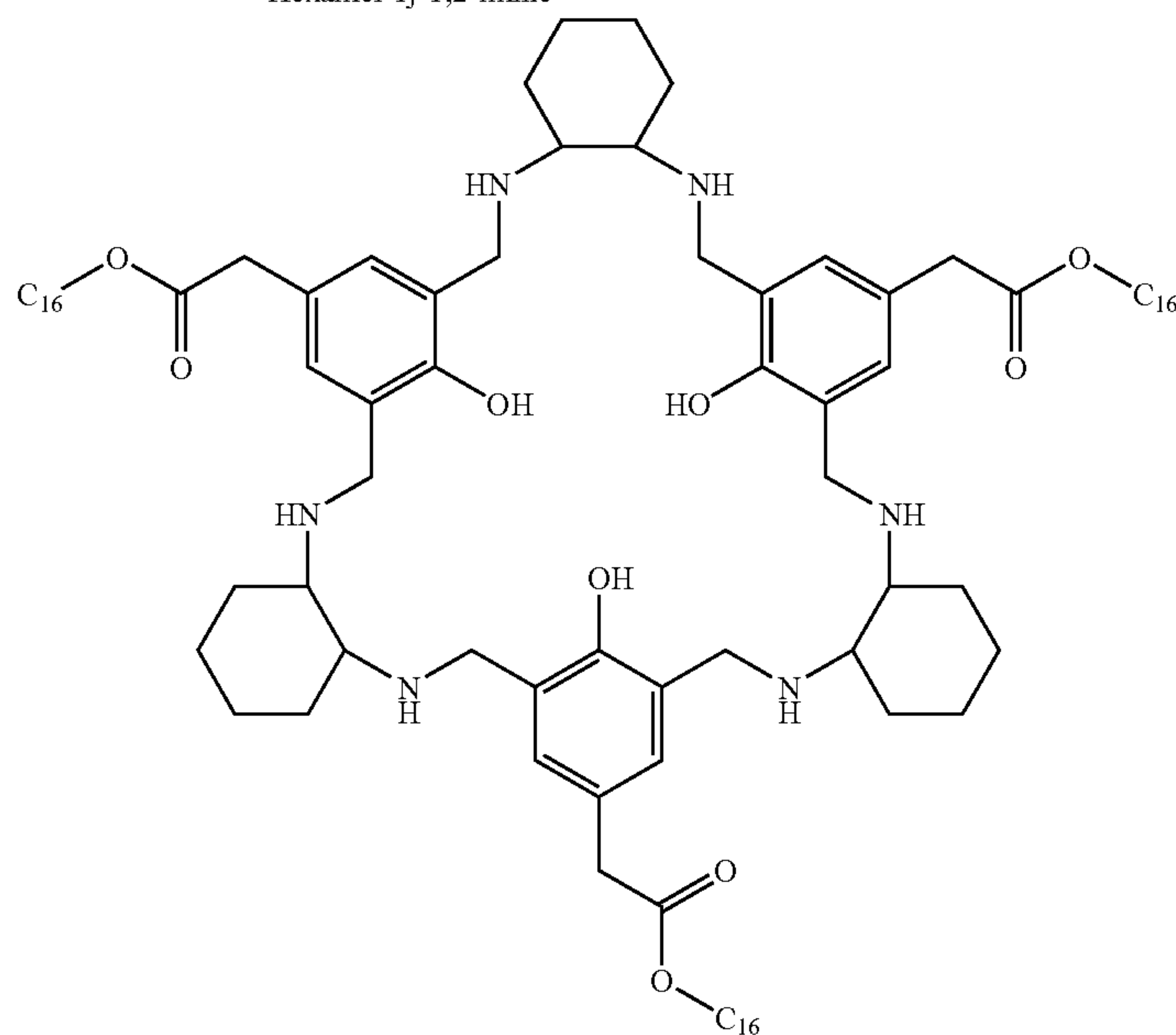
Hexamer 1jh-1,2-amine
