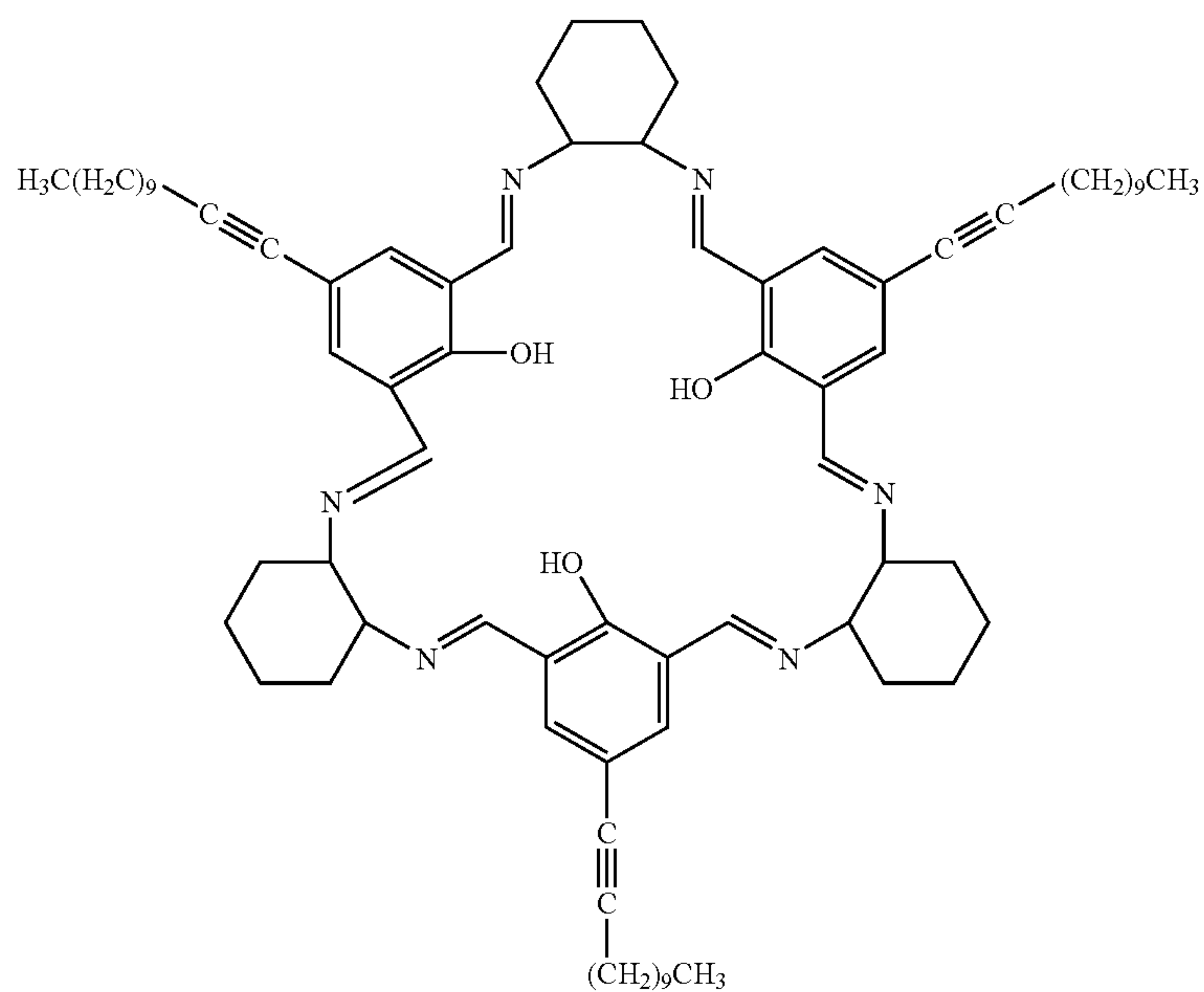
Hexamer 1a
