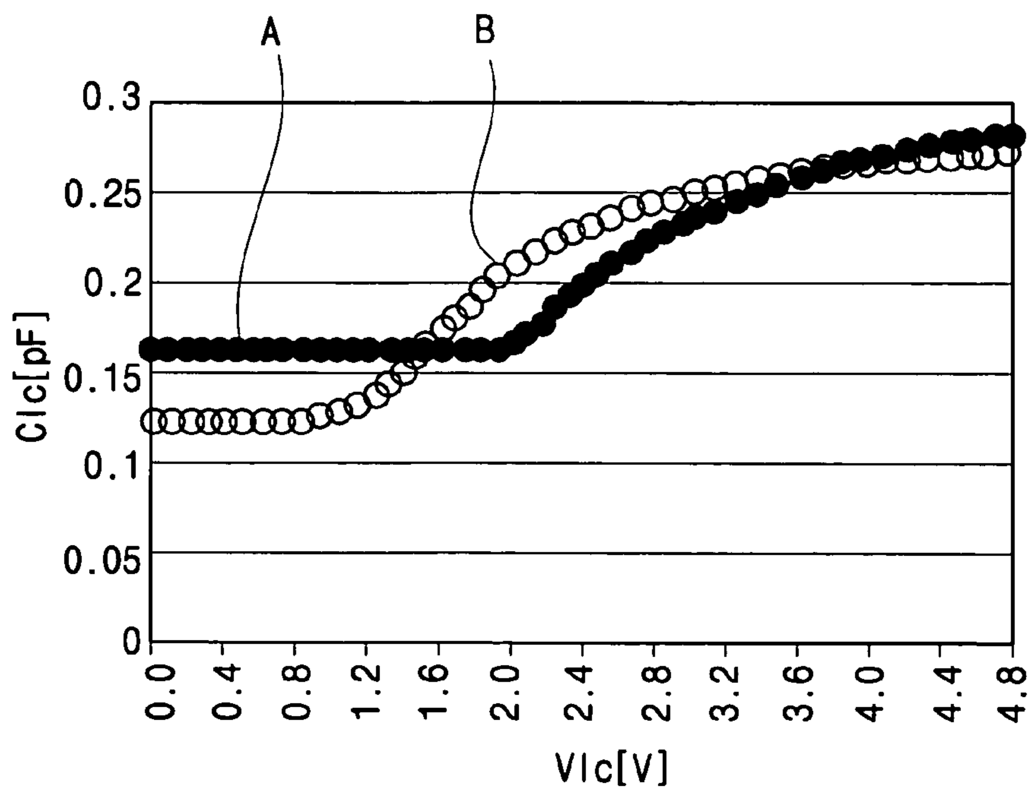
FIG. 3B
