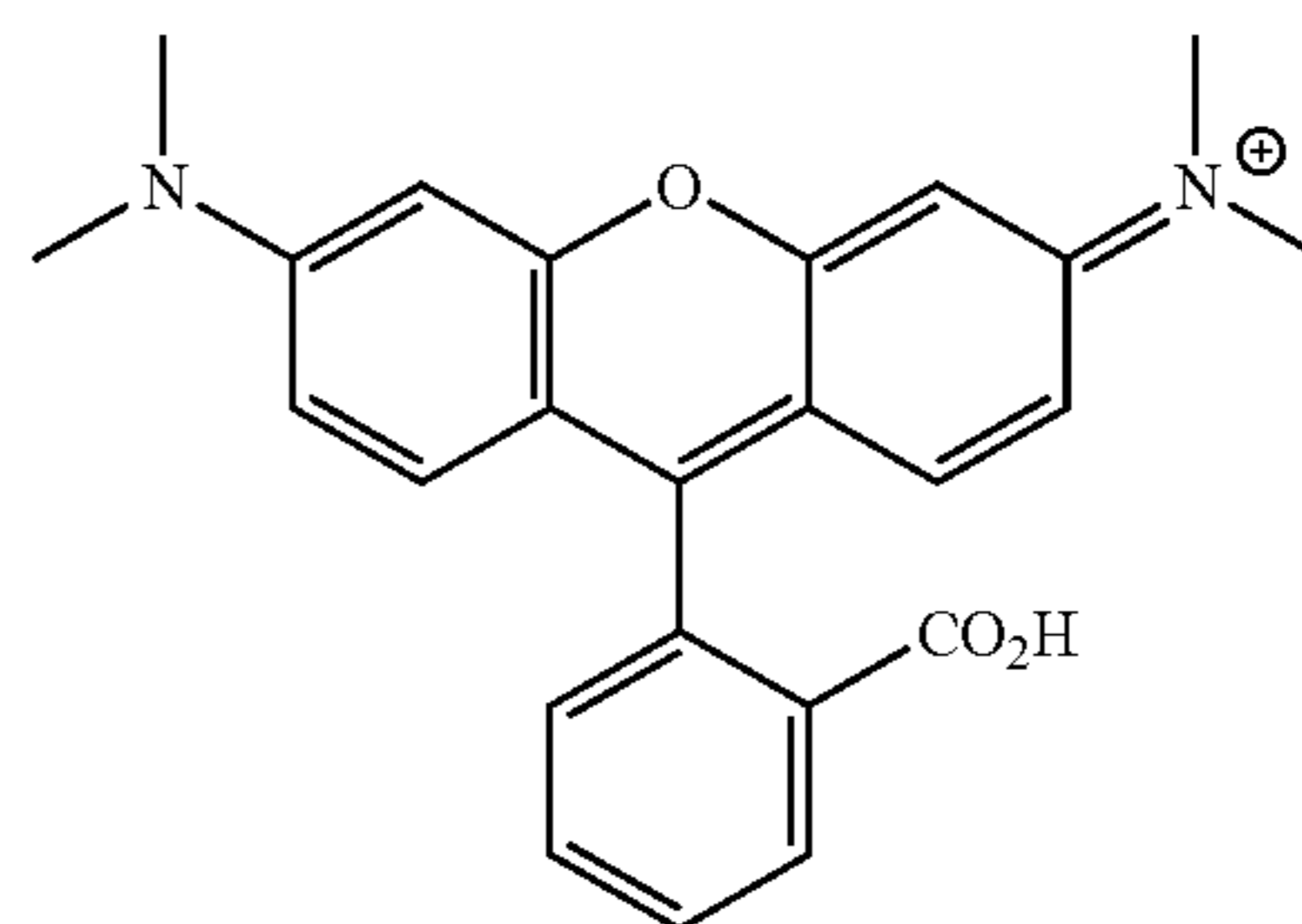
Rhodamine
