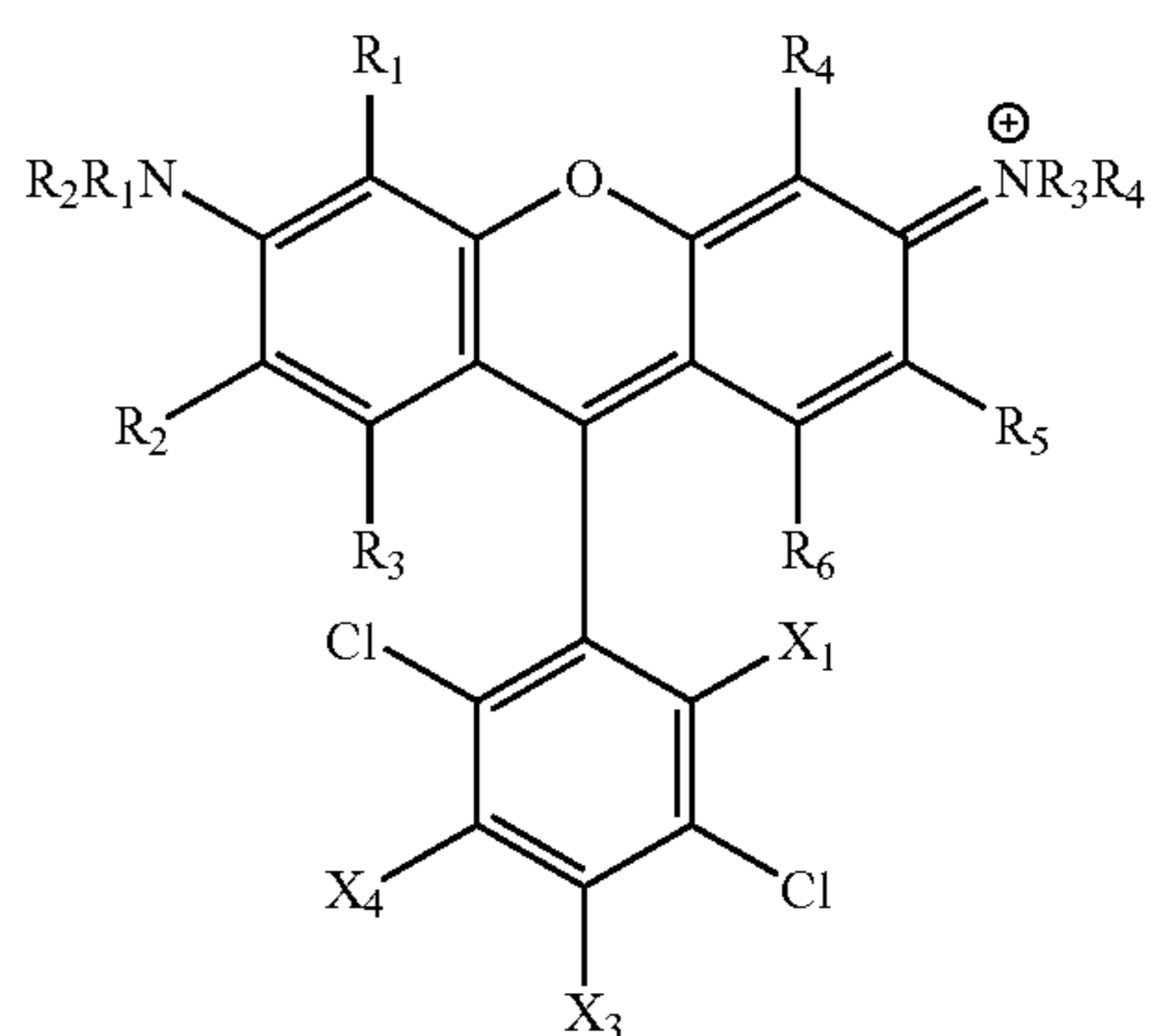
4,7-Dichlororhodamine
