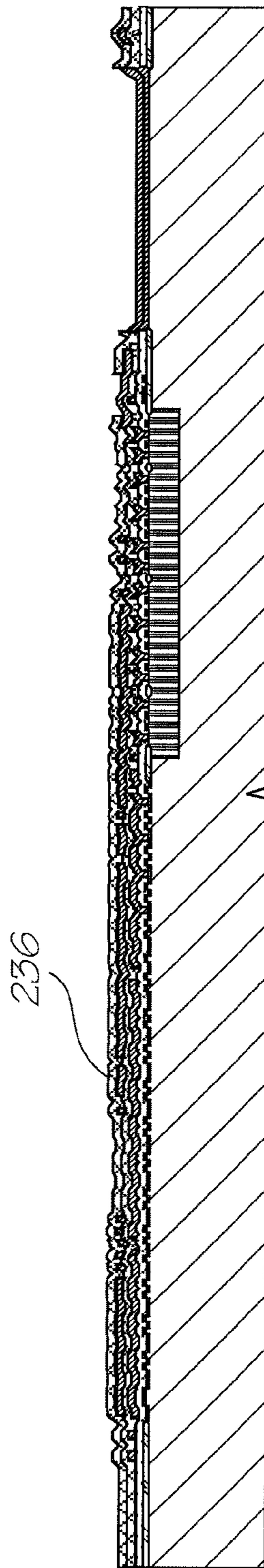
Deposit ILD 3, etch vias
