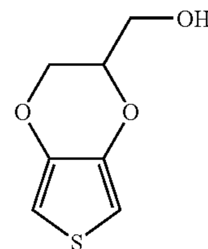
EDT-methanol
