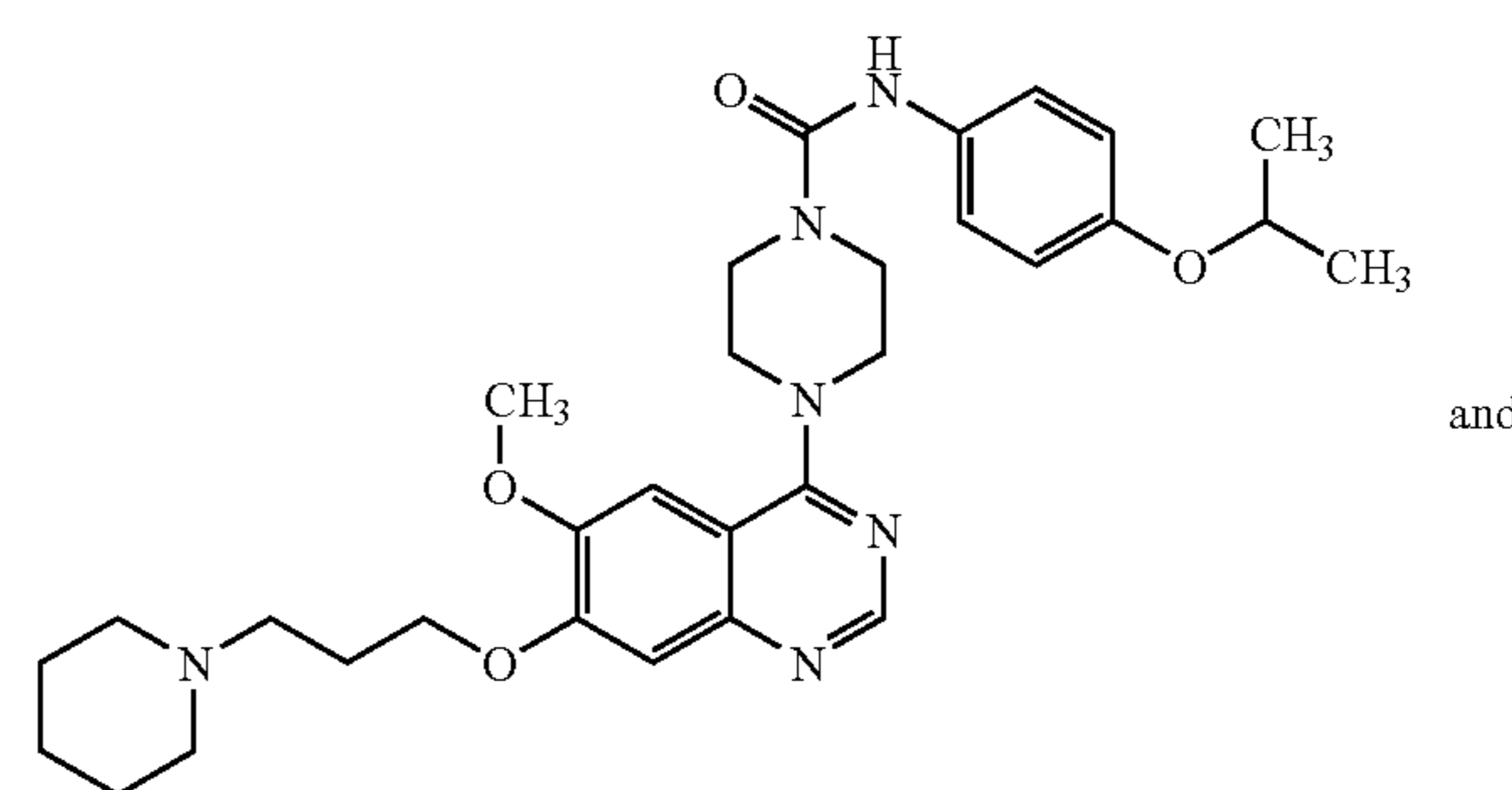
MLN518
